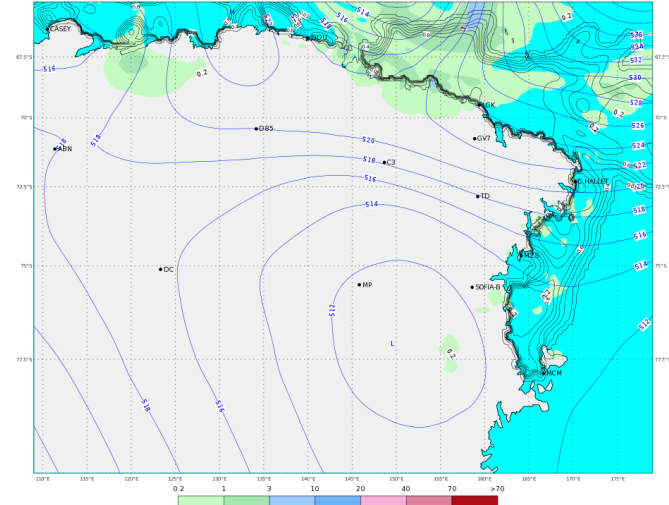
ECMWF 02 Gennaio 2018 00UTC Forecast T+24 VT: Mercoledì 03 Gennaio 2018 00UTC Terra Vittoria - Geopotential at 500 hPa + 6h accumulated precipitation (mm)
