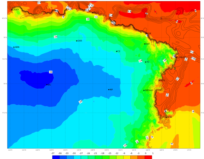
ECMWF 02 Gennaio 2018 00UTC Forecast T+18 VT: Martedì 02 Gennaio 2018 18UTC Terra Vittoria - Temperature at 2 m (°C)
