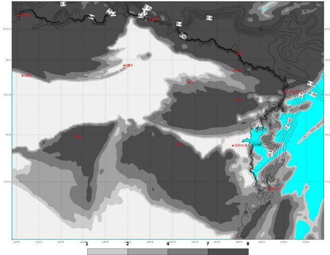
ECMWF 02 Gennaio 2018 00UTC Forecast T+18 VT: Martedì 02 Gennaio 2018 18UTC Terra Vittoria - Total cloud cover (oct)
