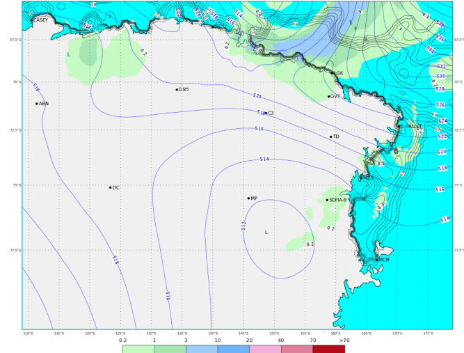
ECMWF 02 Gennaio 2018 00UTC Forecast T+30 VT: Mercoledì 03 Gennaio 2018 06UTC Terra Vittoria - Geopotential at 500 hPa + 6h accumulated precipitation (mm)
