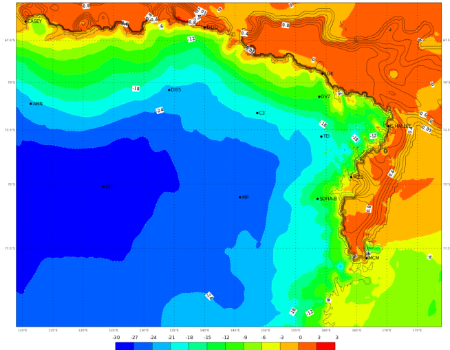
ECMWF 02 Gennaio 2018 00UTC Forecast T+30 VT: Mercoledì 03 Gennaio 2018 06UTC Terra Vittoria - Temperature at 2 m (°C)
