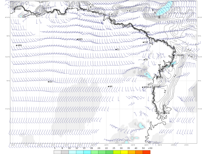
ECMWF 02 Gennaio 2018 00UTC Forecast T+36 VT: Mercoledì 03 Gennaio 2018 12UTC Terra Vittoria - Wind at 10 m (kts)
