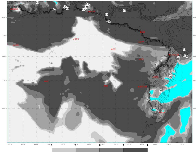
ECMWF 02 Gennaio 2018 00UTC Forecast T+24 VT: Mercoledì 03 Gennaio 2018 00UTC Terra Vittoria - Total cloud cover (oct)
