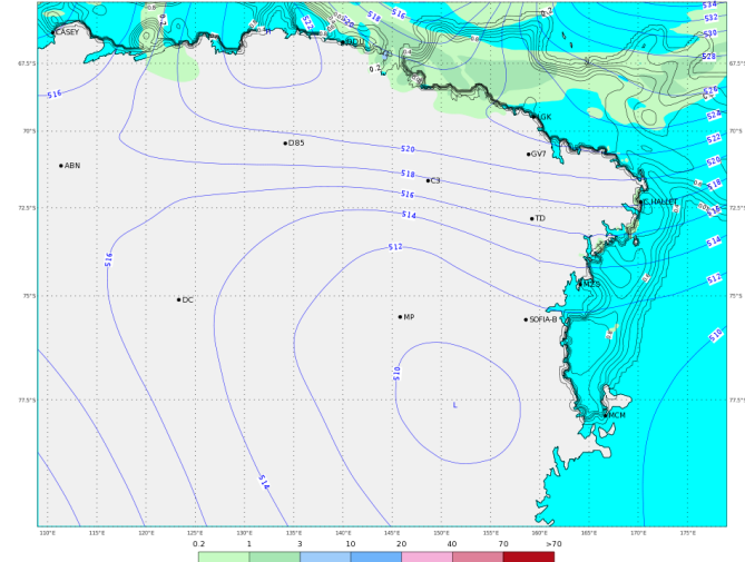
ECMWF 02 Gennaio 2018 00UTC Forecast T+18 VT: Martedì 02 Gennaio 2018 18UTC Terra Vittoria - Geopotential at 500 hPa + 6h accumulated precipitation (mm)
