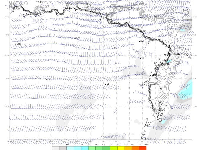
ECMWF 02 Gennaio 2018 00UTC Forecast T+30 VT: Mercoledì 03 Gennaio 2018 06UTC Terra Vittoria - Wind at 10 m (kts)
