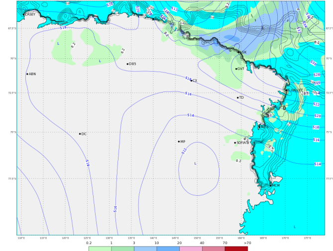
ECMWF 02 Gennaio 2018 00UTC Forecast T+36 VT: Mercoledì 03 Gennaio 2018 12UTC Terra Vittoria - Geopotential at 500 hPa + 6h accumulated precipitation (mm)
