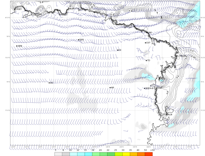
ECMWF 02 Gennaio 2018 00UTC Forecast T+24 VT: Mercoledì 03 Gennaio 2018 00UTC Terra Vittoria - Wind at 10 m (kts)
