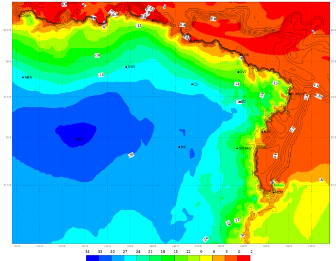
ECMWF 02 Gennaio 2018 00UTC Forecast T+36 VT: Mercoledì 03 Gennaio 2018 12UTC Terra Vittoria - Temperature at 2 m (°C)
