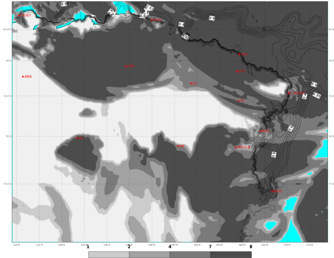
ECMWF 02 Gennaio 2018 00UTC Forecast T+36 VT: Mercoledì 03 Gennaio 2018 12UTC Terra Vittoria - Total cloud cover (oct)
