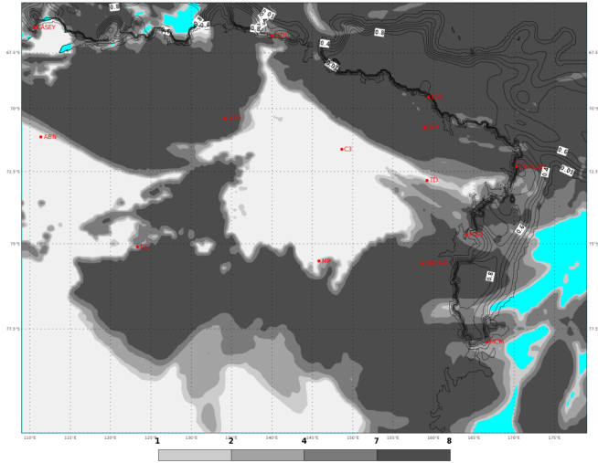
ECMWF 02 Gennaio 2018 00UTC Forecast T+30 VT: Mercoledì 03 Gennaio 2018 06UTC Terra Vittoria - Total cloud cover (oct)
