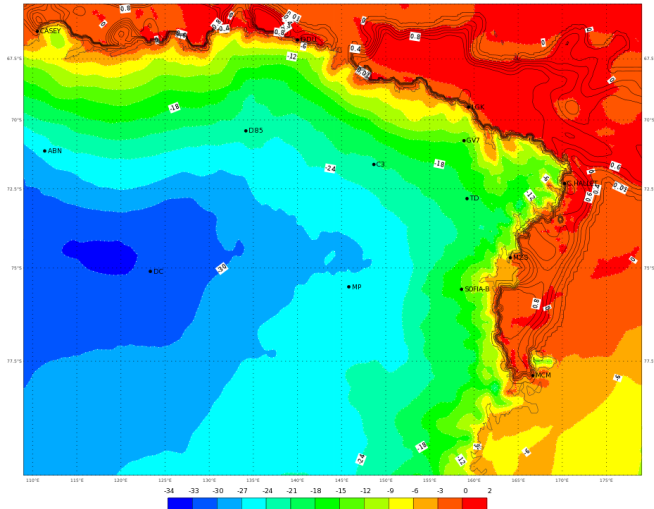
ECMWF 02 Gennaio 2018 00UTC Forecast T+24 VT: Mercoledì 03 Gennaio 2018 00UTC Terra Vittoria - Temperature at 2 m (°C)
