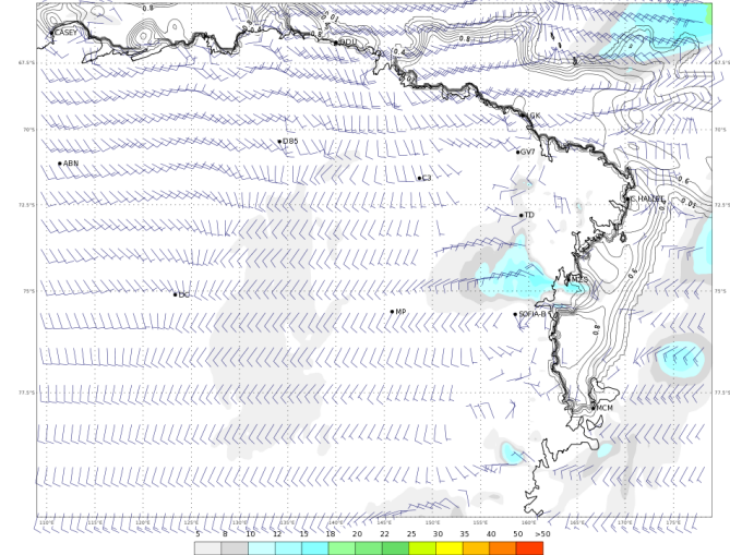
ECMWF 02 Gennaio 2018 00UTC Forecast T+18 VT: Martedì 02 Gennaio 2018 18UTC Terra Vittoria - Wind at 10 m (kts)
