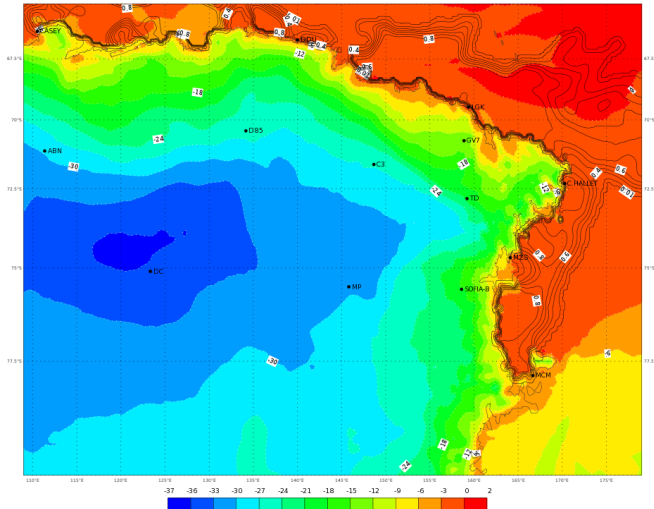
ECMWF 03 Gennaio 2018 00UTC Forecast T+18 VT: Mercoledì 03 Gennaio 2018 18UTC Terra Vittoria - temperature at 2 m (°C)
