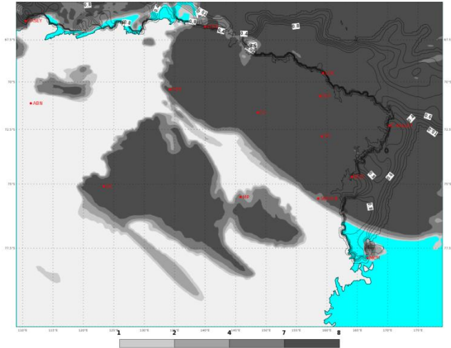
ECMWF 03 Gennaio 2018 00UTC Forecast T+36 VT: Giovedì 04 Gennaio 2018 12UTC Terra Vittoria - Total cloud cover (oct)
