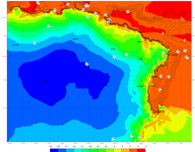
ECMWF 03 Gennaio 2018 00UTC Forecast T+36 VT: Giovedì 04 Gennaio 2018 12UTC Terra Vittoria - Temperature at 2 m (°C)
