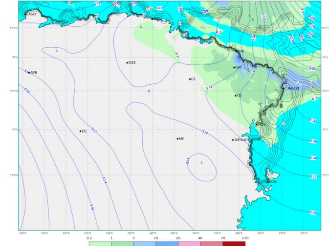
ECMWF 03 Gennaio 2018 00UTC Forecast T+36 VT: Giovedì 04 Gennaio 2018 12UTC Terra Vittoria - Geopotential at 500 hPa + 6h accumulated precipitation (mm)
