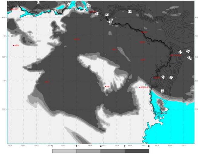
ECMWF 03 Gennaio 2018 00UTC Forecast T+30 VT: Giovedì 04 Gennaio 2018 06UTC Terra Vittoria - Total cloud cover (oct)
