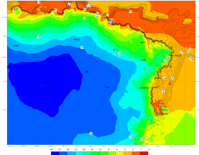
ECMWF 03 Gennaio 2018 00UTC Forecast T+30 VT: Giovedì 04 Gennaio 2018 06UTC Terra Vittoria - Temperature at 2 m (°C)
