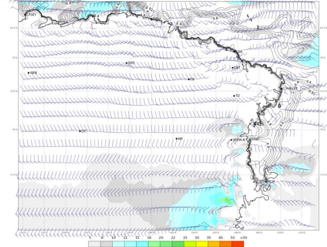
ECMWF 03 Gennaio 2018 00UTC Forecast T+36 VT: Giovedì 04 Gennaio 2018 12UTC Terra Vittoria - Wind at 10 m (kts)
