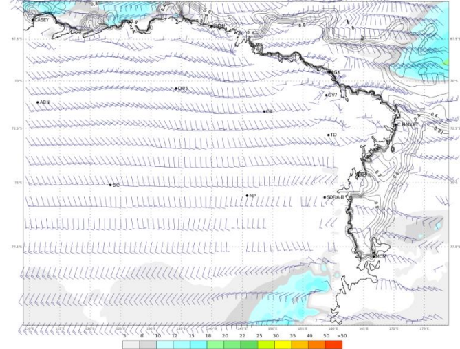
ECMWF 03 Gennaio 2018 00UTC Forecast T+30 VT: Giovedì 04 Gennaio 2018 06UTC Terra Vittoria - Wind at 10 m (kts)
