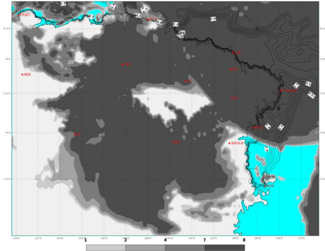
ECMWF 03 Gennaio 2018 00UTC Forecast T+24 VT: Giovedì 04 Gennaio 2018 00UTC Terra Vittoria - Total cloud cover (oct)
