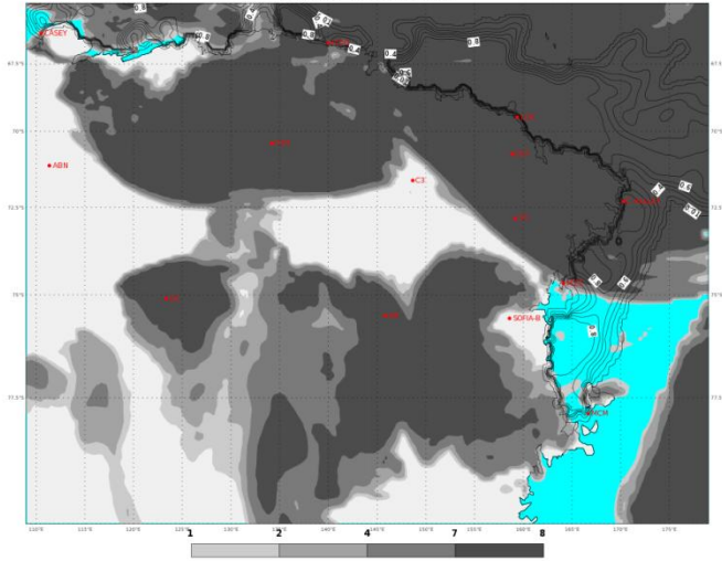
ECMWF 03 Gennaio 2018 00UTC Forecast T+18 VT: Mercoledì 03 Gennaio 2018 18UTC Terra Vittoria - Total cloud cover (oct)
