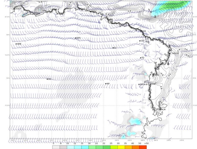
ECMWF 03 Gennaio 2018 00UTC Forecast T+18 VT: Mercoledì 03 Gennaio 2018 18UTC Terra Vittoria - Wind at 10 m (kts)
