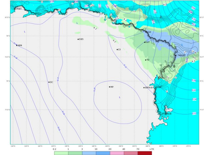
ECMWF 03 Gennaio 2018 00UTC Forecast T+30 VT: Giovedì 04 Gennaio 2018 06UTC Terra Vittoria - Geopotential at 500 hPa + 6h accumulated precipitation (mm)
