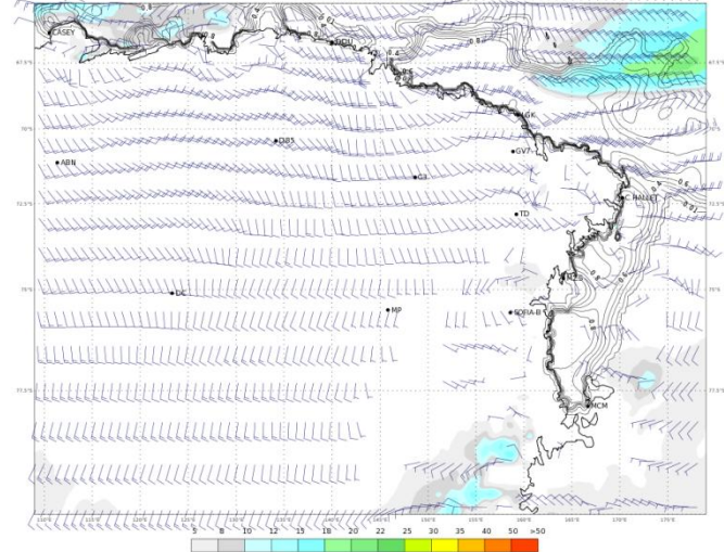
ECMWF 03 Gennaio 2018 00UTC Forecast T+24 VT: Giovedì 04 Gennaio 2018 00UTC Terra Vittoria - Wind at 10 m (kts)
