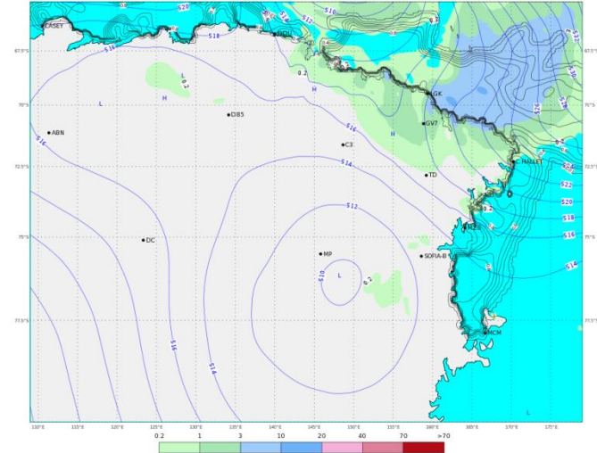
ECMWF 03 Gennaio 2018 00UTC Forecast T+18 VT: Mercoledì 03 Gennaio 2018 18UTC Terra Vittoria - Geopotential at 500 hPa + 6h accumulated precipitation (mm)
