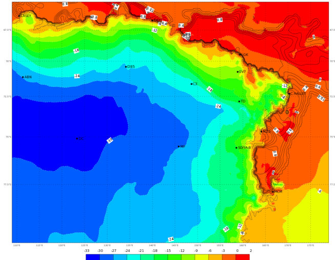
ECMWF 03 Gennaio 2018 00UTC Forecast T+24 VT: Giovedì 04 Gennaio 2018 00UTC Terra Vittoria - Temperature at 2 m (°C)
