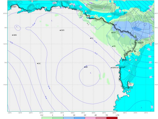
ECMWF 03 Gennaio 2018 00UTC Forecast T+24 VT: Giovedì 04 Gennaio 2018 00UTC Terra Vittoria - Geopotential at 500 hPa + 6h accumulated precipitation (mm)
