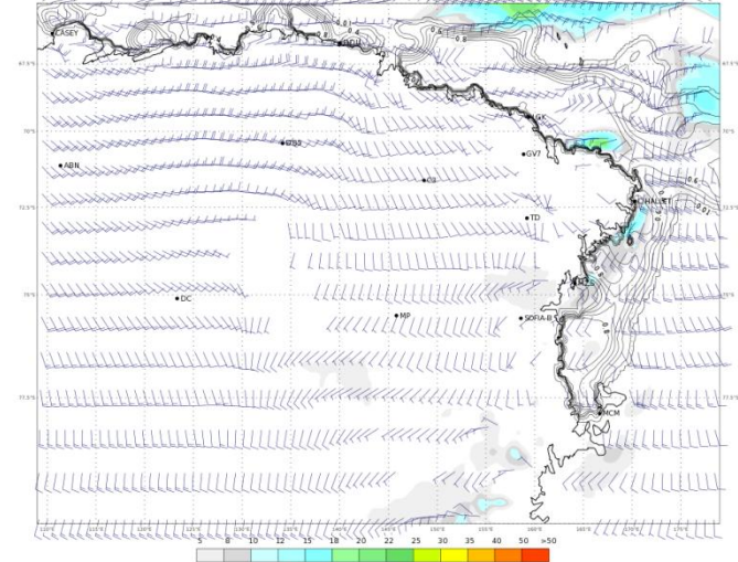
ECMWF 05 Gennaio 2018 00UTC Forecast T+24 VT: Sabato 06 Gennaio 2018 00UTC Terra Vittoria - Wind at 10 m (kts)
