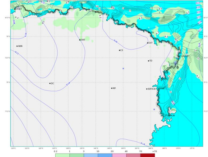
ECMWF 05 Gennaio 2018 00UTC Forecast T+30 VT: Sabato 06 Gennaio 2018 06UTC Terra Vittoria - Geopotential at 500 hPa + 6h accumulated precipitation (mm)
