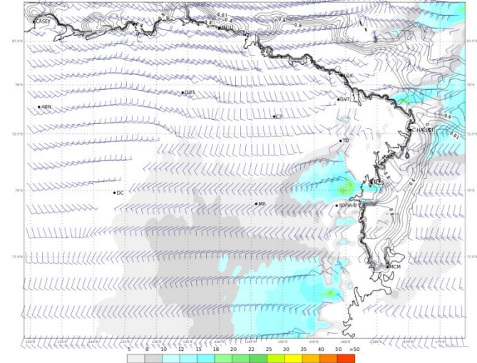
ECMWF 05 Gennaio 2018 00UTC Forecast T+42 VT: Sabato 06 Gennaio 2018 18UTC Terra Vittoria - Wind at 10 m (kts)
