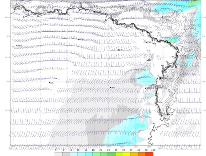
ECMWF 05 Gennaio 2018 00UTC Forecast T+36 VT: Sabato 06 Gennaio 2018 12UTC Terra Vittoria - Wind at 10 m (kts)
