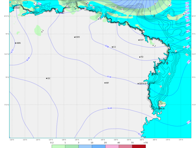
ECMWF 05 Gennaio 2018 00UTC Forecast T+48 VT: Domenica 07 Gennaio 2018 00UTC Terra Vittoria - Geopotential at 500 hPa + 6h accumulated precipitation (mm)
