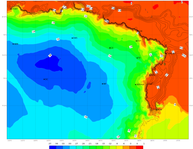
ECMWF 05 Gennaio 2018 00UTC Forecast T+18 VT: Venerdì 05 Gennaio 2018 18UTC Terra Vittoria - temperature at 2 m (°C)
