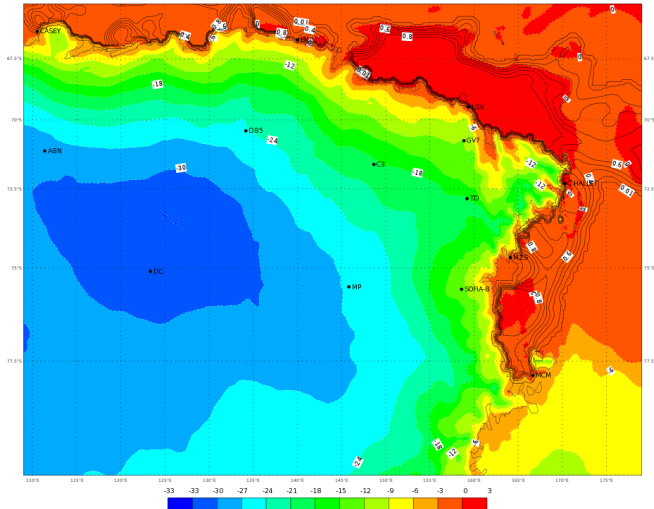
ECMWF 05 Gennaio 2018 00UTC Forecast T+24 VT: Sabato 06 Gennaio 2018 00UTC Terra Vittoria - Temperature at 2 m (°C)
