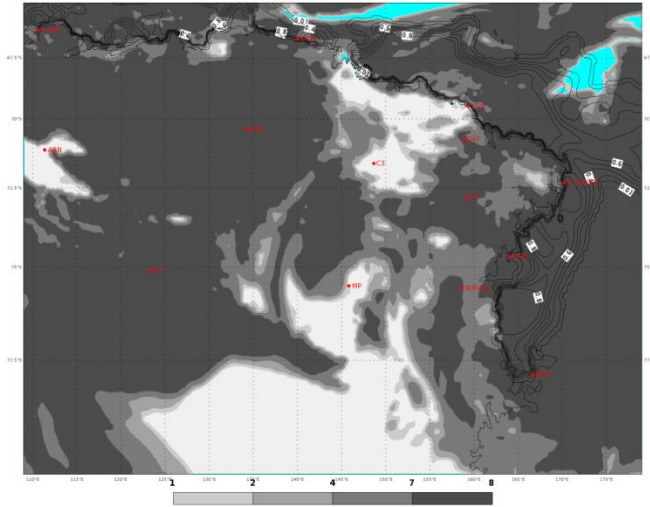
ECMWF 05 Gennaio 2018 00UTC Forecast T+30 VT: Sabato 06 Gennaio 2018 06UTC Terra Vittoria - Total cloud cover (oct)
