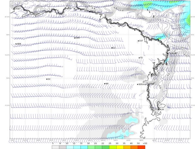
ECMWF 05 Gennaio 2018 00UTC Forecast T+30 VT: Sabato 06 Gennaio 2018 06UTC Terra Vittoria - Wind at 10 m (kts)
