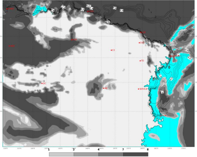
ECMWF 05 Gennaio 2018 00UTC Forecast T+48 VT: Domenica 07 Gennaio 2018 00UTC Terra Vittoria - Total cloud cover (oct)
