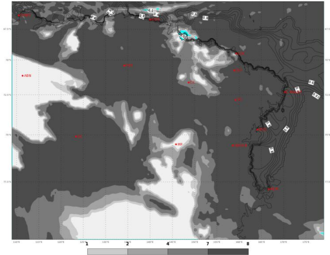
ECMWF 05 Gennaio 2018 00UTC Forecast T+24 VT: Sabato 06 Gennaio 2018 00UTC Terra Vittoria - Total cloud cover (oct)
