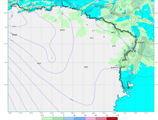
ECMWF 05 Gennaio 2018 00UTC Forecast T+18 VT: Venerdì 05 Gennaio 2018 18UTC Terra Vittoria - Geopotential at 500 hPa + 6h accumulated precipitation (mm)
