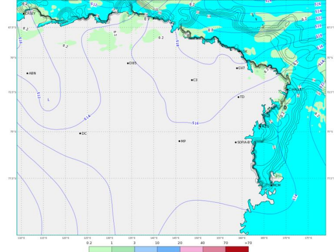
ECMWF 05 Gennaio 2018 00UTC Forecast T+36 VT: Sabato 06 Gennaio 2018 12UTC Terra Vittoria - Geopotential at 500 hPa + 6h accumulated precipitation (mm)
