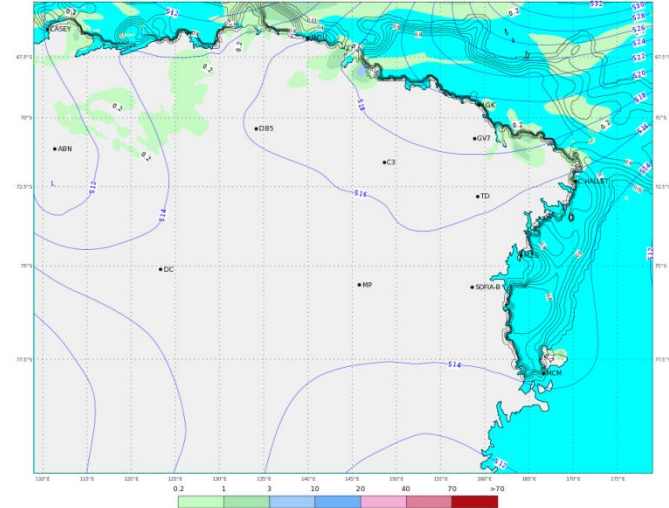
ECMWF 05 Gennaio 2018 00UTC Forecast T+42 VT: Sabato 06 Gennaio 2018 18UTC Terra Vittoria - Geopotential at 500 hPa + 6h accumulated precipitation (mm)
