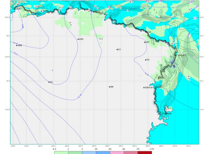
ECMWF 05 Gennaio 2018 00UTC Forecast T+24 VT: Sabato 06 Gennaio 2018 00UTC Terra Vittoria - Geopotential at 500 hPa + 6h accumulated precipitation (mm)
