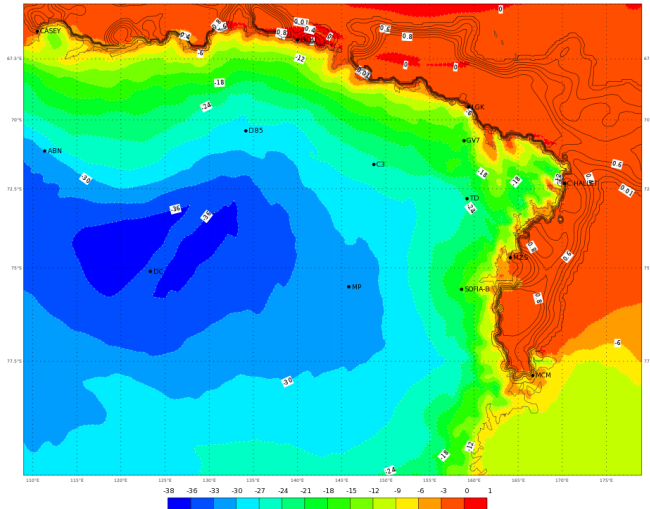
ECMWF 05 Gennaio 2018 00UTC Forecast T+42 VT: Sabato 06 Gennaio 2018 18UTC Terra Vittoria - Temperature at 2 m (°C)
