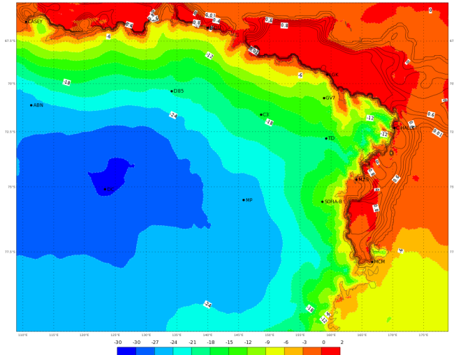
ECMWF 05 Gennaio 2018 00UTC Forecast T+30 VT: Sabato 06 Gennaio 2018 06UTC Terra Vittoria - Temperature at 2 m (°C)
