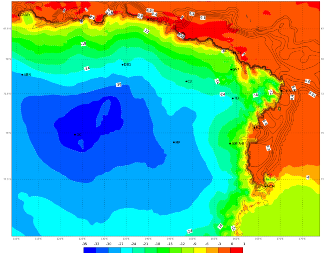
ECMWF 05 Gennaio 2018 00UTC Forecast T+36 VT: Sabato 06 Gennaio 2018 12UTC Terra Vittoria - Temperature at 2 m (°C)
