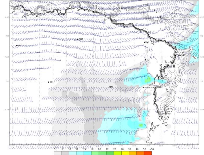
ECMWF 05 Gennaio 2018 00UTC Forecast T+48 VT: Domenica 07 Gennaio 2018 00UTC Terra Vittoria - Wind at 10 m (kts)
