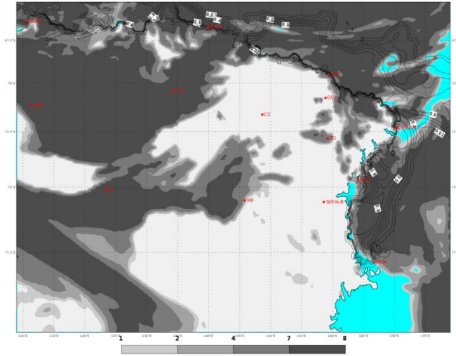
ECMWF 05 Gennaio 2018 00UTC Forecast T+42 VT: Sabato 06 Gennaio 2018 18UTC Terra Vittoria - Total cloud cover (oct)
