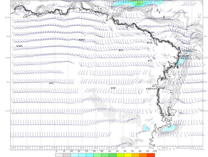
ECMWF 05 Gennaio 2018 00UTC Forecast T+18 VT: Venerdì 05 Gennaio 2018 18UTC Terra Vittoria - Wind at 10 m (kts)
