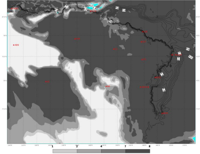
ECMWF 05 Gennaio 2018 00UTC Forecast T+18 VT: Venerdì 05 Gennaio 2018 18UTC Terra Vittoria - Total cloud cover (oct)
