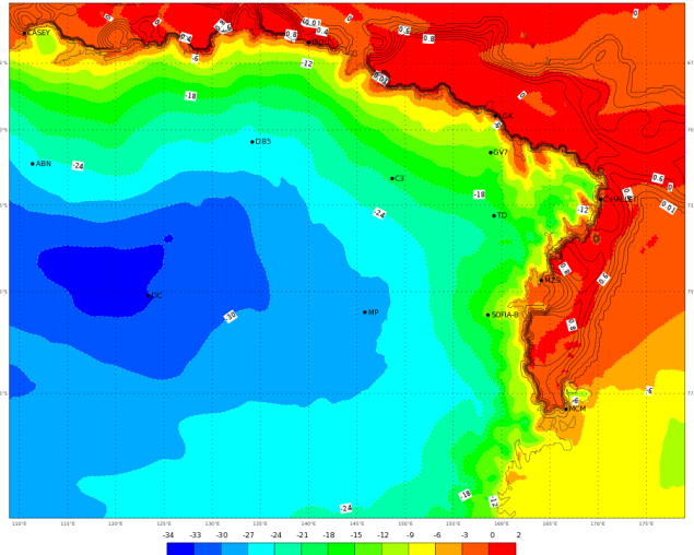
ECMWF 05 Gennaio 2018 00UTC Forecast T+48 VT: Domenica 07 Gennaio 2018 00UTC Terra Vittoria - Temperature at 2 m (°C)
