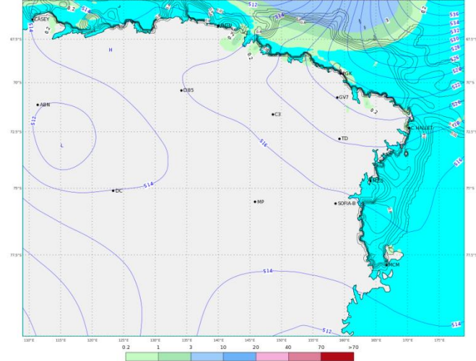
ECMWF 06 Gennaio 2018 00UTC Forecast T+24 VT: Domenica 07 Gennaio 2018 00UTC Terra Vittoria - Geopotential at 500 hPa + 6h accumulated precipitation (mm)
