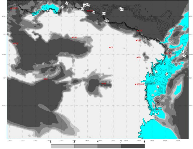
ECMWF 06 Gennaio 2018 00UTC Forecast T+24 VT: Domenica 07 Gennaio 2018 00UTC Terra Vittoria - Total cloud cover (oct)
