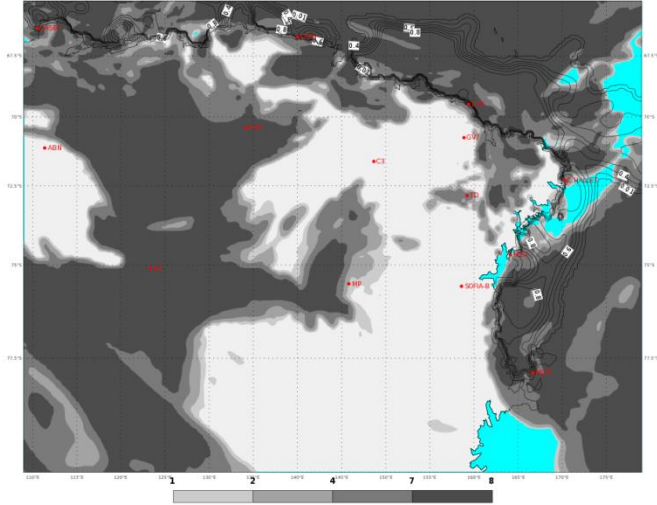
ECMWF 06 Gennaio 2018 00UTC Forecast T+18 VT: Sabato 06 Gennaio 2018 18UTC Terra Vittoria - Total cloud cover (oct)
