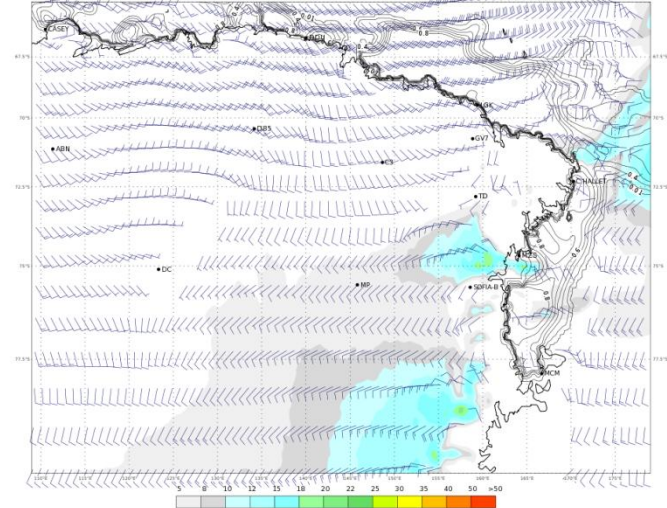
ECMWF 06 Gennaio 2018 00UTC Forecast T+24 VT: Domenica 07 Gennaio 2018 00UTC Terra Vittoria - Wind at 10 m (kts)
