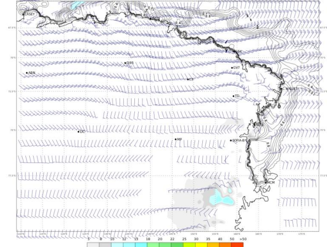
ECMWF 06 Gennaio 2018 00UTC Forecast T+48 VT: Lunedì 08 Gennaio 2018 00UTC Terra Vittoria - Wind at 10 m (kts)
