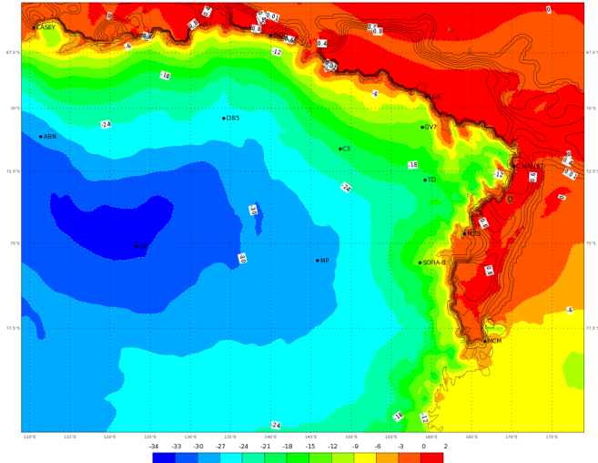
ECMWF 06 Gennaio 2018 00UTC Forecast T+24 VT: Domenica 07 Gennaio 2018 00UTC Terra Vittoria - temperature at 2 m (°C)
