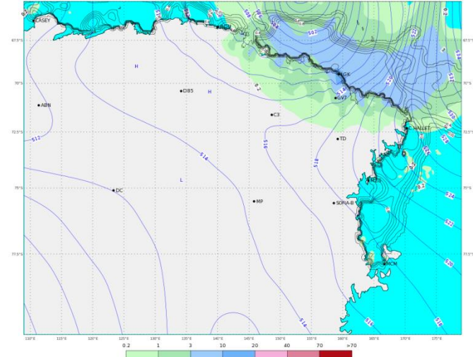
ECMWF 06 Gennaio 2018 00UTC Forecast T+42 VT: Domenica 07 Gennaio 18UTC Terra Vittoria - Geopotential at 500 hPa + 6h accumulated precipitation (mm)
