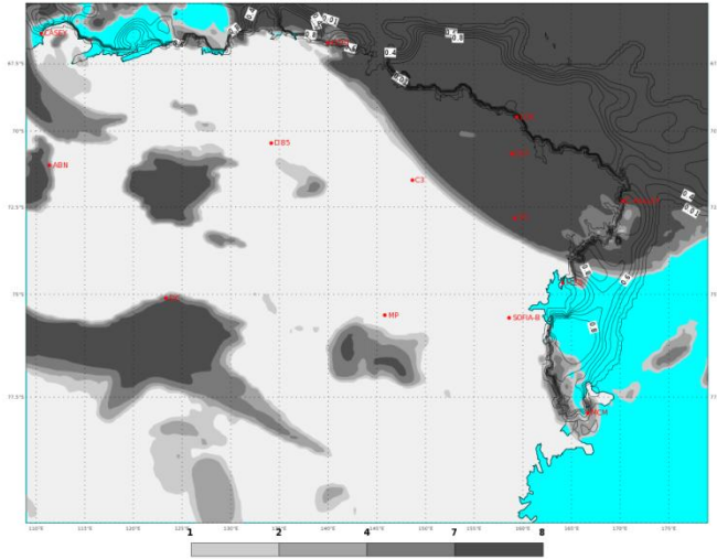
ECMWF 06 Gennaio 2018 00UTC Forecast T+36 VT: Domenica 07 Gennaio 2018 12UTC Terra Vittoria - Total cloud cover (oct)
