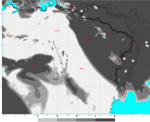
ECMWF 06 Gennaio 2018 00UTC Forecast T+48 VT: Lunedì 08 Gennaio 2018 00UTC Terra Vittoria - Total cloud cover (oct)
