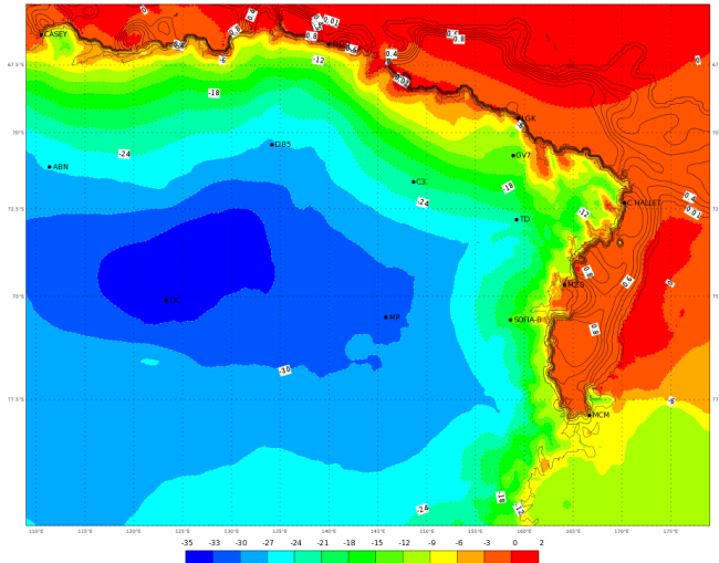
ECMWF 06 Gennaio 2018 00UTC Forecast T+36 VT: Domenica 07 Gennaio 2018 12UTC Terra Vittoria - Temperature at 2 m (°C)
