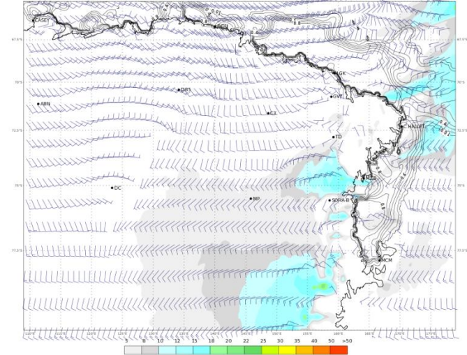
ECMWF 06 Gennaio 2018 00UTC Forecast T+18 VT: Sabato 06 Gennaio 2018 18UTC Terra Vittoria - Wind at 10 m (kts)
