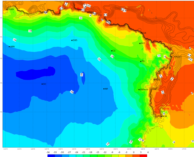
ECMWF 06 Gennaio 2018 00UTC Forecast T+48 VT: Lunedì 08 Gennaio 2018 00UTC Terra Vittoria - temperature at 2 m (°C)
