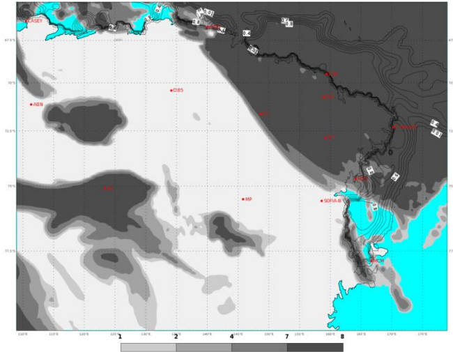
ECMWF 06 Gennaio 2018 00UTC Forecast T+42 VT: Domenica 07 Gennaio 18UTC Terra Vittoria - Total cloud cover (oct)
