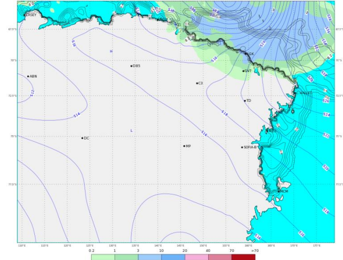
ECMWF 06 Gennaio 2018 00UTC Forecast T+36 VT: Domenica 07 Gennaio 2018 12UTC Terra Vittoria - Geopotential at 500 hPa + 6h accumulated precipitation (mm)
