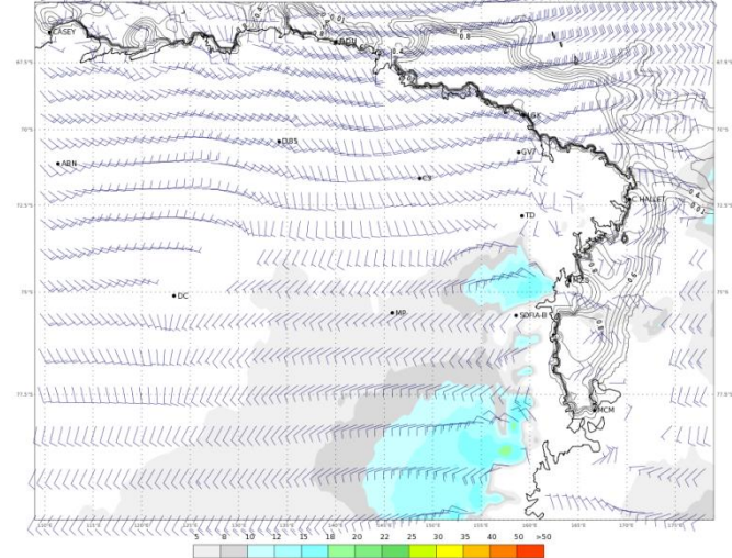
ECMWF 06 Gennaio 2018 00UTC Forecast T+30 VT: Domenica 07 Gennaio 2018 06UTC Terra Vittoria - Wind at 10 m (kts)
