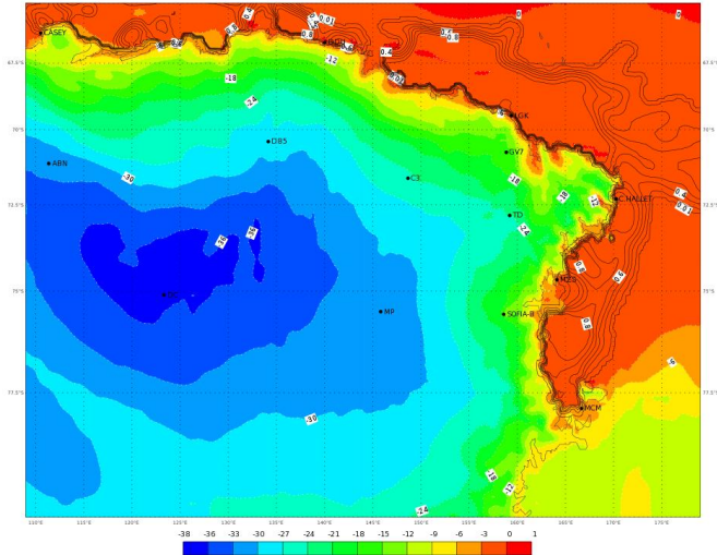
ECMWF 06 Gennaio 2018 00UTC Forecast T+18 VT: Sabato 06 Gennaio 2018 18UTC Terra Vittoria - temperature at 2 m (°C)
