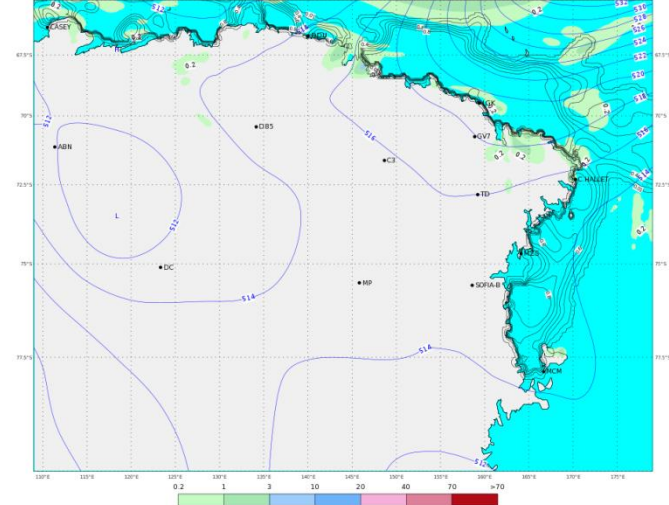
ECMWF 06 Gennaio 2018 00UTC Forecast T+18 VT: Sabato 06 Gennaio 2018 18UTC Terra Vittoria - Geopotential at 500 hPa + 6h accumulated precipitation (mm)
