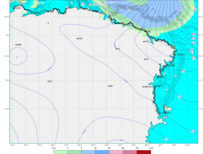
ECMWF 06 Gennaio 2018 00UTC Forecast T+30 VT: Domenica 07 Gennaio 2018 06UTC Terra Vittoria - Geopotential at 500 hPa + 6h accumulated precipitation (mm)
