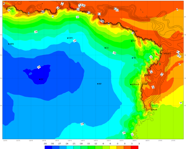
ECMWF 06 Gennaio 2018 00UTC Forecast T+30 VT: Domenica 07 Gennaio 2018 06UTC Terra Vittoria - temperature at 2 m (°C)
