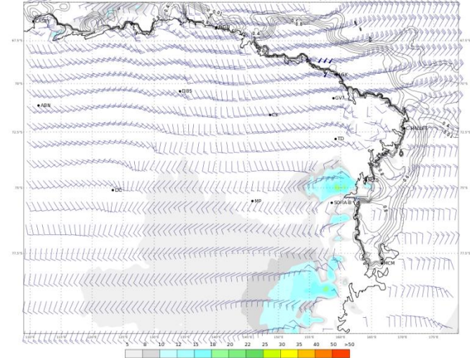
ECMWF 06 Gennaio 2018 00UTC Forecast T+42 VT: Domenica 07 Gennaio 18UTC Terra Vittoria - Wind at 10 m (kts)
