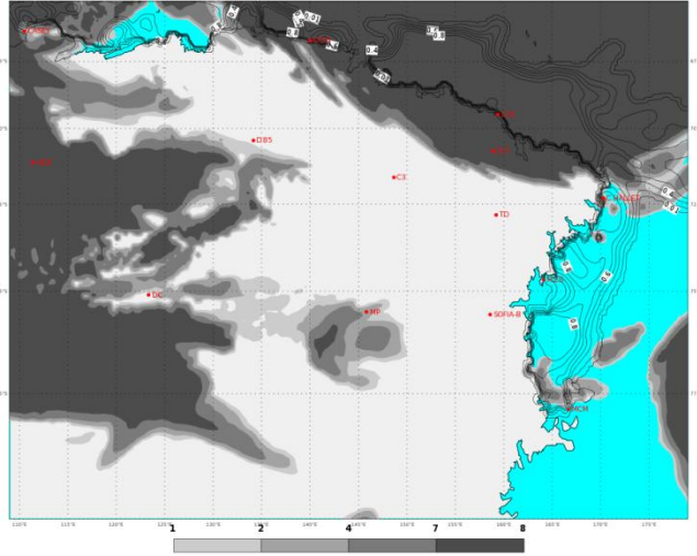
ECMWF 06 Gennaio 2018 00UTC Forecast T+30 VT: Domenica 07 Gennaio 2018 06UTC Terra Vittoria - Total cloud cover (oct)
