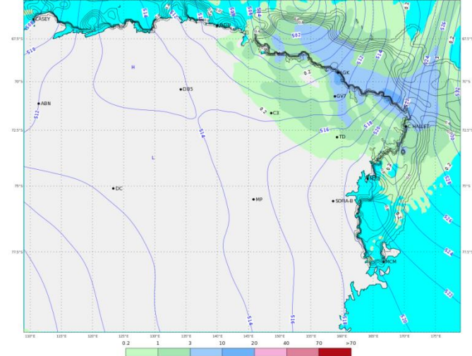
ECMWF 06 Gennaio 2018 00UTC Forecast T+48 VT: Lunedì 08 Gennaio 2018 00UTC Terra Vittoria - Geopotential at 500 hPa + 6h accumulated precipitation (mm)
