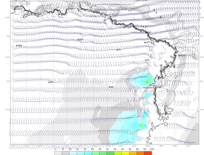
ECMWF 06 Gennaio 2018 00UTC Forecast T+36 VT: Domenica 07 Gennaio 2018 12UTC Terra Vittoria - Wind at 10 m (kts)
