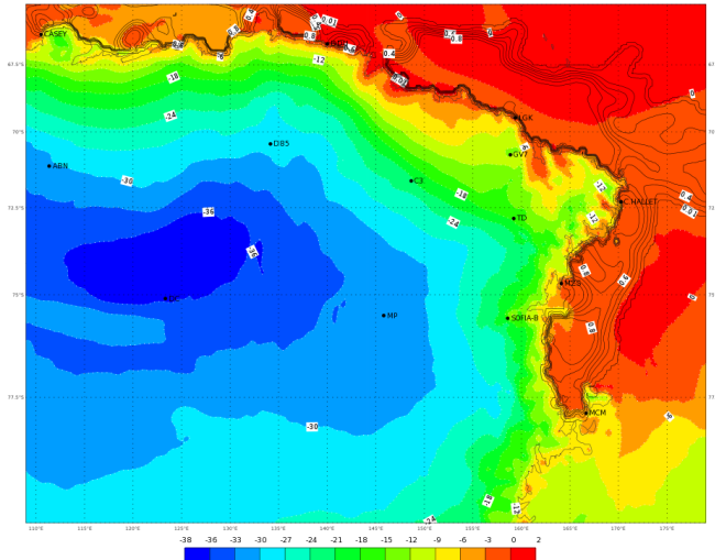
ECMWF 06 Gennaio 2018 00UTC Forecast T+42 VT: Domenica 07 Gennaio 18UTC Terra Vittoria - Temperature at 2 m (°C)
