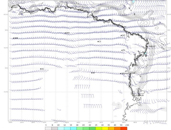
ECMWF 07 Gennaio 2018 00UTC Forecast T+48 VT: Martedì 09 Gennaio 2018 00UTC Terra Vittoria - Wind at 10 m (kts)
