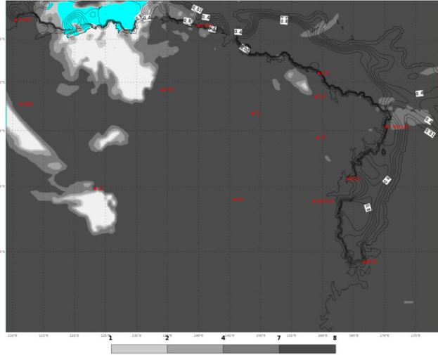
ECMWF 07 Gennaio 2018 00UTC Forecast T+48 VT: Martedì 09 Gennaio 2018 00UTC Terra Vittoria - Total cloud cover (oct)
