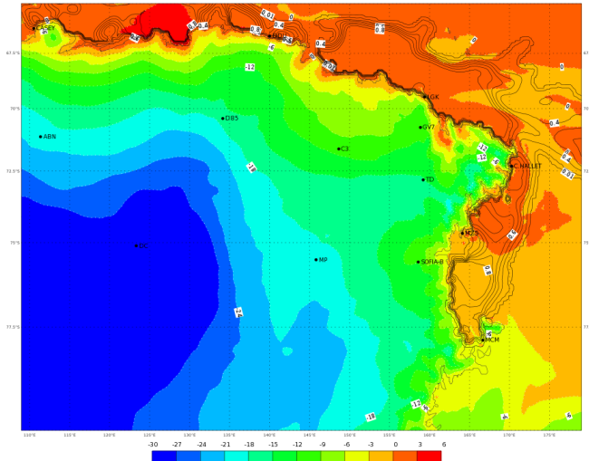
ECMWF 07 Gennaio 2018 00UTC Forecast T+54 VT: Martedì 09 Gennaio 2018 06UTC Terra Vittoria - Temperature at 2 m (°C)
