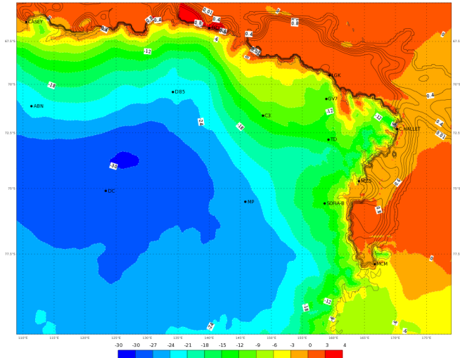
ECMWF 07 Gennaio 2018 00UTC Forecast T+30 VT: Lunedì 08 Gennaio 2018 06UTC Terra Vittoria - temperature at 2 m (°C)
