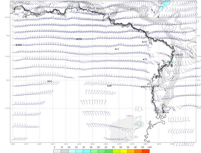
ECMWF 07 Gennaio 2018 00UTC Forecast T+54 VT: Martedì 09 Gennaio 2018 06UTC Terra Vittoria - Wind at 10 m (kts)
