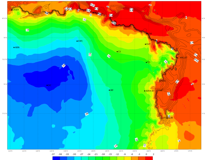
ECMWF 07 Gennaio 2018 00UTC Forecast T+42 VT: Lunedì 08 Gennaio 2018 18UTC Terra Vittoria - Temperature at 2 m (°C)
