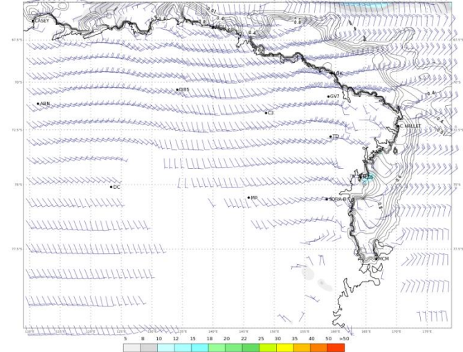
ECMWF 07 Gennaio 2018 00UTC Forecast T+30 VT: Lunedì 08 Gennaio 2018 06UTC Terra Vittoria - Wind at 10 m (kts)
