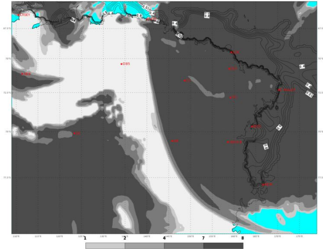
ECMWF 07 Gennaio 2018 00UTC Forecast T+30 VT: Lunedì 08 Gennaio 2018 06UTC Terra Vittoria - Total cloud cover (oct)
