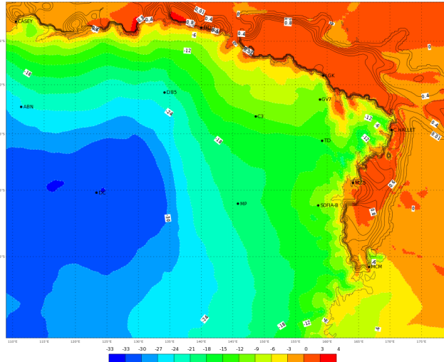
ECMWF 07 Gennaio 2018 00UTC Forecast T+48 VT: Martedì 09 Gennaio 2018 00UTC Terra Vittoria - Temperature at 2 m (°C)
