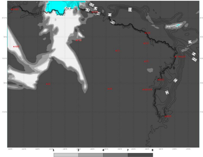
ECMWF 07 Gennaio 2018 00UTC Forecast T+42 VT: Lunedì 08 Gennaio 2018 18UTC Terra Vittoria - Total cloud cover (oct)
