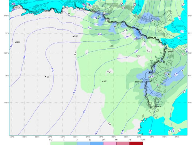
ECMWF 07 Gennaio 2018 00UTC Forecast T+48 VT: Martedì 09 Gennaio 2018 00UTC Terra Vittoria - Geopotential at 500 hPa + 6h accumulated precipitation (mm)
