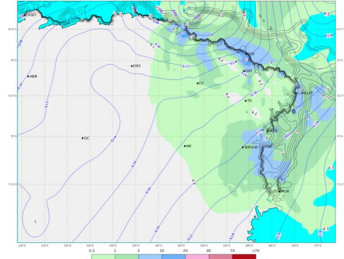
ECMWF 07 Gennaio 2018 00UTC Forecast T+42 VT: Lunedì 08 Gennaio 2018 18UTC Terra Vittoria - Geopotential at 500 hPa + 6h accumulated precipitation (mm)
