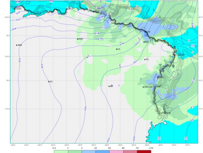
ECMWF 07 Gennaio 2018 00UTC Forecast T+54 VT: Martedì 09 Gennaio 2018 06UTC Terra Vittoria - Geopotential at 500 hPa + 6h accumulated precipitation (mm)
