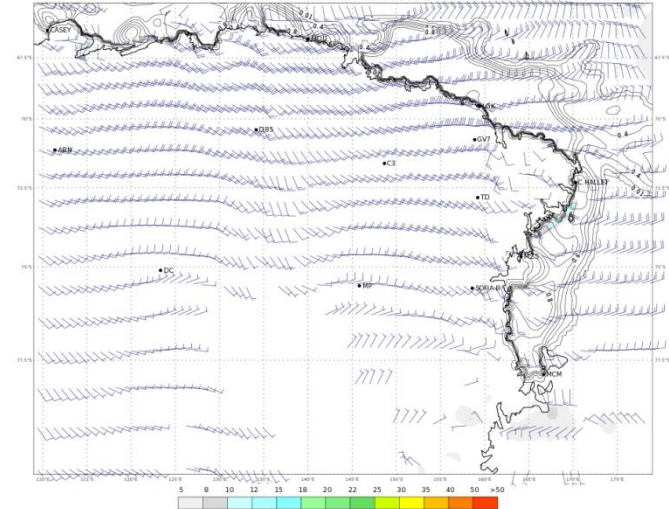
ECMWF 07 Gennaio 2018 00UTC Forecast T+42 VT: Lunedì 08 Gennaio 2018 18UTC Terra Vittoria - Wind at 10 m (kts)
