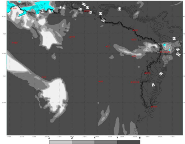
ECMWF 07 Gennaio 2018 00UTC Forecast T+54 VT: Martedì 09 Gennaio 2018 06UTC Terra Vittoria - Total cloud cover (oct)
