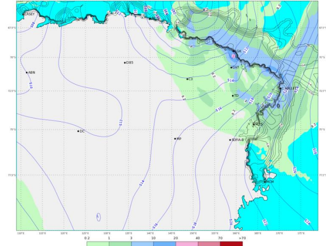
ECMWF 07 Gennaio 2018 00UTC Forecast T+30 VT: Lunedì 08 Gennaio 2018 06UTC Terra Vittoria - Geopotential at 500 hPa + 6h accumulated precipitation (mm)
