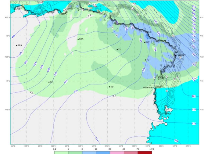
ECMWF 12 Gennaio 2018 00UTC Forecast T+48 VT: Domenica 14 Gennaio 2018 00UTC Terra Vittoria - Geopotential at 500 hPa + 6h accumulated precipitation (mm)
