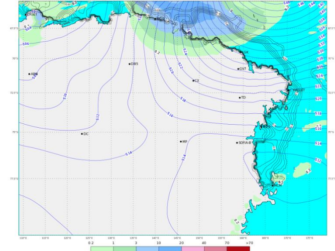
ECMWF 12 Gennaio 2018 00UTC Forecast T+24 VT: Sabato 13 Gennaio 2018 00UTC Terra Vittoria - Geopotential at 500 hPa + 6h accumulated precipitation (mm)
