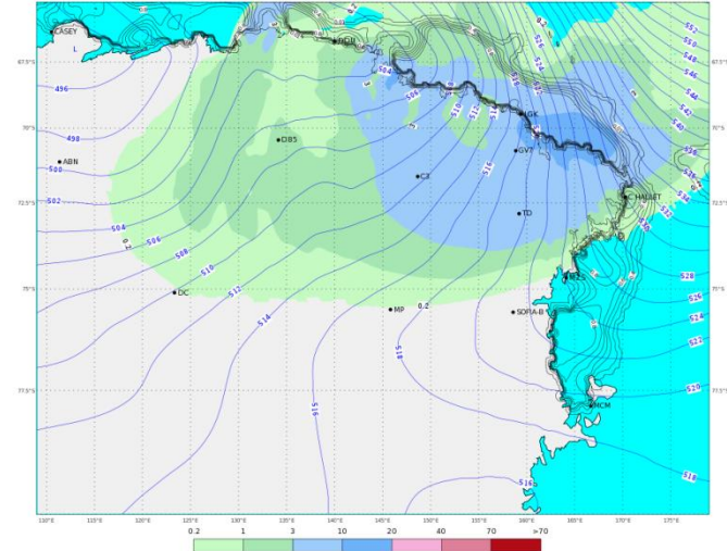
ECMWF 12 Gennaio 2018 00UTC Forecast T+42 VT: Sabato 13 Gennaio 2018 18UTC Terra Vittoria - Geopotential at 500 hPa + 6h accumulated precipitation (mm)
