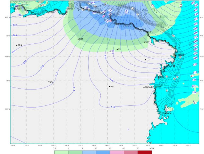
ECMWF 12 Gennaio 2018 00UTC Forecast T+30 VT: Sabato 13 Gennaio 2018 06UTC Terra Vittoria - Geopotential at 500 hPa + 6h accumulated precipitation (mm)
