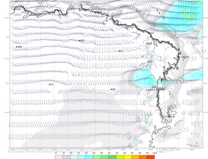
ECMWF 12 Gennaio 2018 00UTC Forecast T+18 VT: Venerdì 12 Gennaio 2018 18UTC Terra Vittoria - Wind at 10 m (kts)
