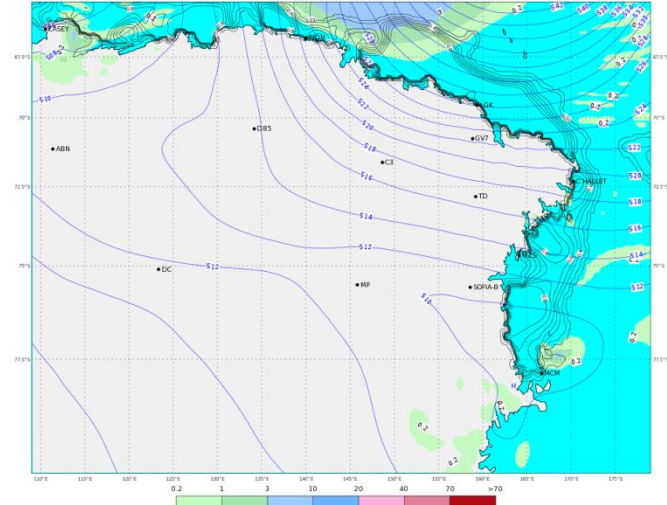
ECMWF 12 Gennaio 2018 00UTC Forecast T+18 VT: Venerdì 12 Gennaio 2018 18UTC Terra Vittoria - Geopotential at 500 hPa + 6h accumulated precipitation (mm)
