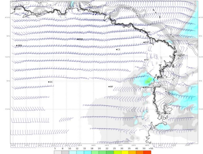
ECMWF 12 Gennaio 2018 00UTC Forecast T+30 VT: Sabato 13 Gennaio 2018 06UTC Terra Vittoria - Wind at 10 m (kts)
