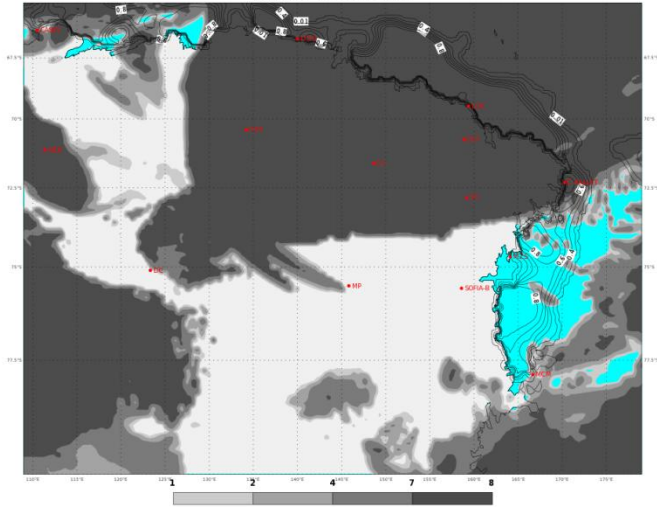
ECMWF 12 Gennaio 2018 00UTC Forecast T+30 VT: Sabato 13 Gennaio 2018 06UTC Terra Vittoria - Total cloud cover (oct)
