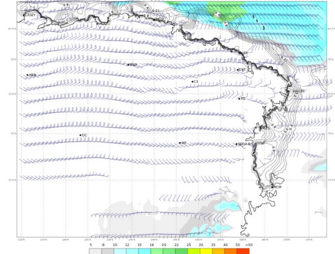
ECMWF 12 Gennaio 2018 00UTC Forecast T+48 VT: Domenica 14 Gennaio 2018 00UTC Terra Vittoria - Wind at 10 m (kts)
