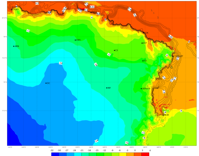
ECMWF 12 Gennaio 2018 00UTC Forecast T+54 VT: Domenica 14 Gennaio 2018 06UTC Terra Vittoria - Temperature at 2 m (°C)
