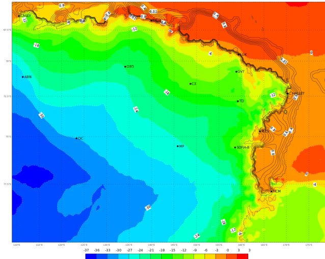
ECMWF 12 Gennaio 2018 00UTC Forecast T+42 VT: Sabato 13 Gennaio 2018 18UTC Terra Vittoria - temperature at 2 m (°C)
