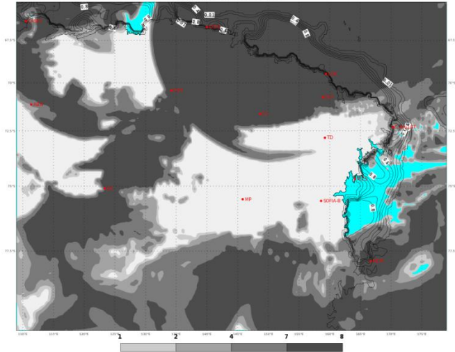
ECMWF 12 Gennaio 2018 00UTC Forecast T+24 VT: Sabato 13 Gennaio 2018 00UTC Terra Vittoria - Total cloud cover (oct)
