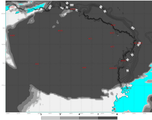
ECMWF 12 Gennaio 2018 00UTC Forecast T+42 VT: Sabato 13 Gennaio 2018 18UTC Terra Vittoria - Total cloud cover (oct)
