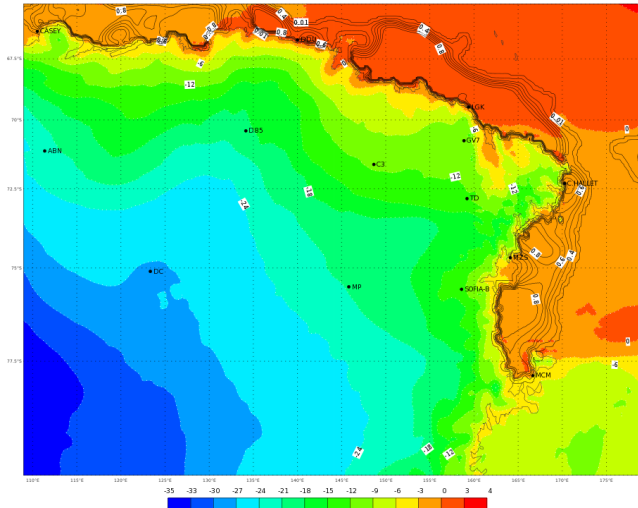
ECMWF 12 Gennaio 2018 00UTC Forecast T+48 VT: Domenica 14 Gennaio 2018 00UTC Terra Vittoria - Temperature at 2 m (°C)
