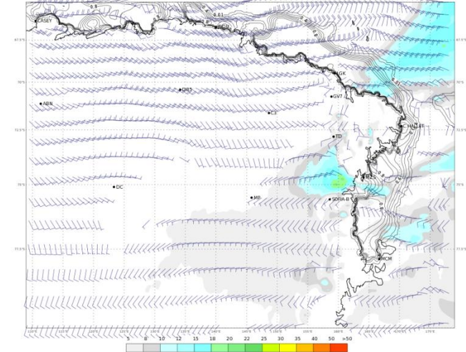
ECMWF 12 Gennaio 2018 00UTC Forecast T+24 VT: Sabato 13 Gennaio 2018 00UTC Terra Vittoria - Wind at 10 m (kts)
