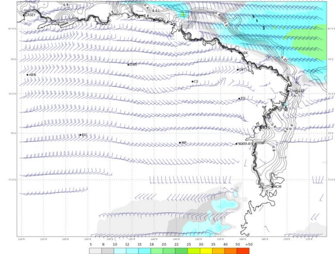
ECMWF 12 Gennaio 2018 00UTC Forecast T+54 VT: Domenica 14 Gennaio 2018 06UTC Terra Vittoria - Wind at 10 m (kts)
