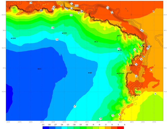
ECMWF 12 Gennaio 2018 00UTC Forecast T+30 VT: Sabato 13 Gennaio 2018 06UTC Terra Vittoria - Temperature at 2 m (°C)
