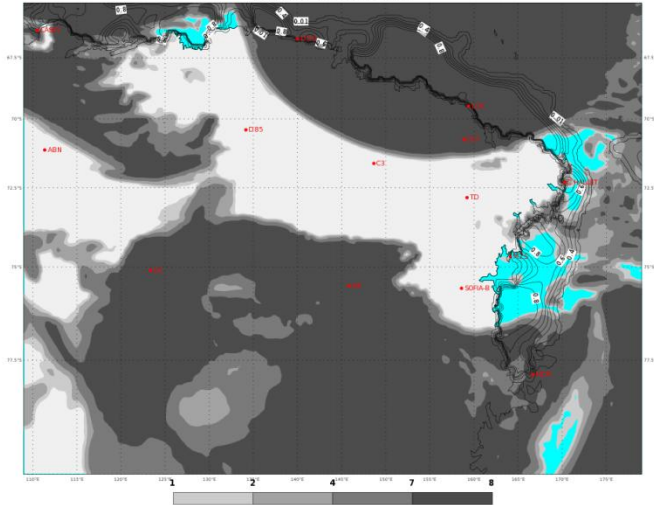
ECMWF 12 Gennaio 2018 00UTC Forecast T+18 VT: Venerdì 12 Gennaio 2018 18UTC Terra Vittoria - Total cloud cover (oct)
