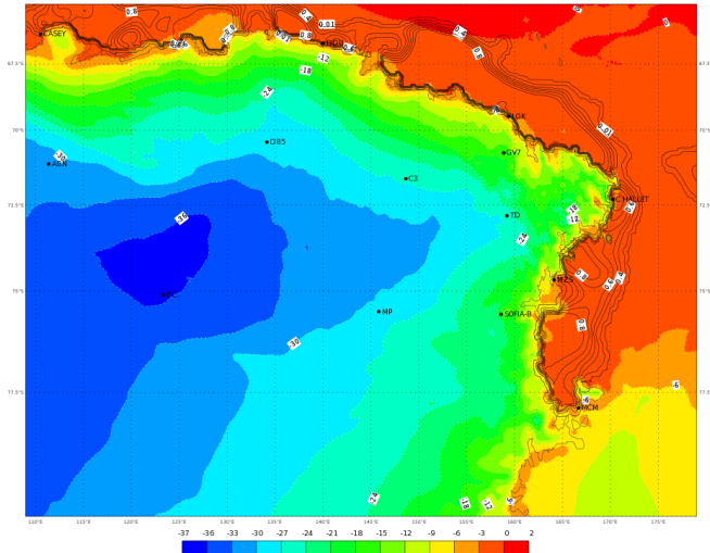
ECMWF 12 Gennaio 2018 00UTC Forecast T+18 VT: Venerdì 12 Gennaio 2018 18UTC Terra Vittoria - temperature at 2 m (°C)
