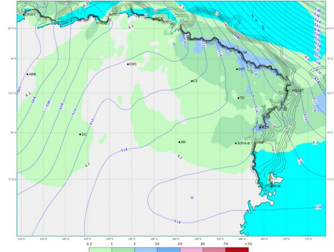
ECMWF 12 Gennaio 2018 00UTC Forecast T+54 VT: Domenica 14 Gennaio 2018 06UTC Terra Vittoria - Geopotential at 500 hPa + 6h accumulated precipitation (mm)
