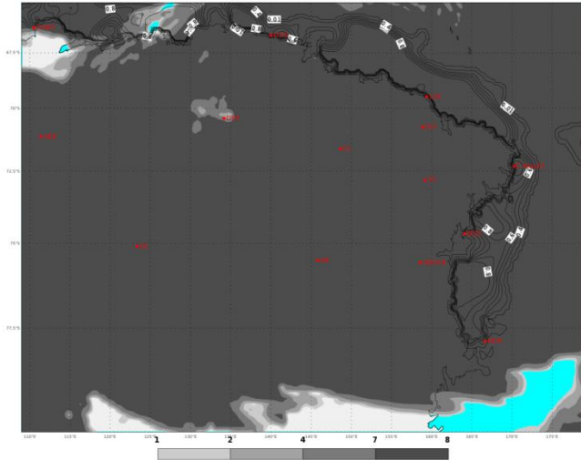
ECMWF 12 Gennaio 2018 00UTC Forecast T+48 VT: Domenica 14 Gennaio 2018 00UTC Terra Vittoria - Total cloud cover (oct)
