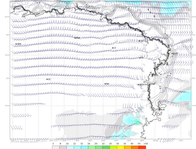
ECMWF 12 Gennaio 2018 00UTC Forecast T+42 VT: Sabato 13 Gennaio 2018 18UTC Terra Vittoria - Wind at 10 m (kts)
