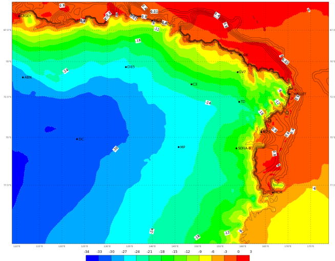
ECMWF 12 Gennaio 2018 00UTC Forecast T+24 VT: Sabato 13 Gennaio 2018 00UTC Terra Vittoria - Temperature at 2 m (°C)
