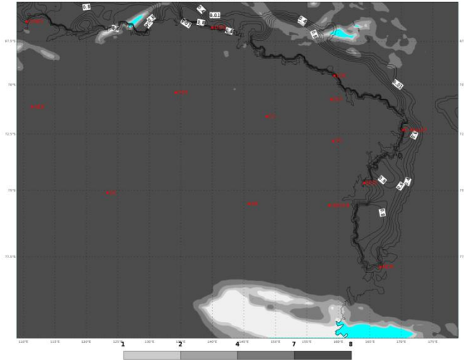
ECMWF 12 Gennaio 2018 00UTC Forecast T+54 VT: Domenica 14 Gennaio 2018 06UTC Terra Vittoria - Total cloud cover (oct)
