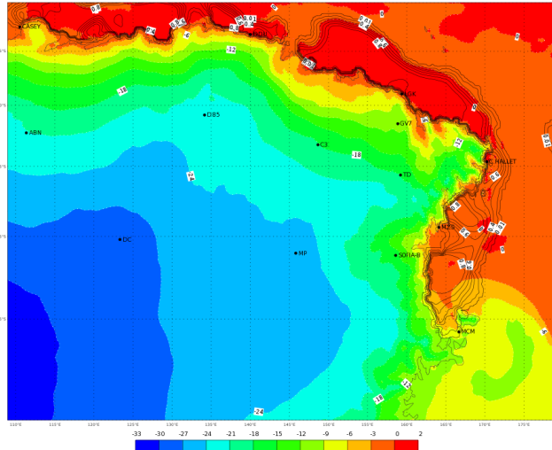
ECMWF 15 Gennaio 2018 00UTC Forecast T+54 VT: Mercoledì 17 Gennaio 2018 06UTC Terra Vittoria - Temperature at 2 m (°C)
