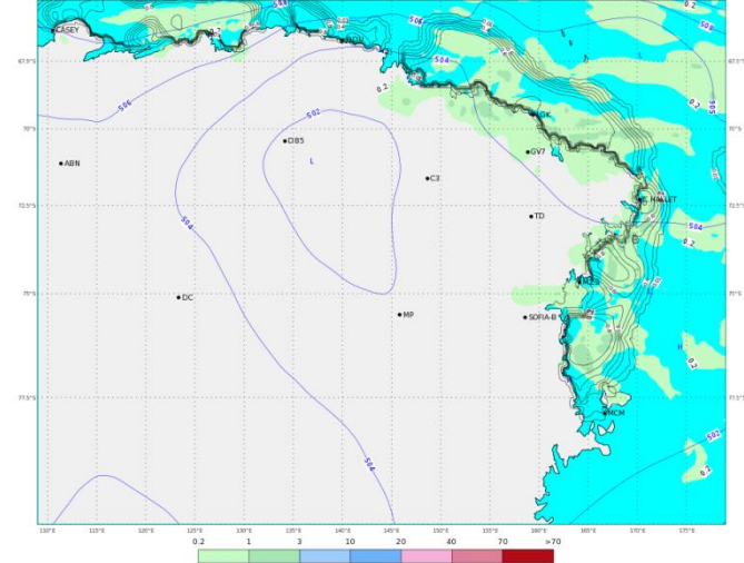
ECMWF 15 Gennaio 2018 00UTC Forecast T+54 VT: Mercoledì 17 Gennaio 2018 06UTC Terra Vittoria - Geopotential at 500 hPa + 6h accumulated precipitation (mm)
