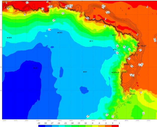
ECMWF 15 Gennaio 2018 00UTC Forecast T+36 VT: Martedì 16 Gennaio 2018 12UTC Terra Vittoria - Temperature at 2 m (°C)
