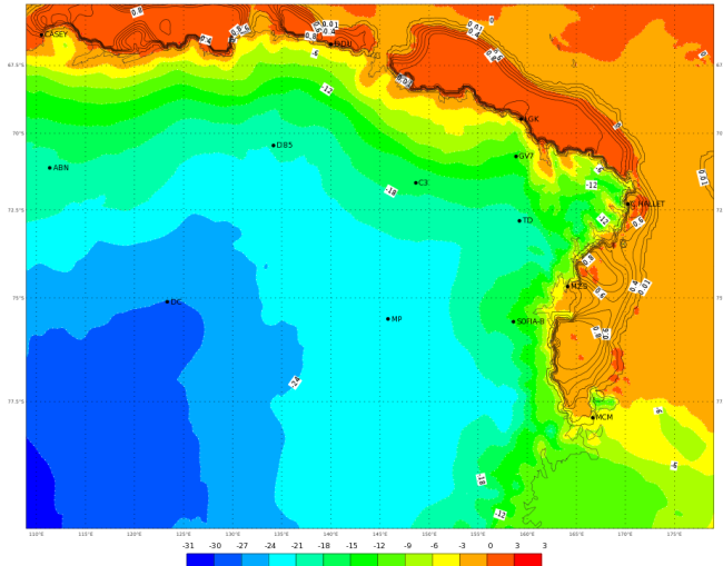
ECMWF 15 Gennaio 2018 00UTC Forecast T+30 VT: Martedì 16 Gennaio 2018 06UTC Terra Vittoria - Temperature at 2 m (°C)
