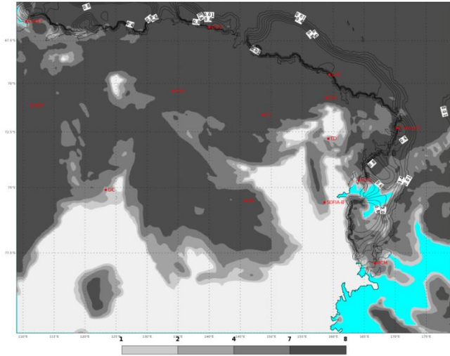
ECMWF 15 Gennaio 2018 00UTC Forecast T+18 VT: Lunedì 15 Gennaio 2018 18UTC Terra Vittoria - total cloud cover (oct)
