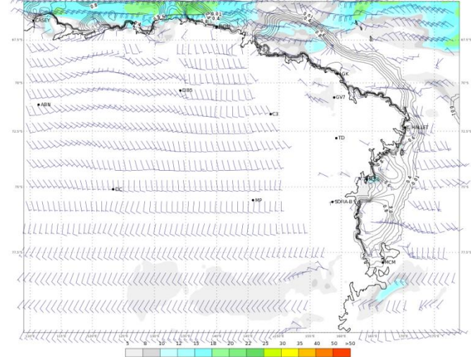
ECMWF 15 Gennaio 2018 00UTC Forecast T+54 VT: Mercoledì 17 Gennaio 2018 06UTC Terra Vittoria - Wind at 10 m (kts)
