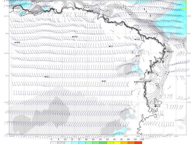
ECMWF 15 Gennaio 2018 00UTC Forecast T+36 VT: Martedì 16 Gennaio 2018 12UTC Terra Vittoria - Wind at 10 m (kts)
