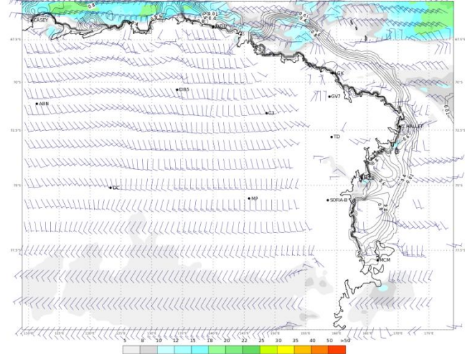
ECMWF 15 Gennaio 2018 00UTC Forecast T+48 VT: Mercoledì 17 Gennaio 2018 00UTC Terra Vittoria - Wind at 10 m (kts)
