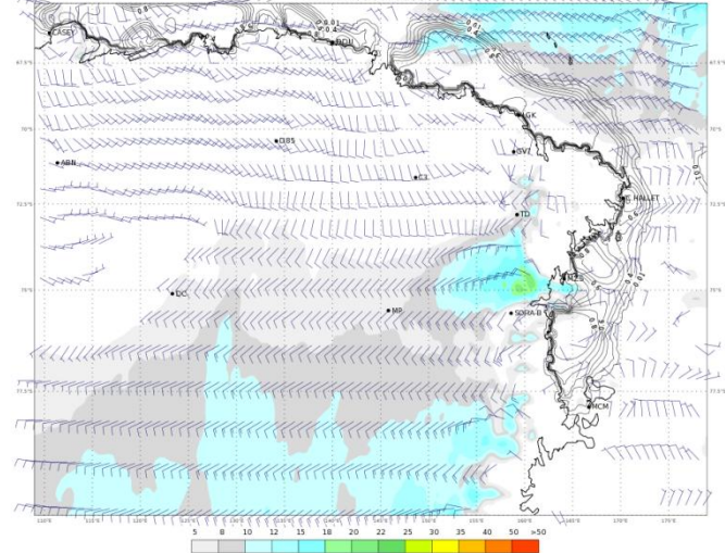
ECMWF 15 Gennaio 2018 00UTC Forecast T+18 VT: Lunedì 15 Gennaio 2018 18UTC Terra Vittoria - Wind at 10 m (kts)
