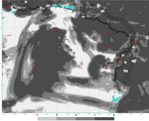
ECMWF 15 Gennaio 2018 00UTC Forecast T+54 VT: Mercoledì 17 Gennaio 2018 06UTC Terra Vittoria - Total cloud cover (oct)
