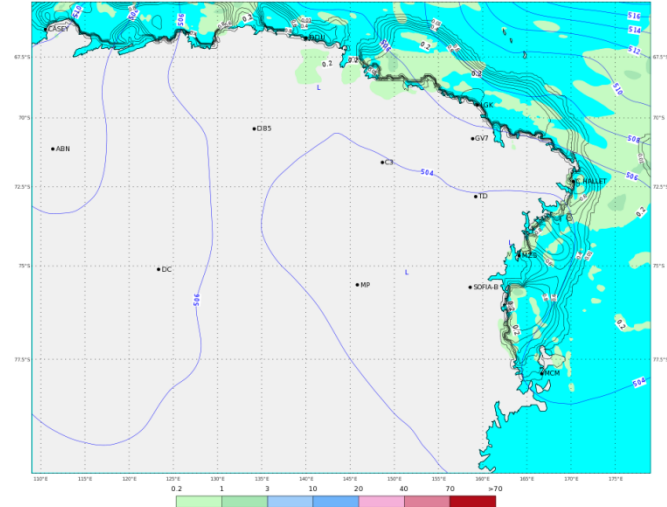
ECMWF 15 Gennaio 2018 00UTC Forecast T+30 VT: Martedì 16 Gennaio 2018 06UTC Terra Vittoria - Geopotential at 500 hPa + 6h accumulated precipitation (mm)
