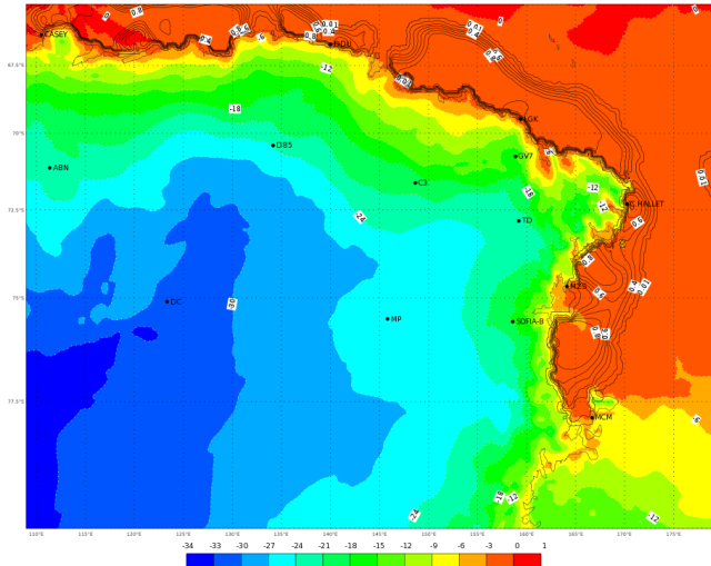
ECMWF 15 Gennaio 2018 00UTC Forecast T+18 VT: Lunedì 15 Gennaio 2018 18UTC Terra Vittoria - temperature at 2 m (°C)
