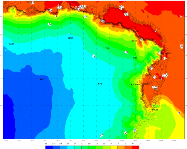
ECMWF 15 Gennaio 2018 00UTC Forecast T+48 VT: Mercoledì 17 Gennaio 2018 00UTC Terra Vittoria - Temperature at 2 m (°C)
