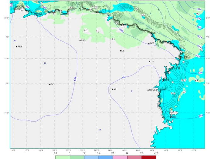
ECMWF 15 Gennaio 2018 00UTC Forecast T+18 VT: Lunedì 15 Gennaio 2018 18UTC Terra Vittoria - Geopotential at 500 hPa + 6h accumulated precipitation (mm)
