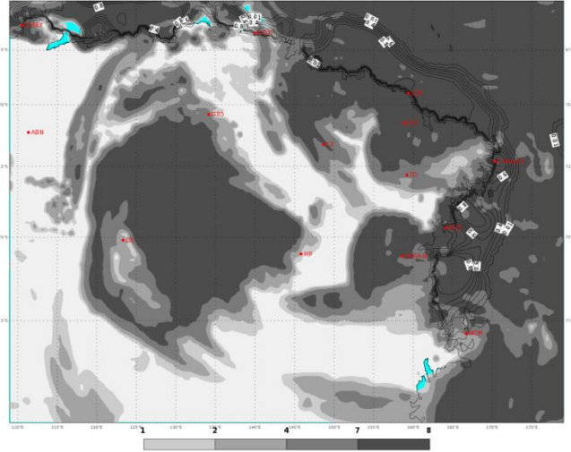
ECMWF 15 Gennaio 2018 00UTC Forecast T+48 VT: Mercoledì 17 Gennaio 2018 00UTC Terra Vittoria - Total cloud cover (oct)
