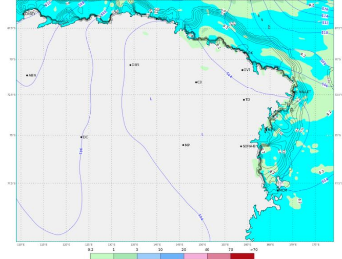
ECMWF 15 Gennaio 2018 00UTC Forecast T+36 VT: Martedì 16 Gennaio 2018 12UTC Terra Vittoria - Geopotential at 500 hPa + 6h accumulated precipitation (mm)
