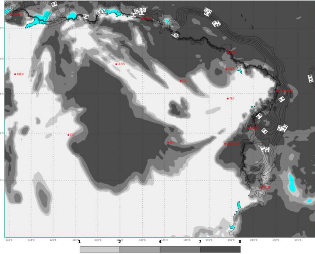
ECMWF 15 Gennaio 2018 00UTC Forecast T+36 VT: Martedì 16 Gennaio 2018 12UTC Terra Vittoria - Total cloud cover (oct)
