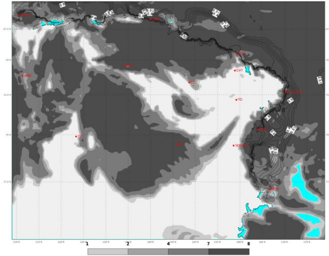
ECMWF 15 Gennaio 2018 00UTC Forecast T+30 VT: Martedì 16 Gennaio 2018 06UTC Terra Vittoria - Total cloud cover (oct)
