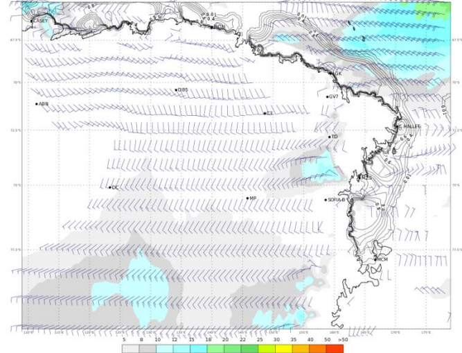
ECMWF 15 Gennaio 2018 00UTC Forecast T+30 VT: Martedì 16 Gennaio 2018 06UTC Terra Vittoria - Wind at 10 m (kts)
