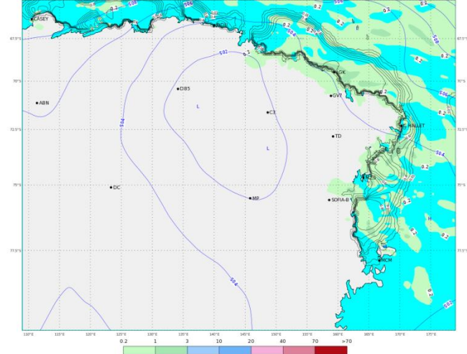
ECMWF 15 Gennaio 2018 00UTC Forecast T+48 VT: Mercoledì 17 Gennaio 2018 00UTC Terra Vittoria - Geopotential at 500 hPa + 6h accumulated precipitation (mm)
