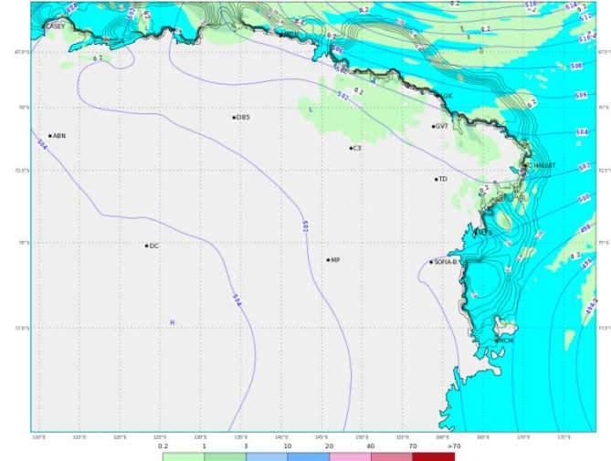
ECMWF 17 Gennaio 2018 00UTC Forecast T+42 VT: Giovedì 18 Gennaio 2018 18UTC Terra Vittoria - Geopotential at 500 hPa + 6h accumulated precipitation (mm)
