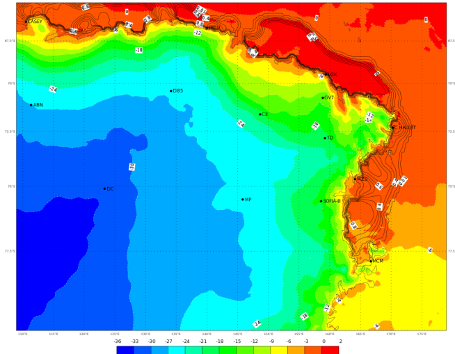
ECMWF 17 Gennaio 2018 00UTC Forecast T+24 VT; Giovedì 18 Gennaio 2018 00UTC Terra Vittoria - Temperature at 2 m (°C)
