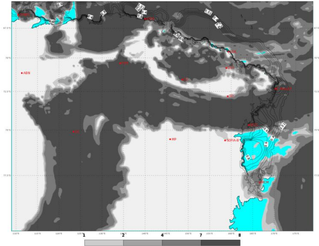
ECMWF 17 Gennaio 2018 00UTC Forecast T+54 VT: Venerdì 19 Gennaio 2018 06UTC Terra Vittoria - Total cloud cover (oct)
