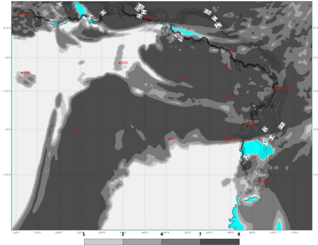
ECMWF 17 Gennaio 2018 00UTC Forecast T+42 VT: Giovedì 18 Gennaio 2018 18UTC Terra Vittoria - Total cloud cover (oct)
