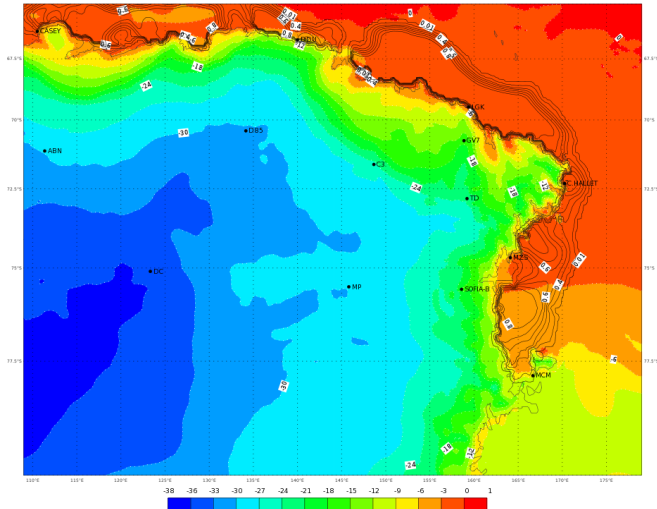
ECMWF 17 Gennaio 2018 00UTC Forecast T+18 VT: Mercoledì 17 Gennaio 2018 18UTC Terra Vittoria - temperature at 2 m (°C)
