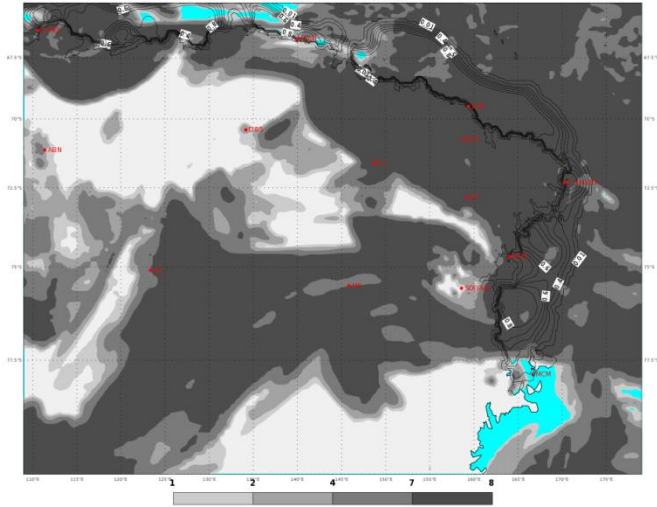
ECMWF 17 Gennaio 2018 00UTC Forecast T+18 VT: Mercoledì 17 Gennaio 2018 18UTC Terra Vittoria - Total cloud cover (oct)
