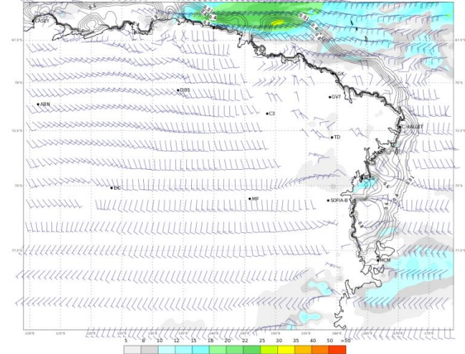
ECMWF 17 Gennaio 2018 00UTC Forecast T+24 VT; Giovedì 18 Gennaio 2018 00UTC Terra Vittoria - Wind at 10 m (kts)
