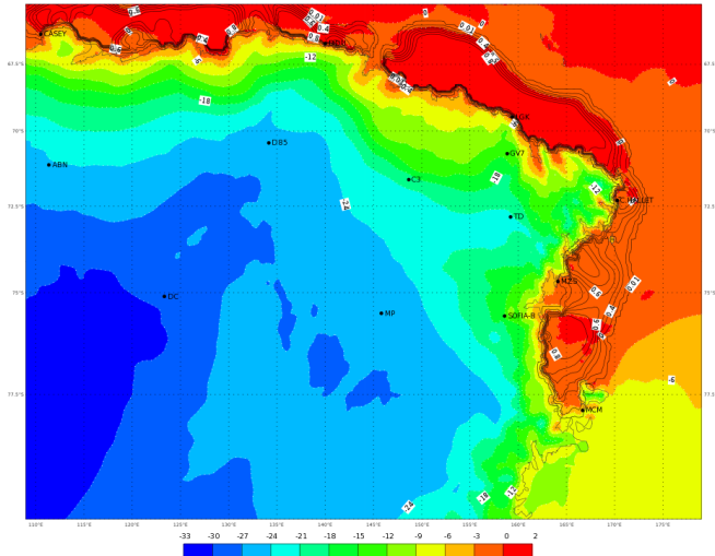
ECMWF 17 Gennaio 2018 00UTC Forecast T+54 VT: Venerdì 19 Gennaio 2018 06UTC Terra Vittoria - Temperature at 2 m (°C)
