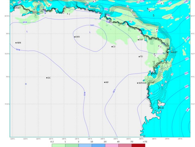
ECMWF 17 Gennaio 2018 00UTC Forecast T+30 VT; Giovedì 18 Gennaio 2018 06UTC Terra Vittoria - Geopotential at 500 hPa + 6h accumulated precipitation (mm)
