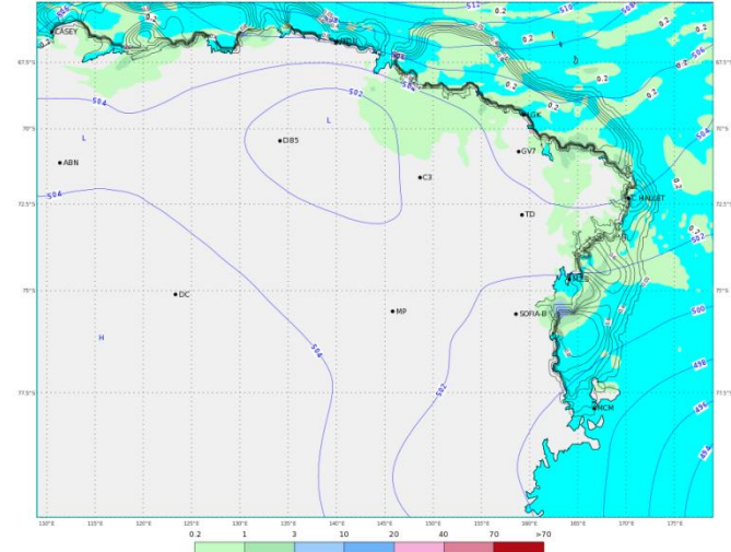
ECMWF 17 Gennaio 2018 00UTC Forecast T+24 VT; Giovedì 18 Gennaio 2018 00UTC Terra Vittoria - Geopotential at 500 hPa + 6h accumulated precipitation (mm)
