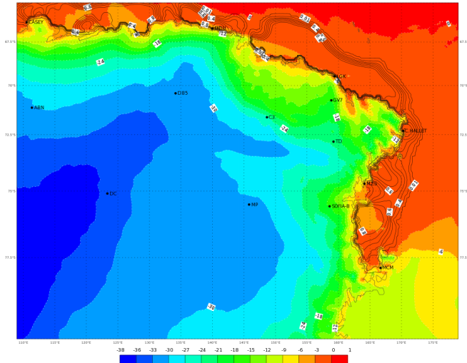
ECMWF 17 Gennaio 2018 00UTC Forecast T+42 VT: Giovedì 18 Gennaio 2018 18UTC Terra Vittoria - Temperature at 2 m (°C)
