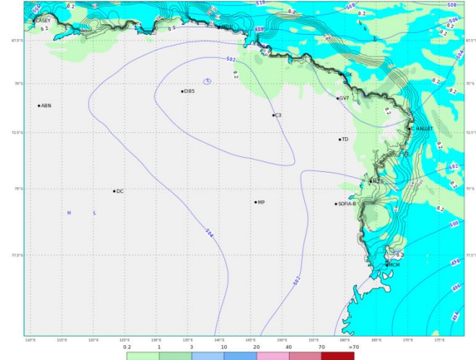
ECMWF 17 Gennaio 2018 00UTC Forecast T+18 VT: Mercoledì 17 Gennaio 2018 18UTC Terra Vittoria - Geopotential at 500 hPa + 6h accumulated precipitation (mm)
