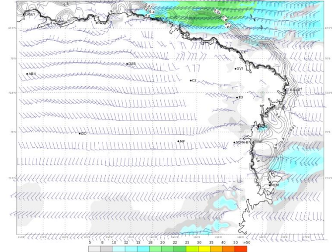
ECMWF 17 Gennaio 2018 00UTC Forecast T+30 VT; Giovedì 18 Gennaio 2018 06UTC Terra Vittoria - Wind at 10 m (kts)
