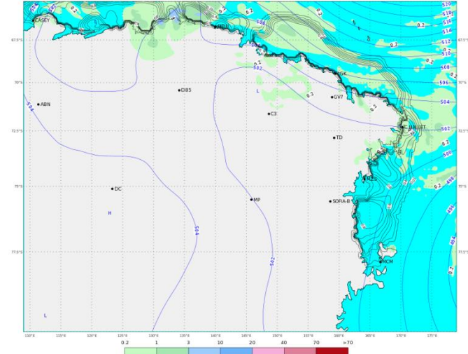
ECMWF 17 Gennaio 2018 00UTC Forecast T+54 VT: Venerdì 19 Gennaio 2018 06UTC Terra Vittoria - Geopotential at 500 hPa + 6h accumulated precipitation (mm)
