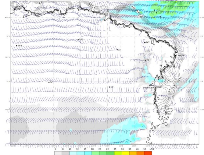
ECMWF 17 Gennaio 2018 00UTC Forecast T+42 VT: Giovedì 18 Gennaio 2018 18UTC Terra Vittoria - Wind at 10 m (kts)
