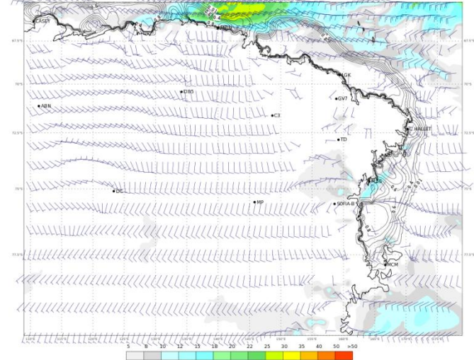
ECMWF 17 Gennaio 2018 00UTC Forecast T+18 VT: Mercoledì 17 Gennaio 2018 18UTC Terra Vittoria - Wind at 10 m (kts)
