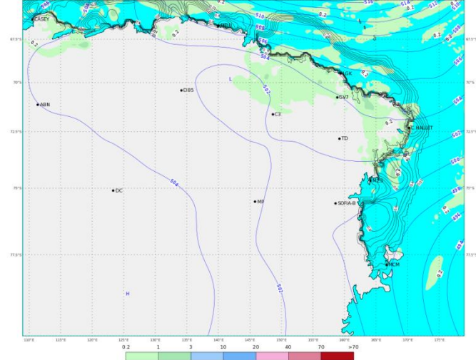
ECMWF 17 Gennaio 2018 00UTC Forecast T+36 VT: Giovedì 18 Gennaio 2018 12UTC Terra Vittoria - Geopotential at 500 hPa + 6h accumulated precipitation (mm)
