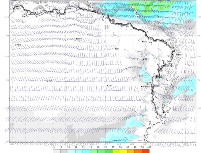
ECMWF 17 Gennaio 2018 00UTC Forecast T+36 VT: Giovedì 18 Gennaio 2018 12UTC Terra Vittoria - Wind at 10 m (kts)
