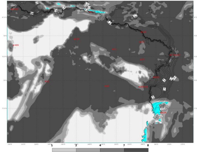
ECMWF 17 Gennaio 2018 00UTC Forecast T+24 VT; Giovedì 18 Gennaio 2018 00UTC Terra Vittoria - Total cloud cover (oct)
