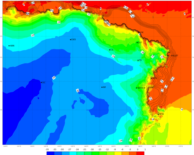
ECMWF 17 Gennaio 2018 00UTC Forecast T+36 VT: Giovedì 18 Gennaio 2018 12UTC Terra Vittoria - Temperature at 2 m (°C)
