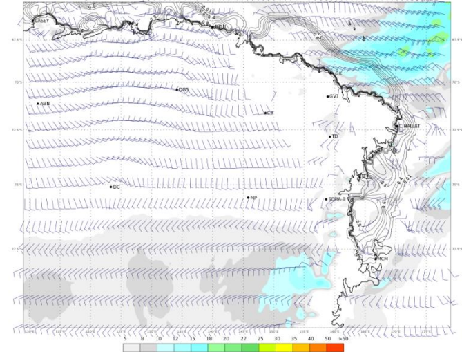
ECMWF 17 Gennaio 2018 00UTC Forecast T+54 VT: Venerdì 19 Gennaio 2018 06UTC Terra Vittoria - Wind at 10 m (kts)
