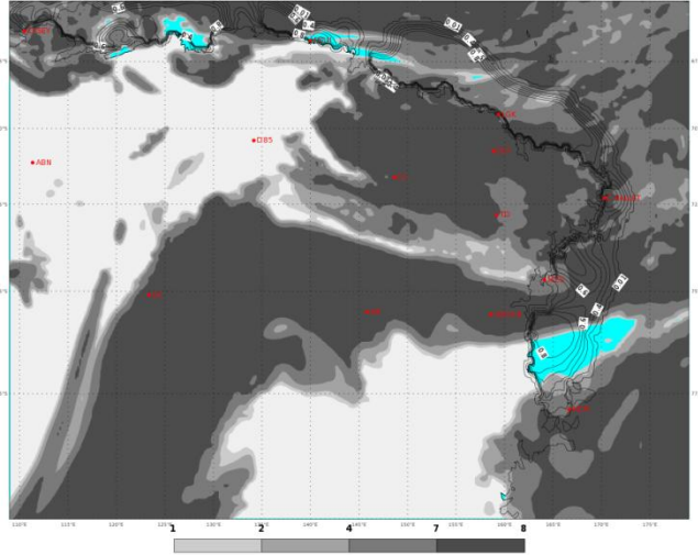
ECMWF 17 Gennaio 2018 00UTC Forecast T+36 VT: Giovedì 18 Gennaio 2018 12UTC Terra Vittoria - Total cloud cover (oct)
