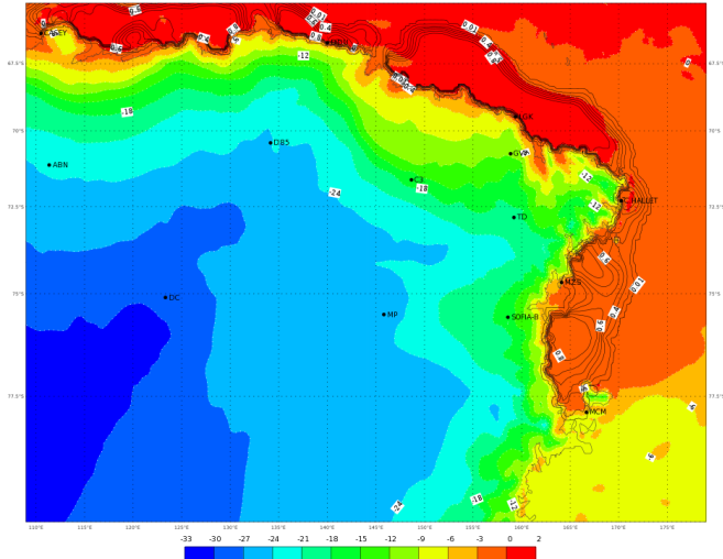
ECMWF 17 Gennaio 2018 00UTC Forecast T+30 VT; Giovedì 18 Gennaio 2018 06UTC Terra Vittoria - Temperature at 2 m (°C)
