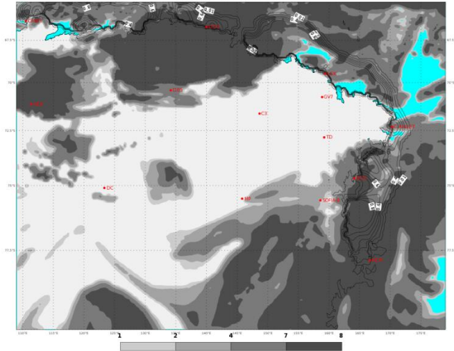
ECMWF 20 Gennaio 2018 00UTC Forecast T+30 VT: Domenica 21 Gennaio 2018 06UTC Terra Vittoria - Total cloud cover (oct)
