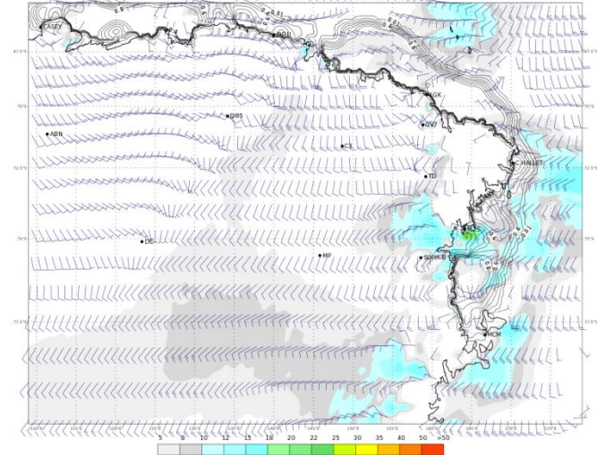
ECMWF 20 Gennaio 2018 00UTC Forecast T+18 VT: Sabato 20 Gennaio 2018 18UTC Terra Vittoria - Wind at 10 m (kts)
