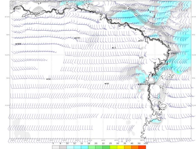
ECMWF 20 Gennaio 2018 00UTC Forecast T+30 VT: Domenica 21 Gennaio 2018 06UTC Terra Vittoria - Wind at 10 m (kts)
