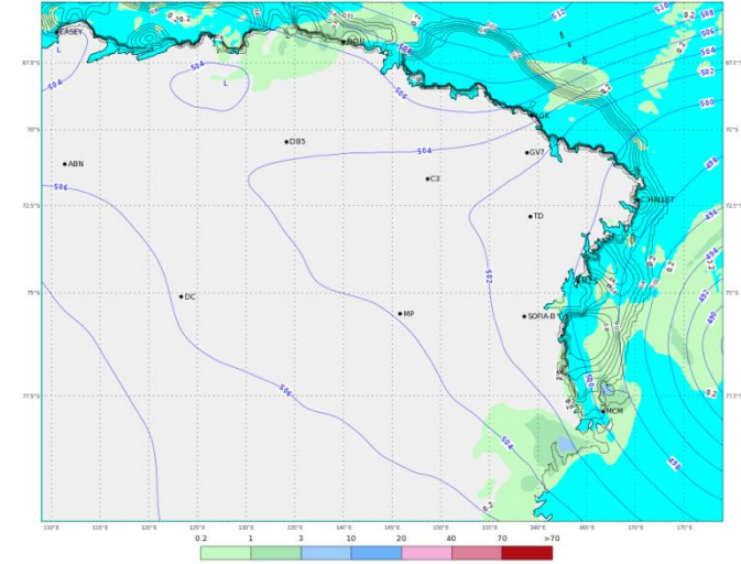
ECMWF 20 Gennaio 2018 00UTC Forecast T+36 VT: Domenica 21 Gennaio 12UTC Terra Vittoria - Geopotential at 500 hPa + 6h accumulated precipitation (mm)
