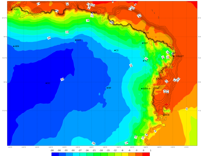
ECMWF 20 Gennaio 2018 00UTC Forecast T+18 VT: Sabato 20 Gennaio 2018 18UTC Terra Vittoria - temperature at 2 m (°C)
