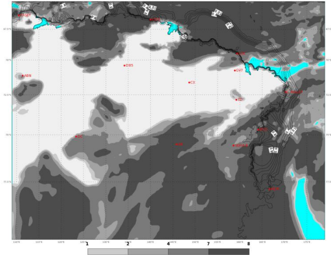
ECMWF 20 Gennaio 2018 00UTC Forecast T+42 VT: Domenica 21 Gennaio 18UTC Terra Vittoria - Total cloud cover (oct)
