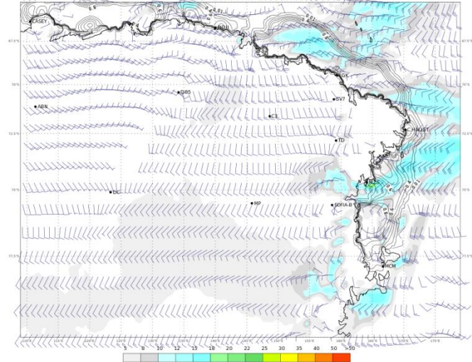
ECMWF 20 Gennaio 2018 00UTC Forecast T+24 VT: Domenica 21 Gennaio 2018 00UTC Terra Vittoria - Wind at 10 m (kts)
