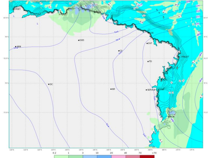
ECMWF 20 Gennaio 2018 00UTC Forecast T+24 VT: Domenica 21 Gennaio 2018 00UTC Terra Vittoria - Geopotential at 500 hPa + 6h accumulated precipitation (mm)
