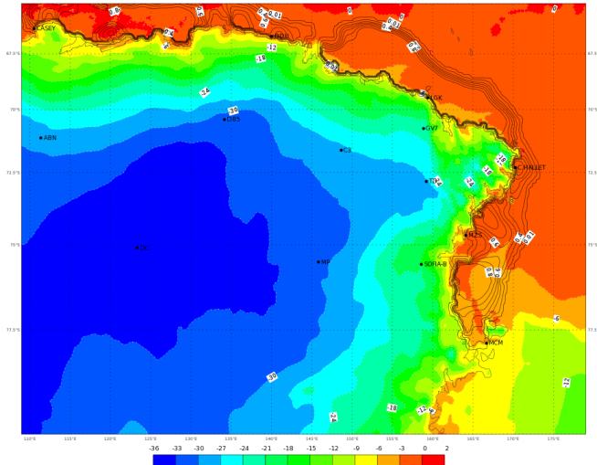
ECMWF 20 Gennaio 2018 00UTC Forecast T+36 VT: Domenica 21 Gennaio 12UTC Terra Vittoria - Temperature at 2 m (°C)
