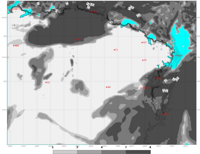
ECMWF 20 Gennaio 2018 00UTC Forecast T+24 VT: Domenica 21 Gennaio 2018 00UTC Terra Vittoria - Total cloud cover (oct)
