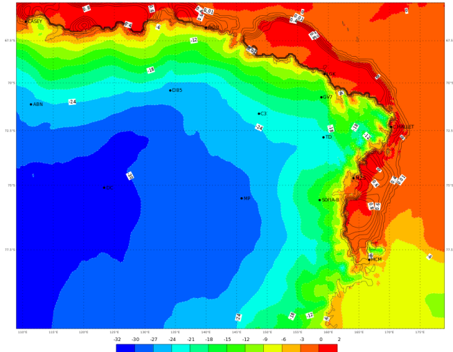
ECMWF 20 Gennaio 2018 00UTC Forecast T+30 VT: Domenica 21 Gennaio 2018 06UTC Terra Vittoria - Temperature at 2 m (°C)
