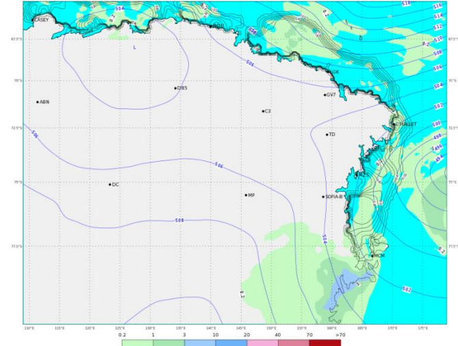
ECMWF 20 Gennaio 2018 00UTC Forecast T+54 VT: Lunedì 22 Gennaio 2018 06UTC Terra Vittoria - Geopotential at 500 hPa + 6h accumulated precipitation (mm)
