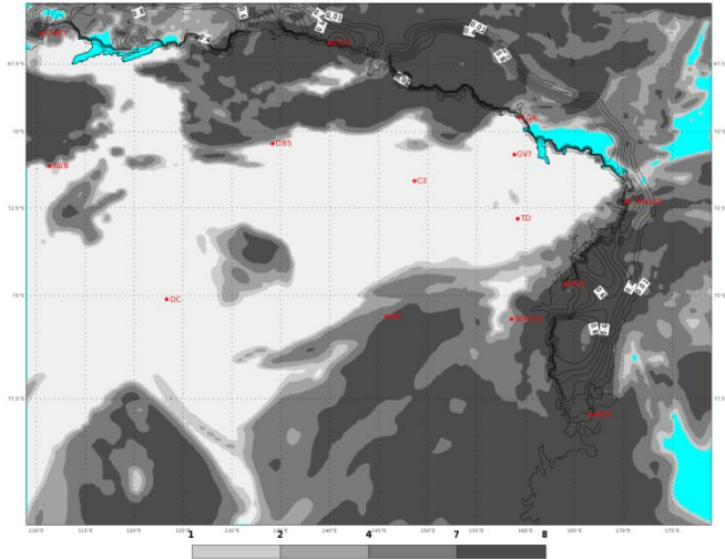
ECMWF 20 Gennaio 2018 00UTC Forecast T+36 VT: Domenica 21 Gennaio 12UTC Terra Vittoria - Total cloud cover (oct)
