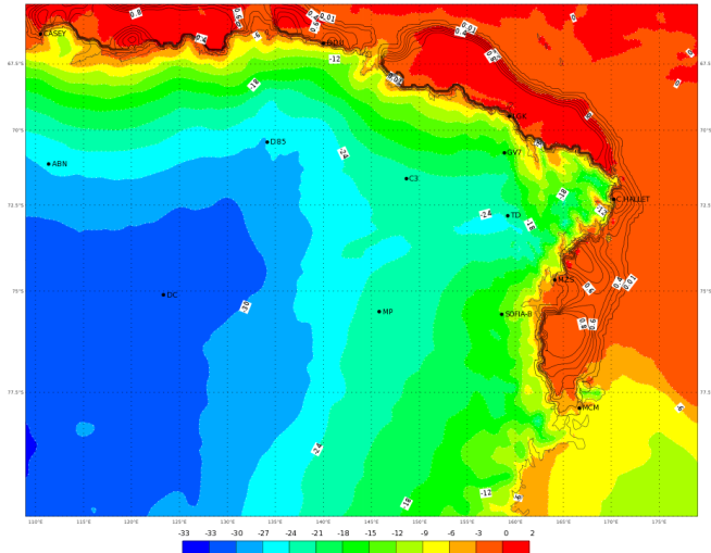
ECMWF 20 Gennaio 2018 00UTC Forecast T+54 VT: Lunedì 22 Gennaio 2018 06UTC Terra Vittoria - Temperature at 2 m (°C)
