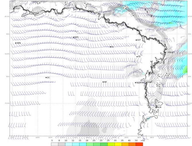
ECMWF 20 Gennaio 2018 00UTC Forecast T+54 VT: Lunedì 22 Gennaio 2018 06UTC Terra Vittoria - Wind at 10 m (kts)
