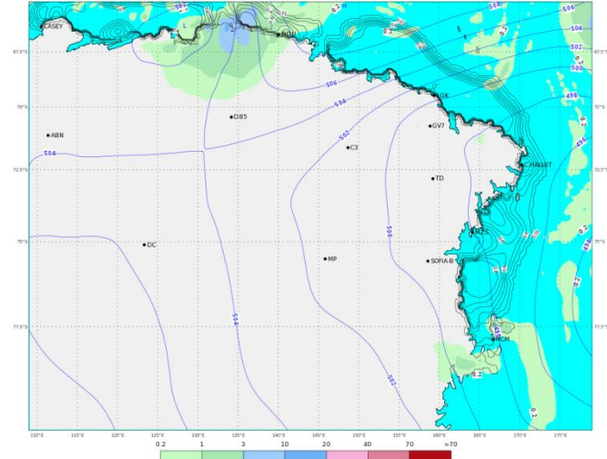
ECMWF 20 Gennaio 2018 00UTC Forecast T+18 VT: Sabato 20 Gennaio 2018 18UTC Terra Vittoria - Geopotential at 500 hPa + 6h accumulated precipitation (mm)
