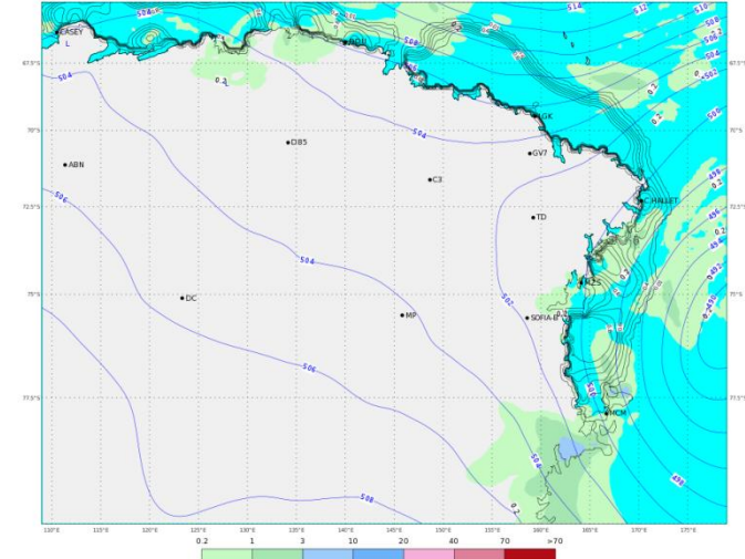
ECMWF 20 Gennaio 2018 00UTC Forecast T+42 VT: Domenica 21 Gennaio 18UTC Terra Vittoria - Geopotential at 500 hPa + 6h accumulated precipitation (mm)
