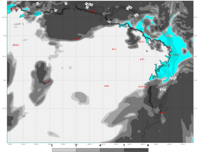
ECMWF 20 Gennaio 2018 00UTC Forecast T+18 VT: Sabato 20 Gennaio 2018 18UTC Terra Vittoria - Total cloud cover (oct)
