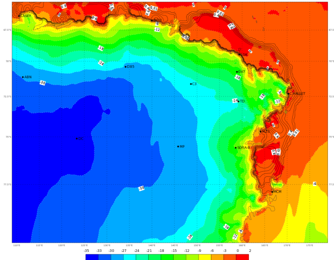
ECMWF 20 Gennaio 2018 00UTC Forecast T+24 VT: Domenica 21 Gennaio 2018 00UTC Terra Vittoria - Temperature at 2 m (°C)
