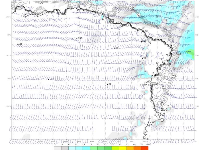
ECMWF 20 Gennaio 2018 00UTC Forecast T+36 VT: Domenica 21 Gennaio 12UTC Terra Vittoria - Wind at 10 m (kts)
