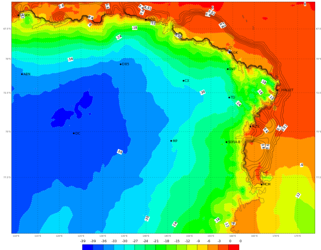
ECMWF 20 Gennaio 2018 00UTC Forecast T+42 VT: Domenica 21 Gennaio 18UTC Terra Vittoria - Temperature at 2 m (°C)
