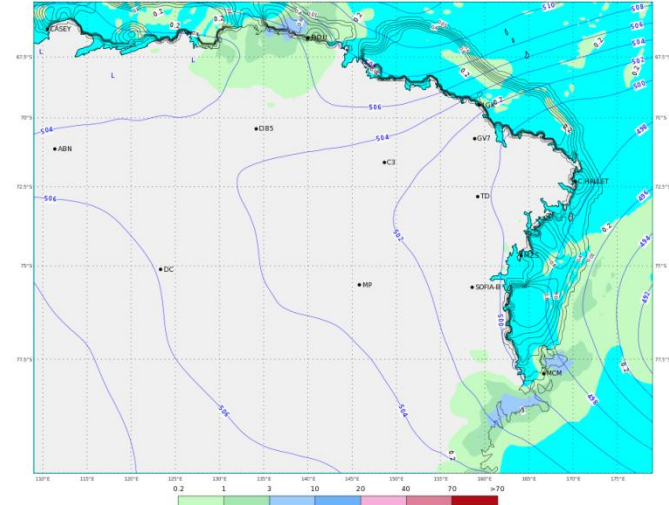
ECMWF 20 Gennaio 2018 00UTC Forecast T+30 VT: Domenica 21 Gennaio 2018 06UTC Terra Vittoria - Geopotential at 500 hPa + 6h accumulated precipitation (mm)
