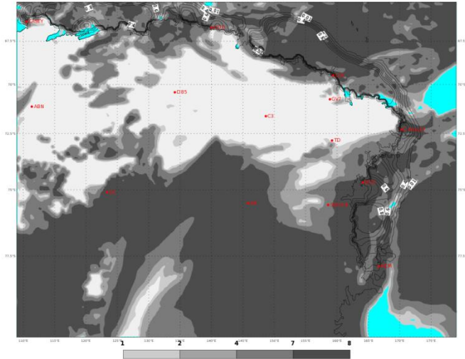
ECMWF 20 Gennaio 2018 00UTC Forecast T+54 VT: Lunedì 22 Gennaio 2018 06UTC Terra Vittoria - Total cloud cover (oct)
