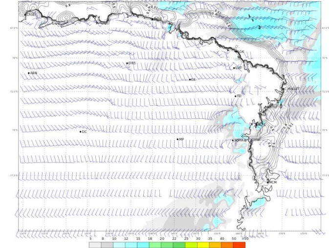
ECMWF 20 Gennaio 2018 00UTC Forecast T+42 VT: Domenica 21 Gennaio 18UTC Terra Vittoria - Wind at 10 m (kts)
