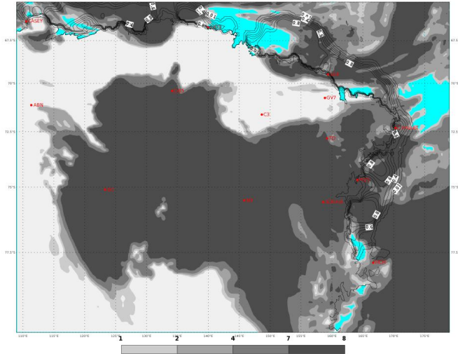
ECMWF 25 Gennaio 2018 00UTC Forecast T+24 VT: Venerdì 26 Gennaio 2018 00UTC Terra Vittoria - total cloud cover (oct)
