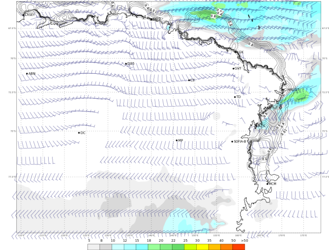
ECMWF 25 Gennaio 2018 00UTC Forecast T+24 VT: Venerdì 26 Gennaio 2018 00UTC Terra Vittoria - Wind at 10 m (kts)
