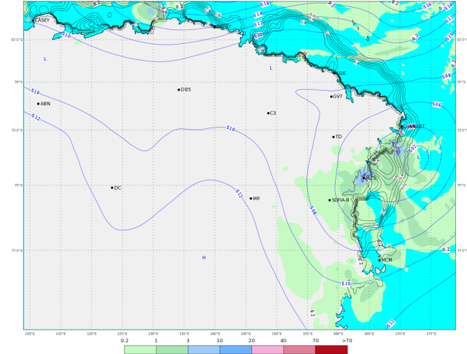
ECMWF 25 Gennaio 2018 00UTC Forecast T+18 VT: Giovedì 25 Gennaio 2018 18UTC Terra Vittoria - Geopotential at 500 hPa + 6h accumulated precipitation (mm)
