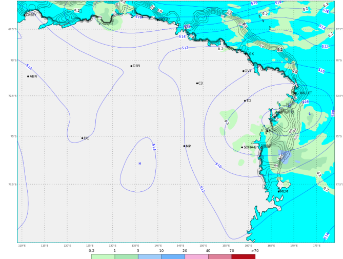
ECMWF 25 Gennaio 2018 00UTC Forecast T+30 VT: Venerdì 26 Gennaio 2018 06UTC Terra Vittoria - Geopotential at 500 hPa + 6h accumulated precipitation (mm)
