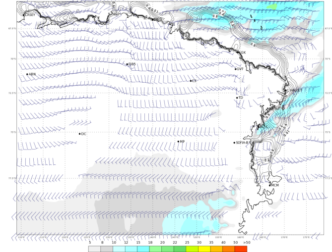
ECMWF 25 Gennaio 2018 00UTC Forecast T+30 VT: Venerdì 26 Gennaio 2018 06UTC Terra Vittoria - Wind at 10 m (kts)
