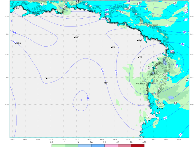
ECMWF 25 Gennaio 2018 00UTC Forecast T+24 VT: Venerdì 26 Gennaio 2018 00UTC Terra Vittoria - Geopotential at 500 hPa + 6h accumulated precipitation (mm)
