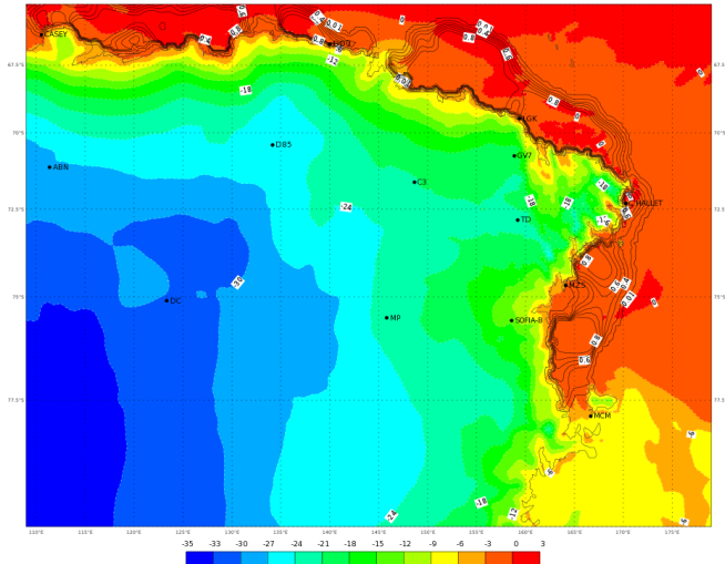
ECMWF 25 Gennaio 2018 00UTC Forecast T+30 VT: Venerdì 26 Gennaio 2018 06UTC Terra Vittoria - Temperature at 2 m (°C)
