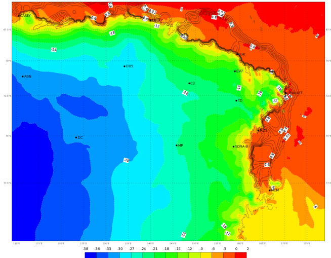
ECMWF 25 Gennaio 2018 00UTC Forecast T+24 VT: Venerdì 26 Gennaio 2018 00UTC Terra Vittoria - temperature at 2 m (°C)
