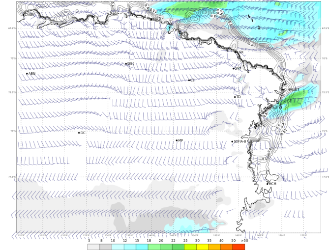
ECMWF 25 Gennaio 2018 00UTC Forecast T+18 VT: Giovedì 25 Gennaio 2018 18UTC Terra Vittoria - Wind at 10 m (kts)
