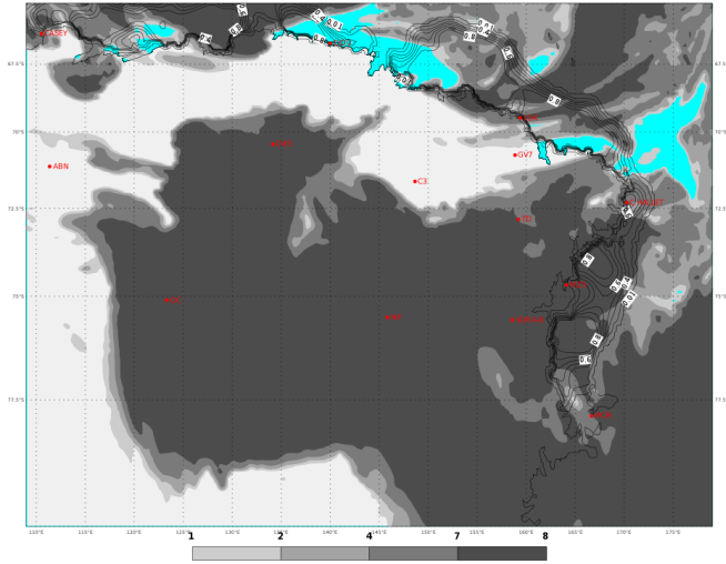
ECMWF 25 Gennaio 2018 00UTC Forecast T+18 VT: Giovedì 25 Gennaio 2018 18UTC Terra Vittoria - total cloud cover (oct)
