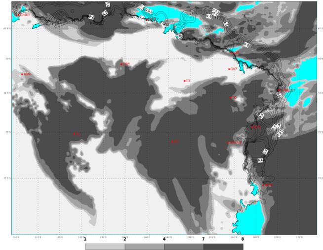
ECMWF 25 Gennaio 2018 00UTC Forecast T+30 VT: Venerdì 26 Gennaio 2018 06UTC Terra Vittoria - Total cloud cover (oct)
