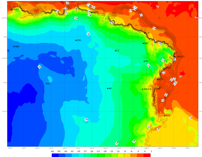
ECMWF 25 Gennaio 2018 00UTC Forecast T+18 VT: Giovedì 25 Gennaio 2018 18UTC Terra Vittoria - temperature at 2 m (°C)
