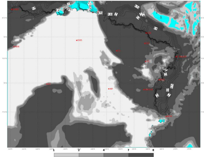
ECMWF 30 Gennaio 2018 00UTC Forecast T+42 VT: Mercoledì 31 Gennaio 2018 18UTC Terra Vittoria - Total cloud cover (oct)
