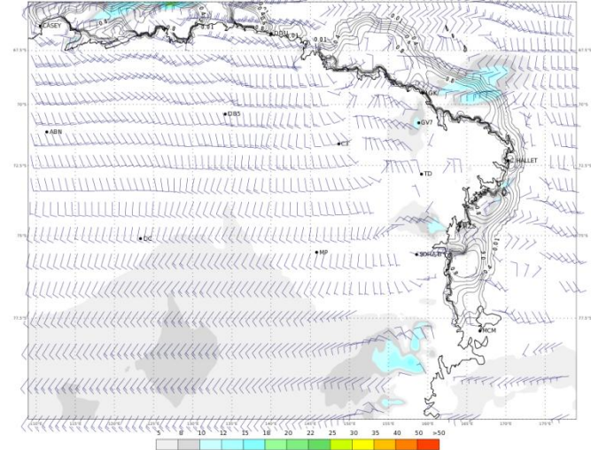
ECMWF 30 Gennaio 2018 00UTC Forecast T+30 VT: Mercoledì 31 Gennaio 2018 06UTC Terra Vittoria - Wind at 10 m (kts)
