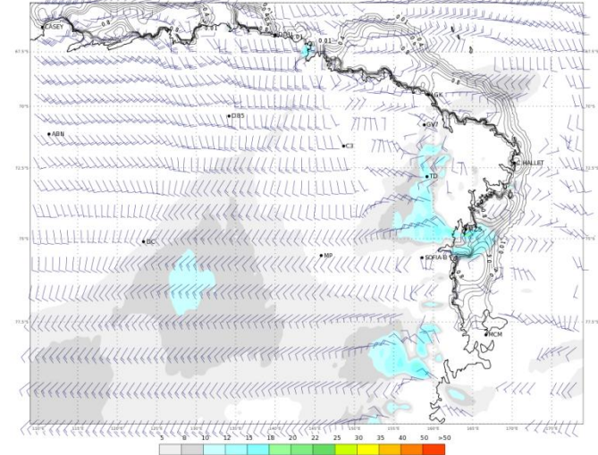
ECMWF 30 Gennaio 2018 00UTC Forecast T+42 VT: Mercoledì 31 Gennaio 2018 18UTC Terra Vittoria - Wind at 10 m (kts)
