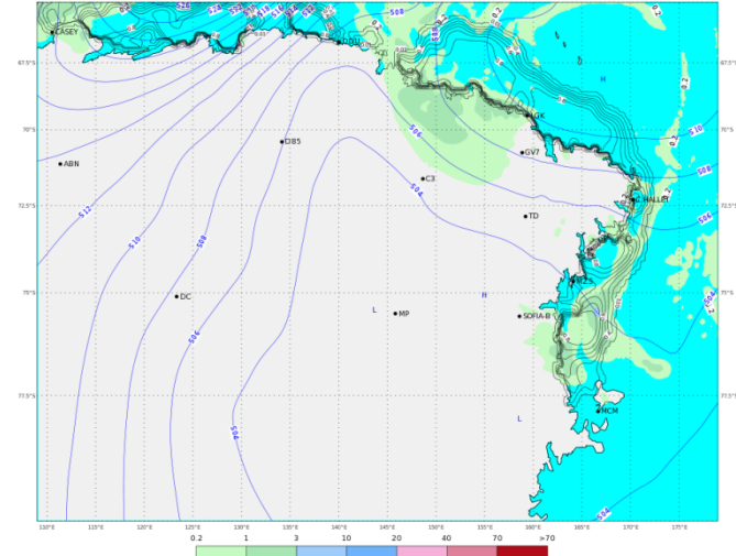
ECMWF 30 Gennaio 2018 00UTC Forecast T+42 VT: Mercoledì 31 Gennaio 2018 18UTC Terra Vittoria - Geopotential at 500 hPa + 6h accumulated precipitation (mm)
