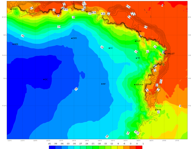
ECMWF 30 Gennaio 2018 00UTC Forecast T+24 VT: Mercoledì 31 Gennaio 2018 00UTC Terra Vittoria - temperature at 2 m (°C)
