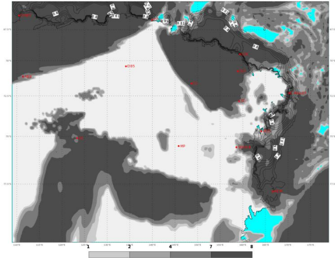
ECMWF 30 Gennaio 2018 00UTC Forecast T+54 VT: Giovedì 01 Febbraio 2018 06UTC Terra Vittoria - Total cloud cover (oct)
