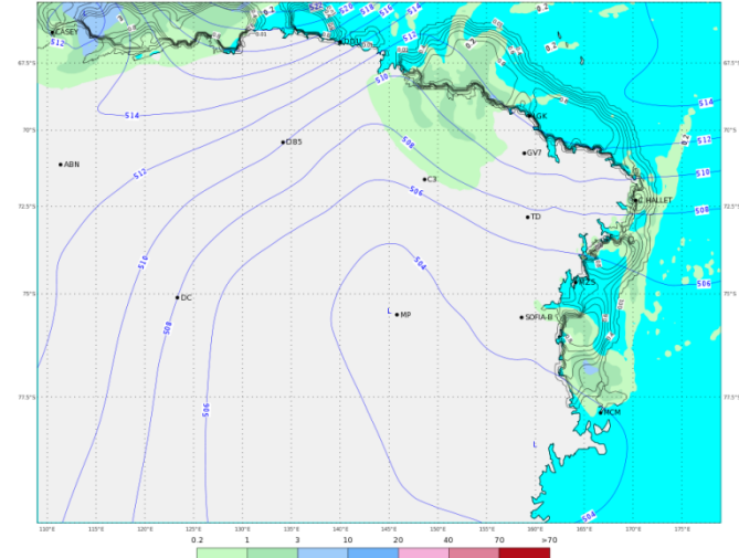
ECMWF 30 Gennaio 2018 00UTC Forecast T+54 VT: Giovedì 01 Febbraio 2018 06UTC Terra Vittoria - Geopotential at 500 hPa + 6h accumulated precipitation (mm)
