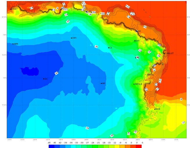
ECMWF 30 Gennaio 2018 00UTC Forecast T+42 VT: Mercoledì 31 Gennaio 2018 18UTC Terra Vittoria - Temperature at 2 m (°C)
