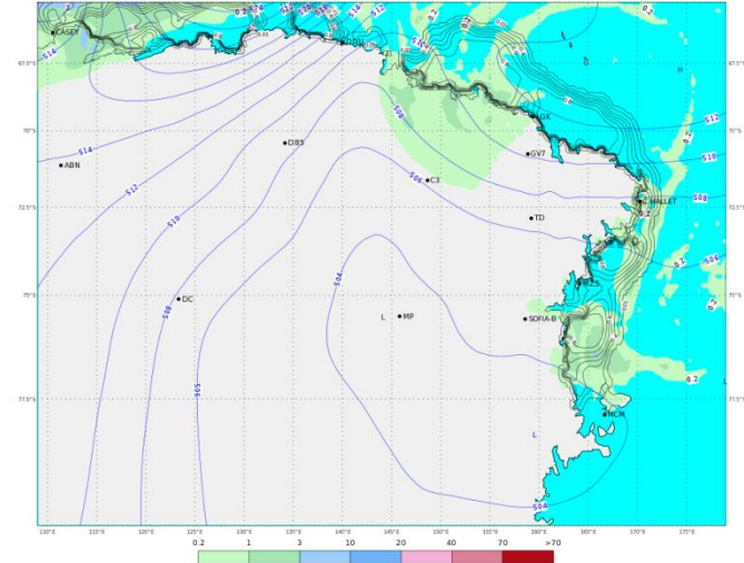
ECMWF 30 Gennaio 2018 00UTC Forecast T+48 VT: Giovedì 01 Febbraio 2018 00UTC Terra Vittoria - Geopotential at 500 hPa + 6h accumulated precipitation (mm)
