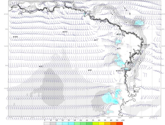
ECMWF 30 Gennaio 2018 00UTC Forecast T+36 VT: Mercoledì 31 Gennaio 2018 12UTC Terra Vittoria - Wind at 10 m (kts)
