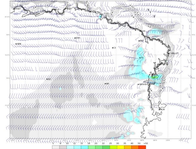
ECMWF 30 Gennaio 2018 00UTC Forecast T+48 VT: Giovedì 01 Febbraio 2018 00UTC Terra Vittoria - Wind at 10 m (kts)
