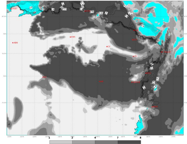
ECMWF 30 Gennaio 2018 00UTC Forecast T+24 VT: Mercoledì 31 Gennaio 2018 00UTC Terra Vittoria - Total cloud cover (oct)
