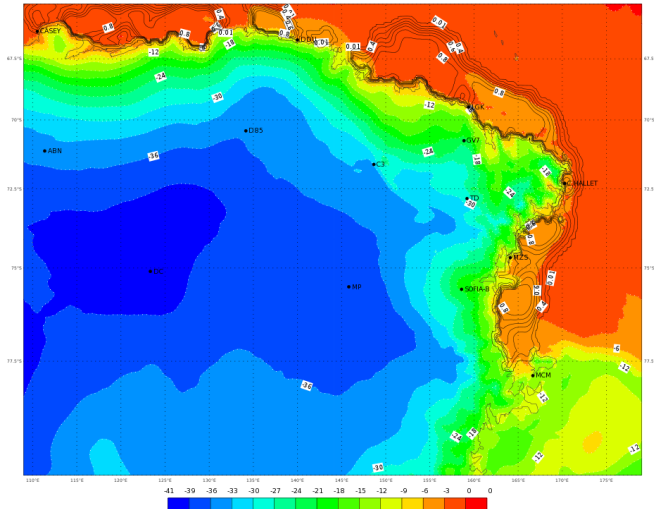
ECMWF 30 Gennaio 2018 00UTC Forecast T+36 VT: Mercoledì 31 Gennaio 2018 12UTC Terra Vittoria - Temperature at 2 m (°C)
