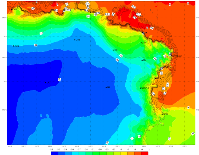
ECMWF 30 Gennaio 2018 00UTC Forecast T+54 VT: Giovedì 01 Febbraio 2018 06UTC Terra Vittoria - Temperature at 2 m (°C)
