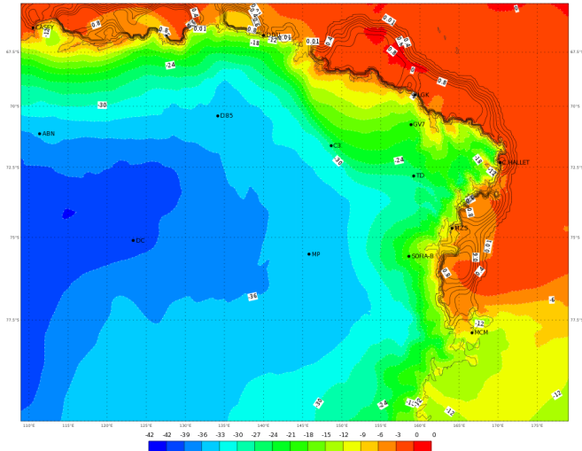
ECMWF 30 Gennaio 2018 00UTC Forecast T+48 VT: Giovedì 01 Febbraio 2018 00UTC Terra Vittoria - temperature at 2 m (°C)
