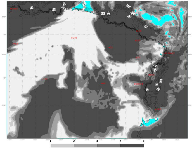
ECMWF 30 Gennaio 2018 00UTC Forecast T+48 VT: Giovedì 01 Febbraio 2018 00UTC Terra Vittoria - Total cloud cover (oct)
