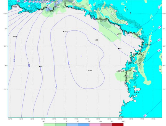
ECMWF 30 Gennaio 2018 00UTC Forecast T+30 VT: Mercoledì 31 Gennaio 2018 06UTC Terra Vittoria - Geopotential at 500 hPa + 6h accumulated precipitation (mm)
