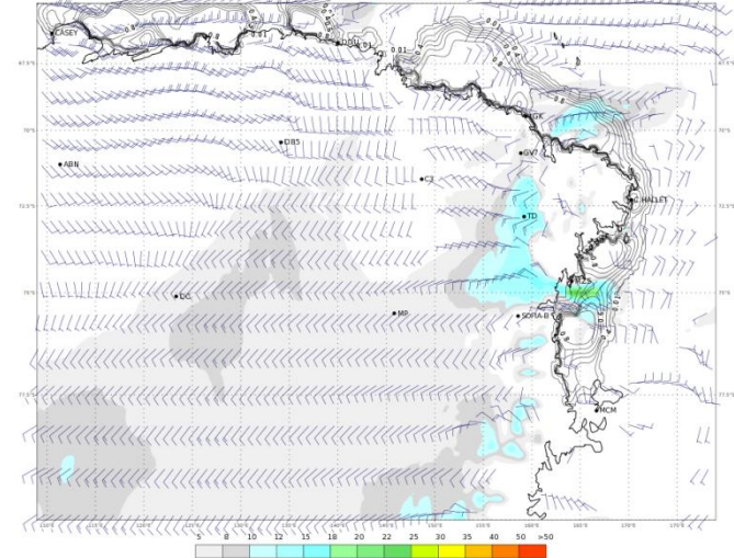
ECMWF 30 Gennaio 2018 00UTC Forecast T+54 VT: Giovedì 01 Febbraio 2018 06UTC Terra Vittoria - Wind at 10 m (kts)
