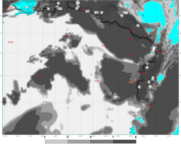
ECMWF 30 Gennaio 2018 00UTC Forecast T+30 VT: Mercoledì 31 Gennaio 2018 06UTC Terra Vittoria - Total cloud cover (oct)
