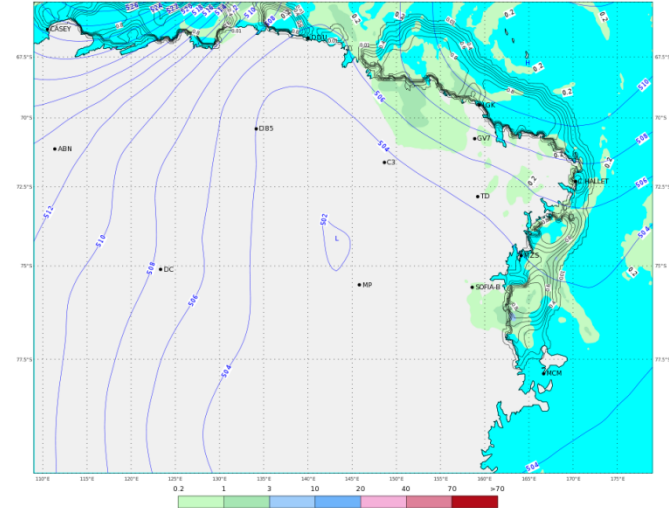
ECMWF 30 Gennaio 2018 00UTC Forecast T+36 VT: Mercoledì 31 Gennaio 2018 12UTC Terra Vittoria - Geopotential at 500 hPa + 6h accumulated precipitation (mm)
