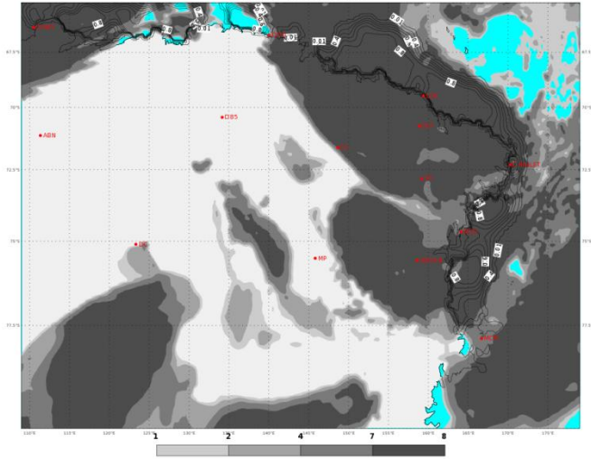
ECMWF 30 Gennaio 2018 00UTC Forecast T+36 VT: Mercoledì 31 Gennaio 2018 12UTC Terra Vittoria - Total cloud cover (oct)
