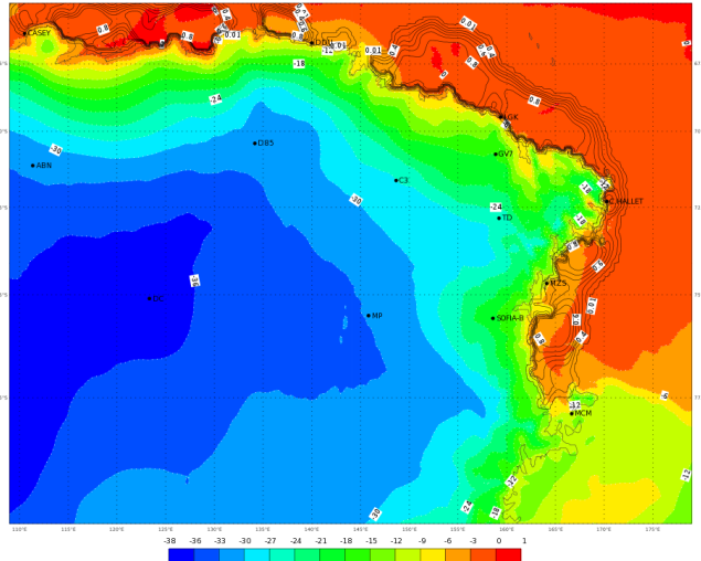
ECMWF 30 Gennaio 2018 00UTC Forecast T+30 VT: Mercoledì 31 Gennaio 2018 06UTC Terra Vittoria - temperature at 2 m (°C)
