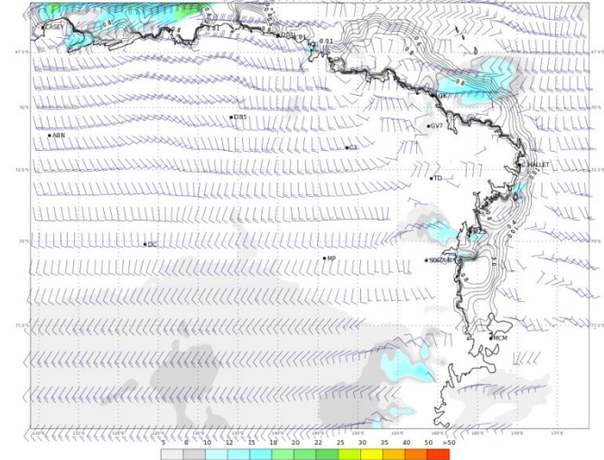
ECMWF 30 Gennaio 2018 00UTC Forecast T+24 VT: Mercoledì 31 Gennaio 2018 00UTC Terra Vittoria - Wind at 10 m (kts)
