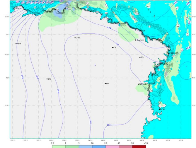
ECMWF 30 Gennaio 2018 00UTC Forecast T+24 VT: Mercoledì 31 Gennaio 2018 00UTC Terra Vittoria - Geopotential at 500 hPa + 6h accumulated precipitation (mm)
