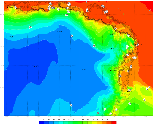
ECMWF 01 Febbraio 2018 00UTC Forecast T+36 VT: Venerdì 02 Febbraio 2018 12UTC Terra Vittoria - temperature at 2 m (°C)
