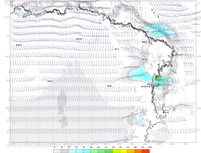
ECMWF 01 Febbraio 2018 00UTC Forecast T+30 VT: Venerdì 02 Febbraio 2018 06UTC Terra Vittoria - Wind at 10 m (kts)
