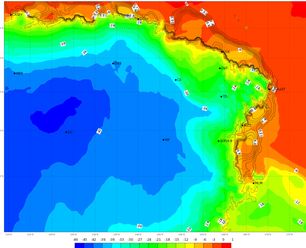
ECMWF 01 Febbraio 2018 00UTC Forecast T+42 VT: Venerdì 02 Febbraio 2018 18UTC Terra Vittoria - Temperature at 2 m (°C)
