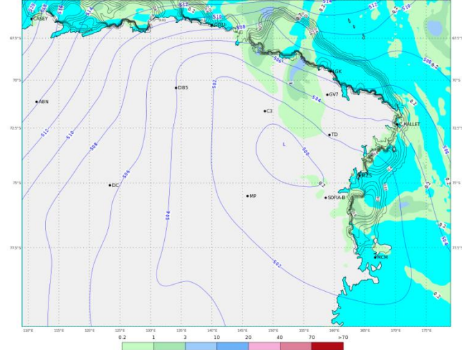
ECMWF 01 Febbraio 2018 00UTC Forecast T+42 VT: Venerdì 02 Febbraio 2018 18UTC Terra Vittoria - Geopotential at 500 hPa + 6h accumulated precipitation (mm)
