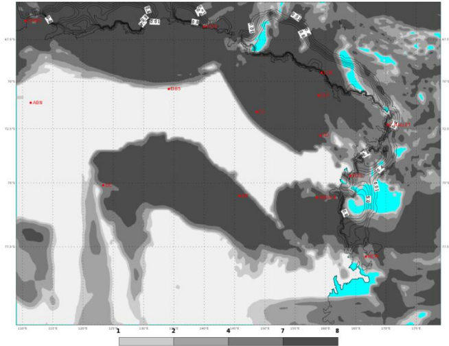
ECMWF 01 Febbraio 2018 00UTC Forecast T+18 VT: Giovedì 01 Febbraio 2018 18UTC Terra Vittoria - Total cloud cover (oct)
