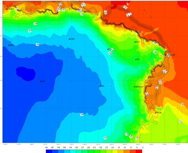
ECMWF 01 Febbraio 2018 00UTC Forecast T+48 VT: Sabato 03 Febbraio 2018 00UTC Terra Vittoria - Temperature at 2 m (°C)
