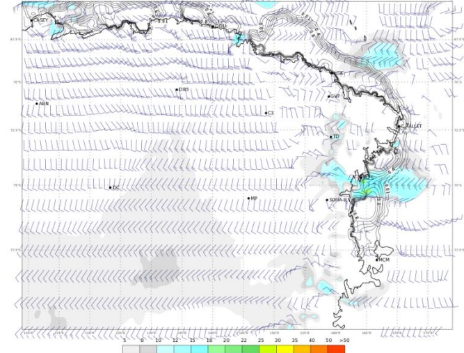
ECMWF 01 Febbraio 2018 00UTC Forecast T+42 VT: Venerdì 02 Febbraio 2018 18UTC Terra Vittoria - Wind at 10 m (kts)
