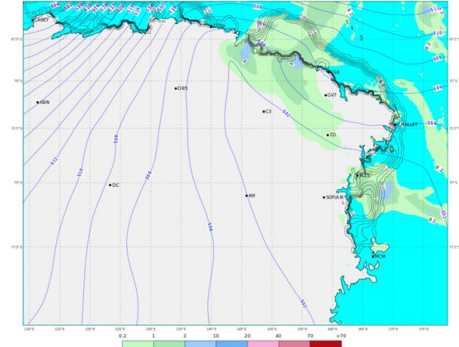
ECMWF 01 Febbraio 2018 00UTC Forecast T+54 VT: Sabato 03 Febbraio 2018 06UTC Terra Vittoria - Geopotential at 500 hPa + 6h accumulated precipitation (mm)
