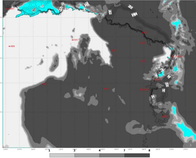
ECMWF 01 Febbraio 2018 00UTC Forecast T+48 VT: Sabato 03 Febbraio 2018 00UTC Terra Vittoria - Total cloud cover (oct)
