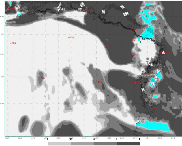
ECMWF 01 Febbraio 2018 00UTC Forecast T+36 VT: Venerdì 02 Febbraio 2018 12UTC Terra Vittoria - Total cloud cover (oct)
