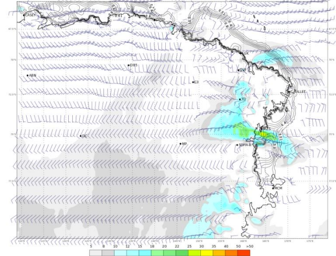
ECMWF 01 Febbraio 2018 00UTC Forecast T+18 VT: Giovedì 01 Febbraio 2018 18UTC Terra Vittoria - Wind at 10 m (kts)
