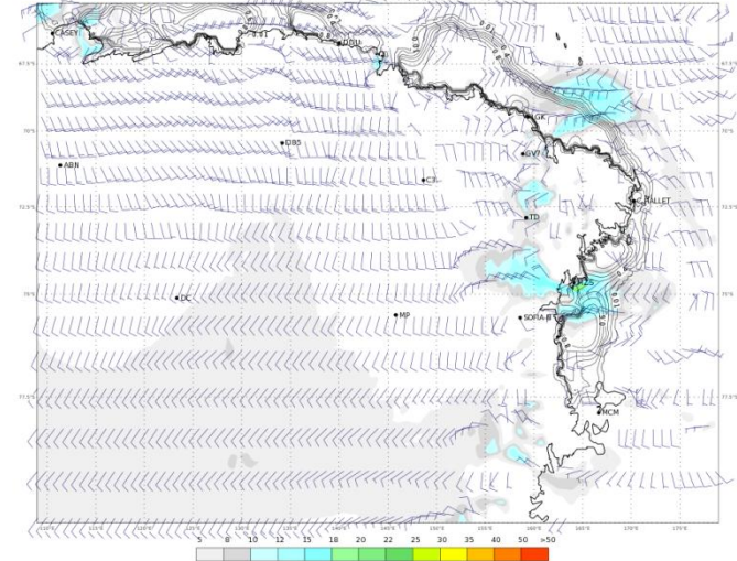
ECMWF 01 Febbraio 2018 00UTC Forecast T+36 VT: Venerdì 02 Febbraio 2018 12UTC Terra Vittoria - Wind at 10 m (kts)
