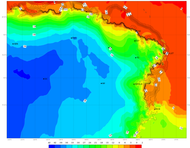
ECMWF 01 Febbraio 2018 00UTC Forecast T+24 VT: Venerdì 02 Febbraio 2018 00UTC Terra Vittoria - Temperature at 2 m (°C)
