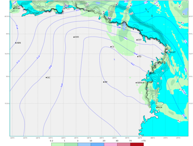
ECMWF 01 Febbraio 2018 00UTC Forecast T+36 VT: Venerdì 02 Febbraio 2018 12UTC Terra Vittoria - Geopotential at 500 hPa + 6h accumulated precipitation (mm)
