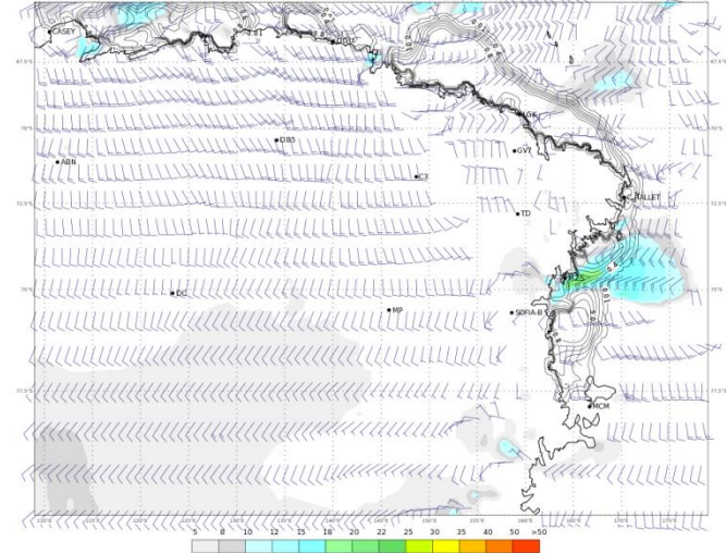
ECMWF 01 Febbraio 2018 00UTC Forecast T+48 VT: Sabato 03 Febbraio 2018 00UTC Terra Vittoria - Wind at 10 m (kts)
