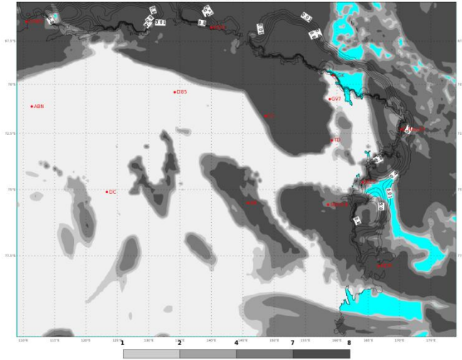
ECMWF 01 Febbraio 2018 00UTC Forecast T+30 VT: Venerdì 02 Febbraio 2018 06UTC Terra Vittoria - Total cloud cover (oct)
