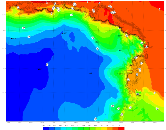
ECMWF 01 Febbraio 2018 00UTC Forecast T+30 VT: Venerdì 02 Febbraio 2018 06UTC Terra Vittoria - Temperature at 2 m (°C)
