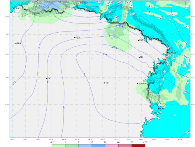
ECMWF 01 Febbraio 2018 00UTC Forecast T+18 VT: Giovedì 01 Febbraio 2018 18UTC Terra Vittoria - Geopotential at 500 hPa + 6h accumulated precipitation (mm)
