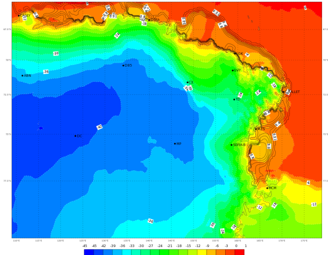
ECMWF 01 Febbraio 2018 00UTC Forecast T+18 VT: Giovedì 01 Febbraio 2018 18UTC Terra Vittoria - Temperature at 2 m (°C)
