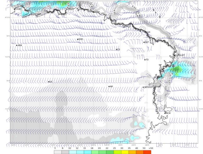
ECMWF 01 Febbraio 2018 00UTC Forecast T+54 VT: Sabato 03 Febbraio 2018 06UTC Terra Vittoria - Wind at 10 m (kts)
