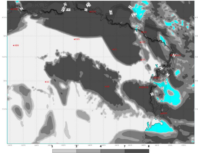
ECMWF 01 Febbraio 2018 00UTC Forecast T+24 VT: Venerdì 02 Febbraio 2018 00UTC Terra Vittoria - Total cloud cover (oct)
