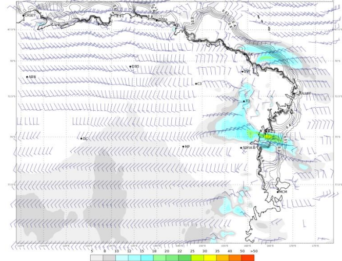
ECMWF 01 Febbraio 2018 00UTC Forecast T+24 VT: Venerdì 02 Febbraio 2018 00UTC Terra Vittoria - Wind at 10 m (kts)
