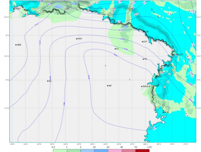
ECMWF 01 Febbraio 2018 00UTC Forecast T+24 VT: Venerdì 02 Febbraio 2018 00UTC Terra Vittoria - Geopotential at 500 hPa + 6h accumulated precipitation (mm)
