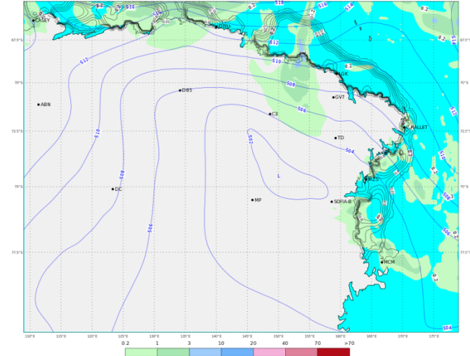
ECMWF 01 Febbraio 2018 00UTC Forecast T+30 VT: Venerdì 02 Febbraio 2018 06UTC Terra Vittoria - Geopotential at 500 hPa + 6h accumulated precipitation (mm)
