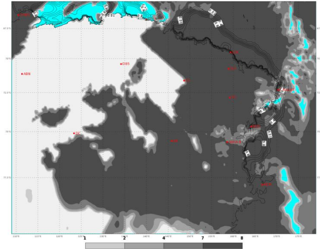
ECMWF 01 Febbraio 2018 00UTC Forecast T+54 VT: Sabato 03 Febbraio 2018 06UTC Terra Vittoria - Total cloud cover (oct)
