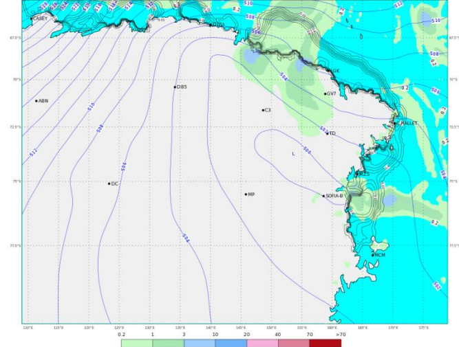
ECMWF 01 Febbraio 2018 00UTC Forecast T+48 VT: Sabato 03 Febbraio 2018 00UTC Terra Vittoria - Geopotential at 500 hPa + 6h accumulated precipitation (mm)
