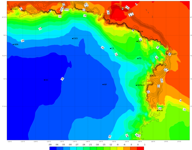
ECMWF 01 Febbraio 2018 00UTC Forecast T+54 VT: Sabato 03 Febbraio 2018 06UTC Terra Vittoria - Temperature at 2 m (°C)
