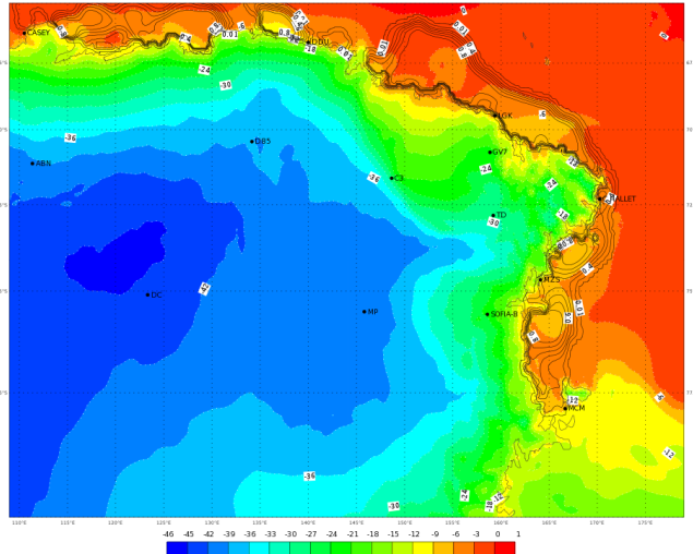
ECMWF 02 Febbraio 2018 00UTC Forecast T+18 VT: Venerdì 02 Febbraio 2018 18UTC Terra Vittoria - temperature at 2 m (°C)
