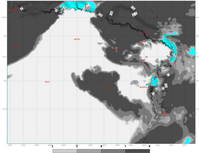
ECMWF 02 Febbraio 2018 00UTC Forecast T+42 VT: Sabato 03 Febbraio 2018 18UTC Terra Vittoria - Total cloud cover (oct)
