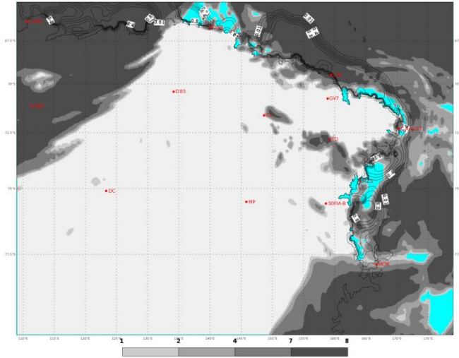
ECMWF 02 Febbraio 2018 00UTC Forecast T+48 VT: Domenica 04 Febbraio 2018 00UTC Terra Vittoria - Total cloud cover (oct)
