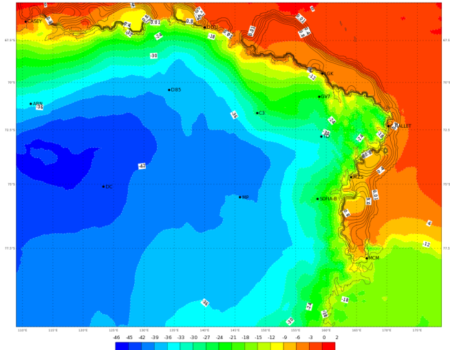
ECMWF 02 Febbraio 2018 00UTC Forecast T+42 VT: Sabato 03 Febbraio 2018 18UTC Terra Vittoria - Temperature at 2 m (°C)
