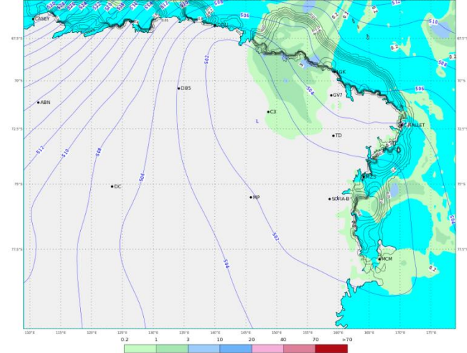
ECMWF 02 Febbraio 2018 00UTC Forecast T+24 VT: Sabato 03 Febbraio 2018 00UTC Terra Vittoria - Geopotential at 500 hPa + 6h accumulated precipitation (mm)
