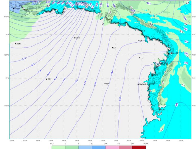
ECMWF 02 Febbraio 2018 00UTC Forecast T+48 VT: Domenica 04 Febbraio 2018 00UTC Terra Vittoria - Geopotential at 500 hPa + 6h accumulated precipitation (mm)
