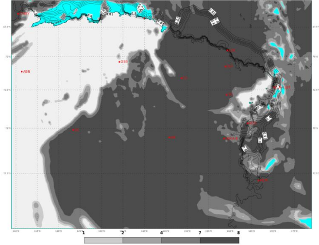
ECMWF 02 Febbraio 2018 00UTC Forecast T+24 VT: Sabato 03 Febbraio 2018 00UTC Terra Vittoria - Total cloud cover (oct)
