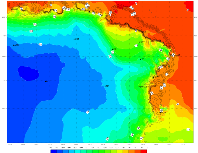
ECMWF 02 Febbraio 2018 00UTC Forecast T+24 VT: Sabato 03 Febbraio 2018 00UTC Terra Vittoria - Temperature at 2 m (°C)
