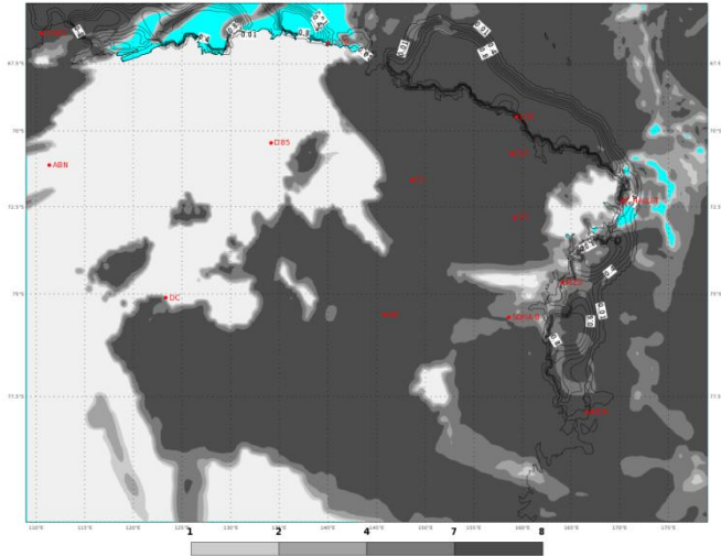
ECMWF 02 Febbraio 2018 00UTC Forecast T+30 VT: Sabato 03 Febbraio 2018 06UTC Terra Vittoria - Total cloud cover (oct)
