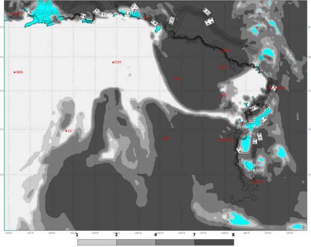
ECMWF 02 Febbraio 2018 00UTC Forecast T+18 VT: Venerdì 02 Febbraio 2018 18UTC Terra Vittoria - Total cloud cover (oct)
