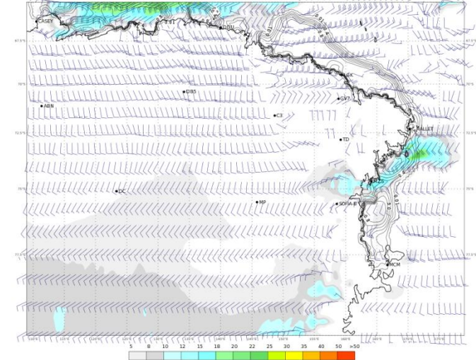
ECMWF 02 Febbraio 2018 00UTC Forecast T+30 VT: Sabato 03 Febbraio 2018 06UTC Terra Vittoria - Wind at 10 m (kts)
