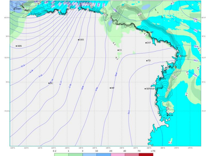
ECMWF 02 Febbraio 2018 00UTC Forecast T+42 VT: Sabato 03 Febbraio 2018 18UTC Terra Vittoria - Geopotential at 500 hPa + 6h accumulated precipitation (mm)
