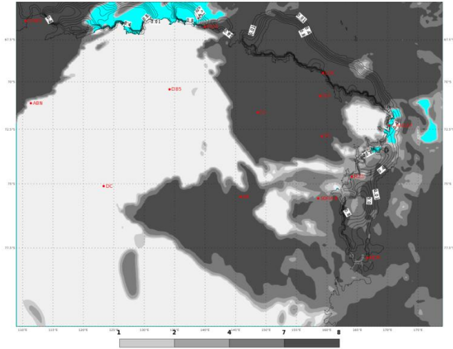
ECMWF 02 Febbraio 2018 00UTC Forecast T+36 VT: Sabato 03 Febbraio 2018 12UTC Terra Vittoria - Total cloud cover (oct)
