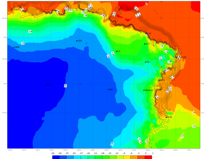
ECMWF 02 Febbraio 2018 00UTC Forecast T+30 VT: Sabato 03 Febbraio 2018 06UTC Terra Vittoria - Temperature at 2 m (°C)
