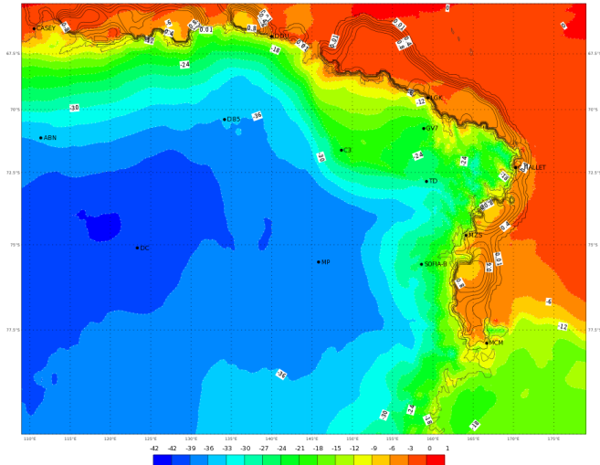
ECMWF 02 Febbraio 2018 00UTC Forecast T+36 VT: Sabato 03 Febbraio 2018 12UTC Terra Vittoria - temperature at 2 m (°C)
