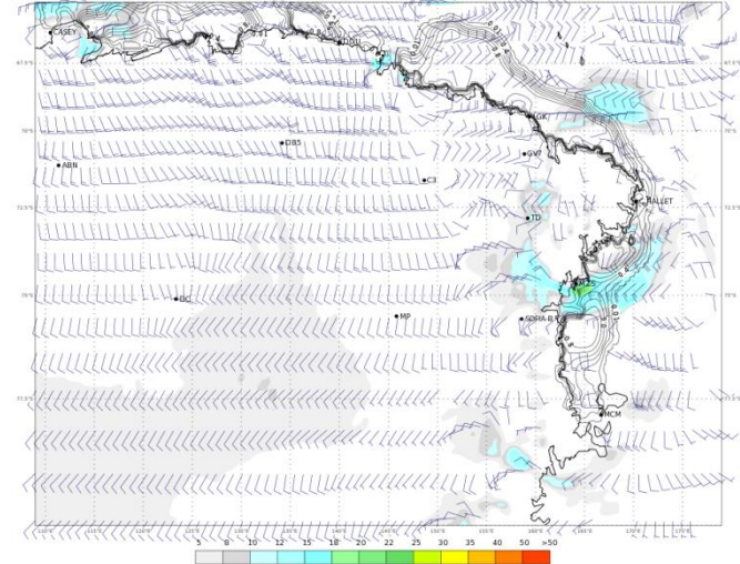
ECMWF 02 Febbraio 2018 00UTC Forecast T+18 VT: Venerdì 02 Febbraio 2018 18UTC Terra Vittoria - Wind at 10 m (kts)
