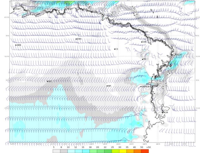
ECMWF 02 Febbraio 2018 00UTC Forecast T+36 VT: Sabato 03 Febbraio 2018 12UTC Terra Vittoria - Wind at 10 m (kts)
