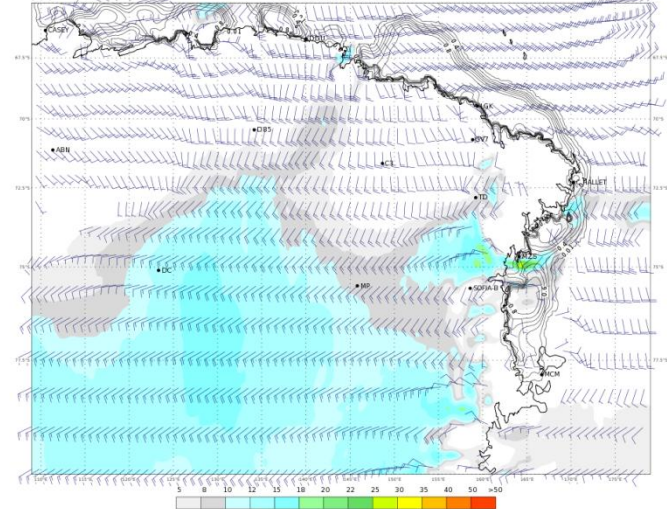
ECMWF 02 Febbraio 2018 00UTC Forecast T+48 VT: Domenica 04 Febbraio 2018 00UTC Terra Vittoria - Wind at 10 m (kts)
