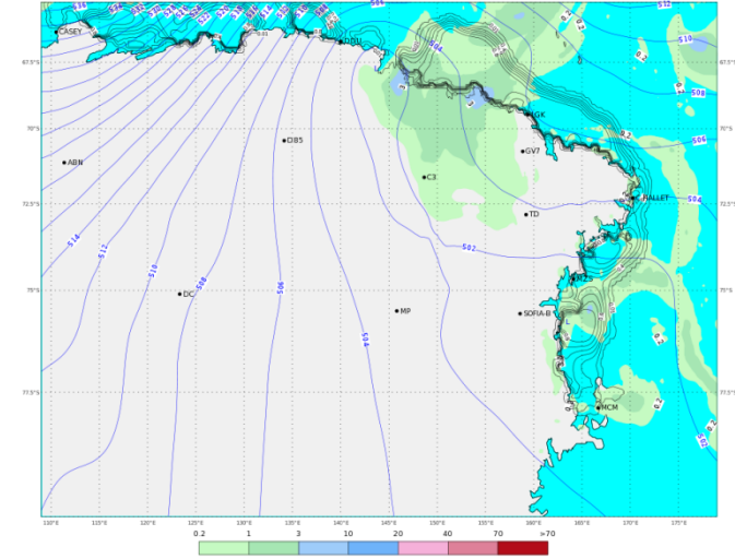
ECMWF 02 Febbraio 2018 00UTC Forecast T+30 VT: Sabato 03 Febbraio 2018 06UTC Terra Vittoria - Geopotential at 500 hPa + 6h accumulated precipitation (mm)
