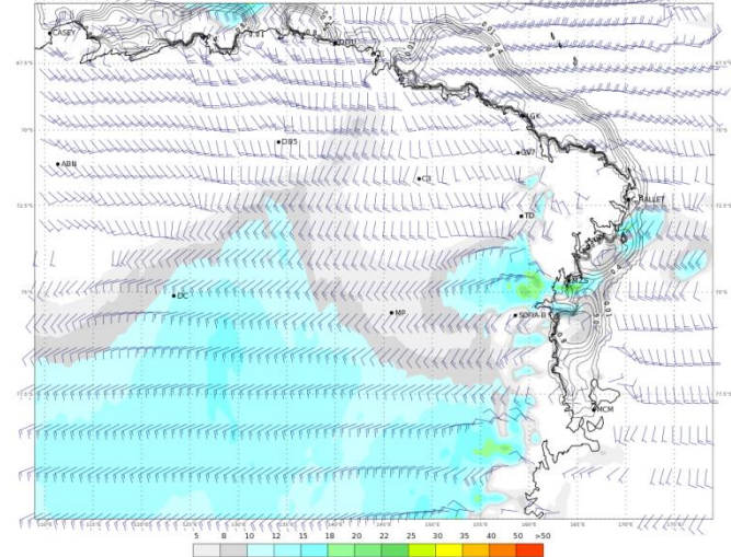
ECMWF 02 Febbraio 2018 00UTC Forecast T+42 VT: Sabato 03 Febbraio 2018 18UTC Terra Vittoria - Wind at 10 m (kts)
