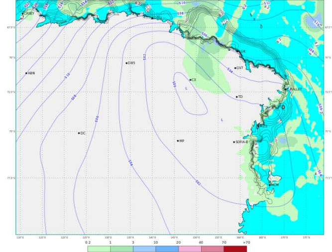
ECMWF 02 Febbraio 2018 00UTC Forecast T+18 VT: Venerdì 02 Febbraio 2018 18UTC Terra Vittoria - Geopotential at 500 hPa + 6h accumulated precipitation (mm)
