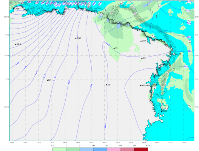
ECMWF 02 Febbraio 2018 00UTC Forecast T+36 VT: Sabato 03 Febbraio 2018 12UTC Terra Vittoria - Geopotential at 500 hPa + 6h accumulated precipitation (mm)
