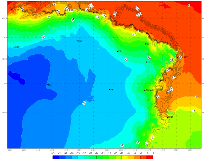
ECMWF 02 Febbraio 2018 00UTC Forecast T+48 VT: Domenica 04 Febbraio 2018 00UTC Terra Vittoria - Temperature at 2 m (°C)
