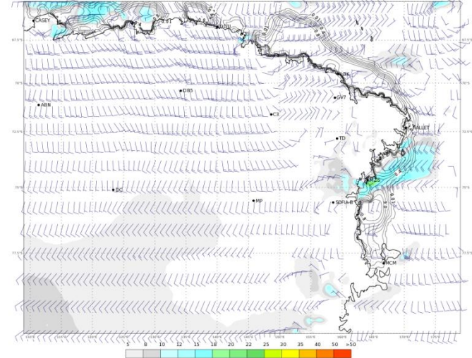
ECMWF 02 Febbraio 2018 00UTC Forecast T+24 VT: Sabato 03 Febbraio 2018 00UTC Terra Vittoria - Wind at 10 m (kts)
