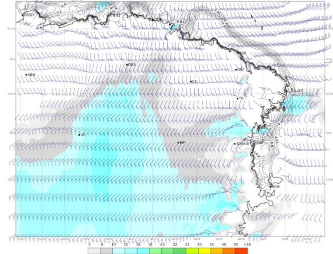
ECMWF 03 Febbraio 2018 00UTC Forecast T+30 VT: Domenica 04 Febbraio 2018 06UTC Terra Vittoria - Wind at 10 m (kts)
