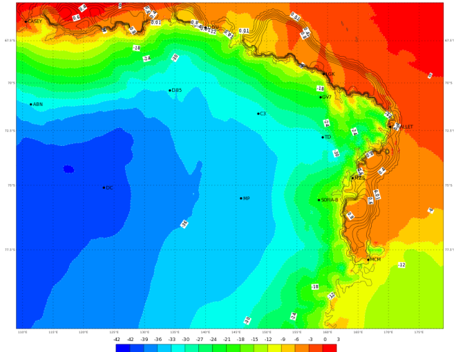
ECMWF 03 Febbraio 2018 00UTC Forecast T+48 VT: Lunedì 05 Febbraio 2018 00UTC Terra Vittoria - Temperature at 2 m (°C)
