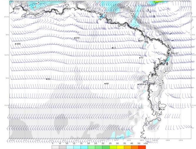
ECMWF 03 Febbraio 2018 00UTC Forecast T+54 VT: Lunedì 05 Febbraio 2018 06UTC Terra Vittoria - Wind at 10 m (kts)
