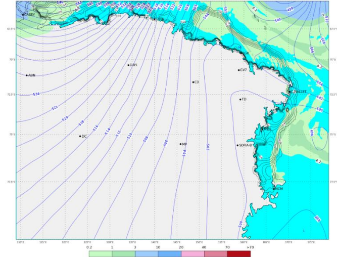
ECMWF 03 Febbraio 2018 00UTC Forecast T+30 VT: Domenica 04 Febbraio 2018 06UTC Terra Vittoria - Geopotential at 500 hPa + 6h accumulated precipitation (mm)
