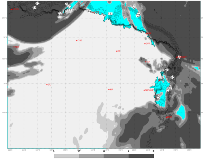
ECMWF 03 Febbraio 2018 00UTC Forecast T+36 VT: Domenica 04 Febbraio 2018 12UTC Terra Vittoria - Total cloud cover (oct)
