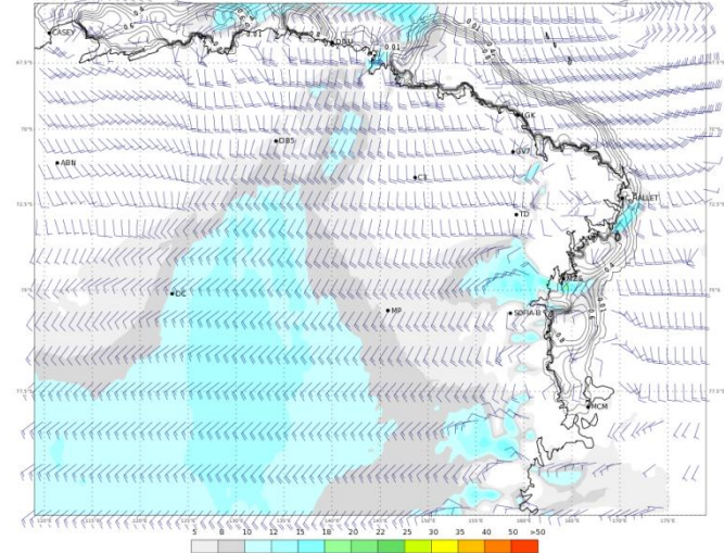
ECMWF 03 Febbraio 2018 00UTC Forecast T+36 VT: Domenica 04 Febbraio 2018 12UTC Terra Vittoria - Wind at 10 m (kts)
