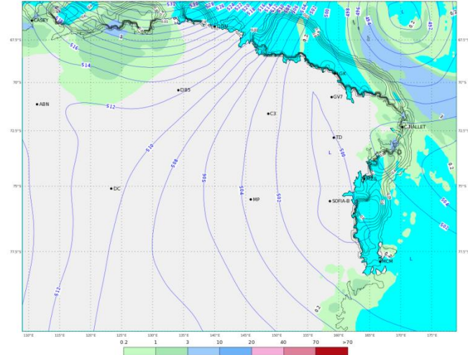
ECMWF 03 Febbraio 2018 00UTC Forecast T+54 VT: Lunedì 05 Febbraio 2018 06UTC Terra Vittoria - Geopotential at 500 hPa + 6h accumulated precipitation (mm)
