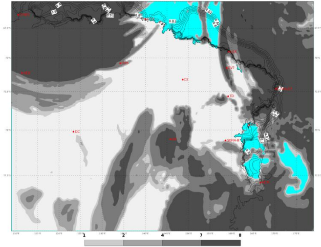
ECMWF 03 Febbraio 2018 00UTC Forecast T+48 VT: Lunedì 05 Febbraio 00UTC Terra Vittoria - Total cloud cover (oct)
