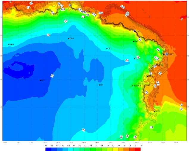
ECMWF 03 Febbraio 2018 00UTC Forecast T+18 VT: Sabato 03 Febbraio 2018 18UTC Terra Vittoria - temperature at 2 m (°C)
