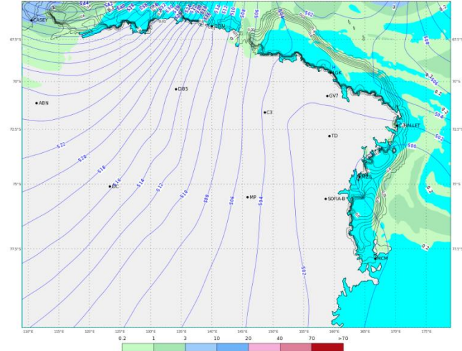
ECMWF 03 Febbraio 2018 00UTC Forecast T+24 VT: Domenica 04 Febbraio 2018 00UTC Terra Vittoria - Geopotential at 500 hPa + 6h accumulated precipitation (mm)
