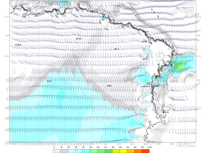
ECMWF 03 Febbraio 2018 00UTC Forecast T+18 VT: Sabato 03 Febbraio 2018 18UTC Terra Vittoria - Wind at 10 m (kts)
