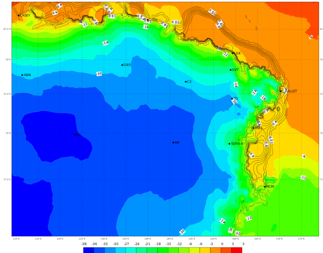
ECMWF 03 Febbraio 2018 00UTC Forecast T+30 VT: Domenica 04 Febbraio 2018 06UTC Terra Vittoria - Temperature at 2 m (°C)
