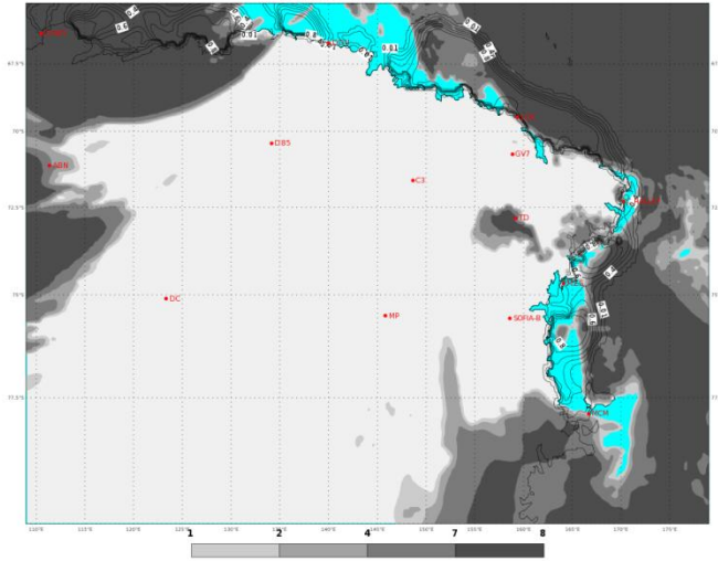
ECMWF 03 Febbraio 2018 00UTC Forecast T+30 VT: Domenica 04 Febbraio 2018 06UTC Terra Vittoria - Total cloud cover (oct)
