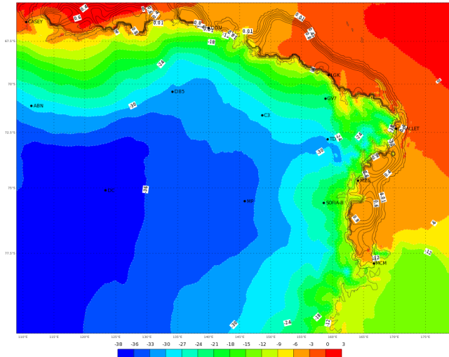
ECMWF 03 Febbraio 2018 00UTC Forecast T+54 VT: Lunedì 05 Febbraio 2018 06UTC Terra Vittoria - temperature at 2 m (°C)
