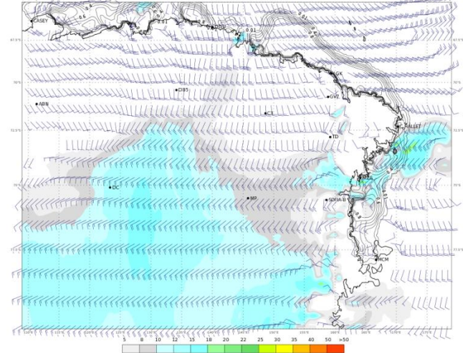
ECMWF 03 Febbraio 2018 00UTC Forecast T+24 VT: Domenica 04 Febbraio 2018 00UTC Terra Vittoria - Wind at 10 m (kts)
