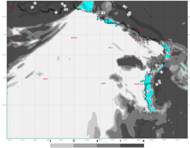
ECMWF 03 Febbraio 2018 00UTC Forecast T+24 VT: Domenica 04 Febbraio 2018 00UTC Terra Vittoria - Total cloud cover (oct)
