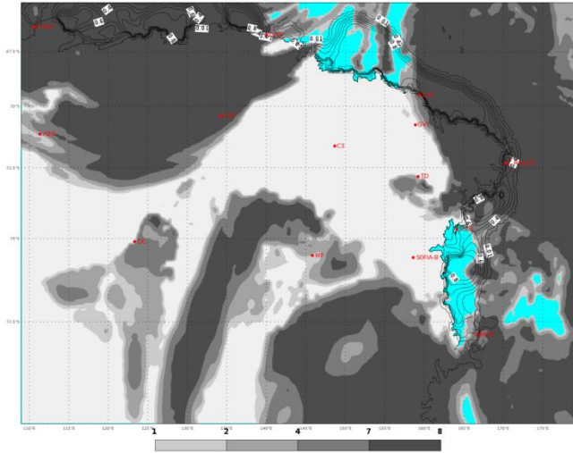
ECMWF 03 Febbraio 2018 00UTC Forecast T+54 VT: Lunedì 05 Febbraio 2018 06UTC Terra Vittoria - Total cloud cover (oct)
