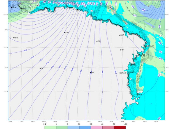
ECMWF 03 Febbraio 2018 00UTC Forecast T+36 VT: Domenica 04 Febbraio 2018 12UTC Terra Vittoria - Geopotential at 500 hPa + 6h accumulated precipitation (mm)
