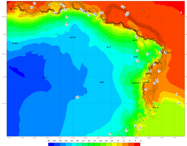
ECMWF 03 Febbraio 2018 00UTC Forecast T+24 VT: Domenica 04 Febbraio 2018 00UTC Terra Vittoria - Temperature at 2 m (°C)
