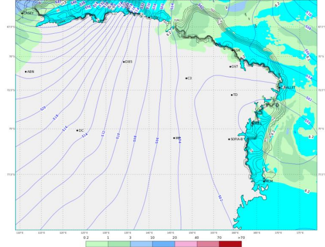
ECMWF 03 Febbraio 2018 00UTC Forecast T+18 VT: Sabato 03 Febbraio 2018 18UTC Terra Vittoria - Geopotential at 500 hPa + 6h accumulated precipitation (mm)
