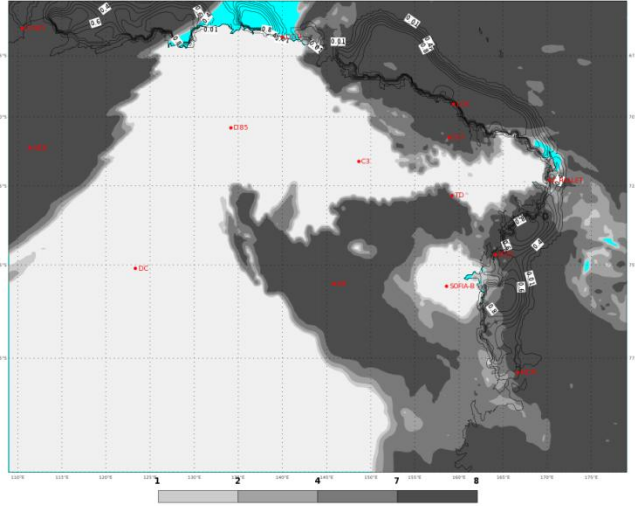
ECMWF 03 Febbraio 2018 00UTC Forecast T+18 VT: Sabato 03 Febbraio 2018 18UTC Terra Vittoria - Total cloud cover (oct)
