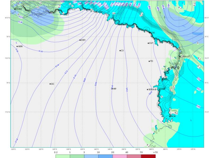
ECMWF 03 Febbraio 2018 00UTC Forecast T+48 VT: Lunedì 05 Febbraio 2018 00UTC Terra Vittoria - Geopotential at 500 hPa + 6h accumulated precipitation (mm)
