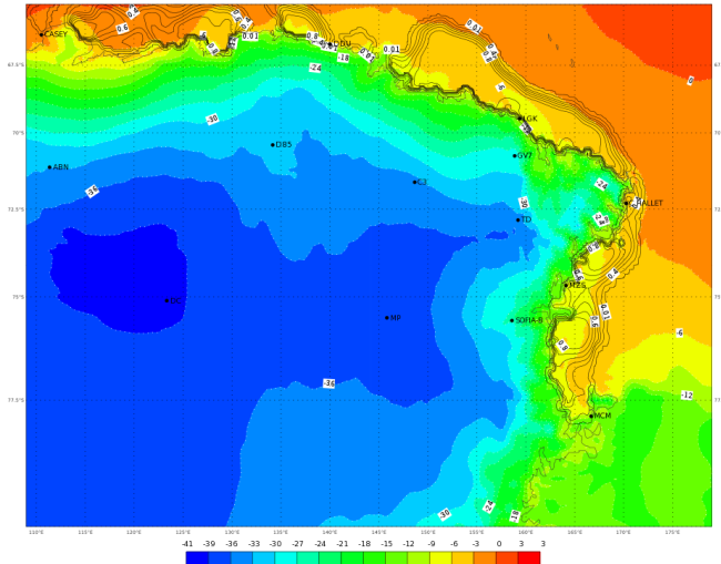
ECMWF 03 Febbraio 2018 00UTC Forecast T+36 VT: Domenica 04 Febbraio 2018 12UTC Terra Vittoria - Temperature at 2 m (°C)
