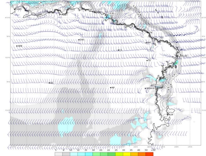
ECMWF 03 Febbraio 2018 00UTC Forecast T+48 VT: Lunedì 05 Febbraio 2018 00UTC Terra Vittoria - Wind at 10 m (kts)
