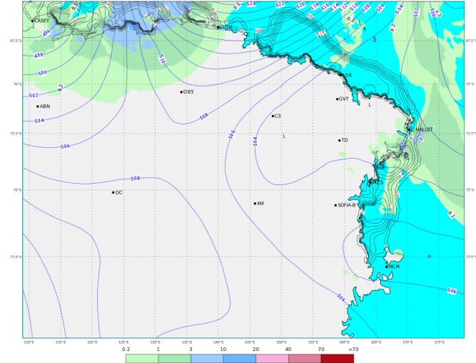
ECMWF 04 Febbraio 2018 00UTC Forecast T+54 VT: Martedì 06 Febbraio 2018 06UTC Terra Vittoria - Geopotential at 500 hPa + 6h accumulated precipitation (mm)
