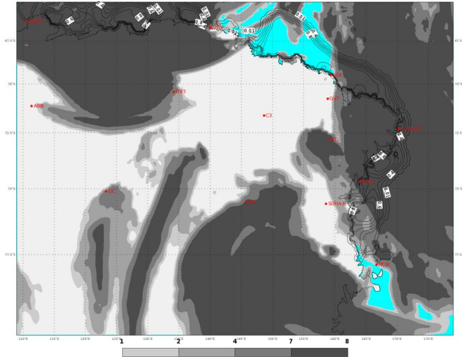
ECMWF 04 Febbraio 2018 00UTC Forecast T+36 VT: Lunedì 05 Febbraio 2018 12UTC Terra Vittoria - total cloud cover (oct)
