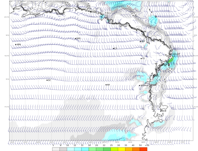
ECMWF 04 Febbraio 2018 00UTC Forecast T+42 VT: Lunedì 05 Febbraio 2018 18UTC Terra Vittoria - Wind at 10 m (kts)
