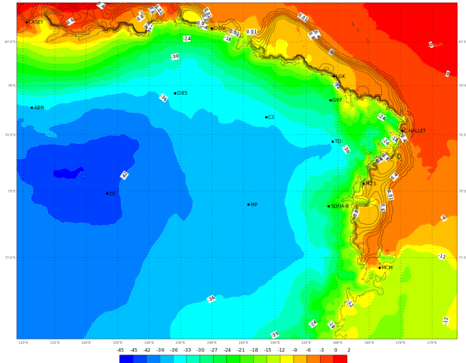
ECMWF 04 Febbraio 2018 00UTC Forecast T+18 VT: Domenica 04 Febbraio 2018 18UTC Terra Vittoria - temperature at 2 m (°C)
