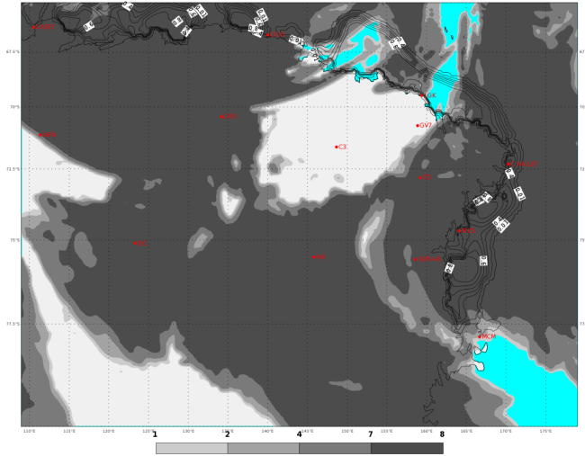
ECMWF 04 Febbraio 2018 00UTC Forecast T+48 VT: Martedì 06 Febbraio 2018 00UTC Terra Vittoria - Total cloud cover (oct)
