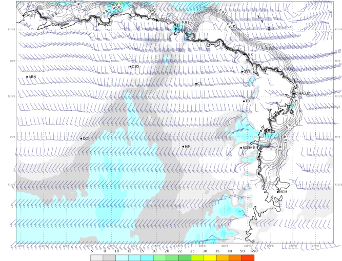
ECMWF 04 Febbraio 2018 00UTC Forecast T+18 VT: Domenica 04 Febbraio 2018 18UTC Terra Vittoria - Wind at 10 m (kts)
