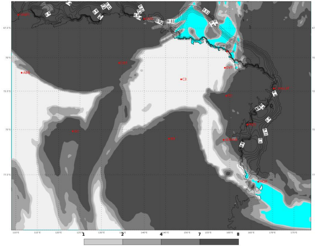
ECMWF 04 Febbraio 2018 00UTC Forecast T+42 VT: Lunedì 05 Febbraio 2018 18UTC Terra Vittoria - total cloud cover (oct)
