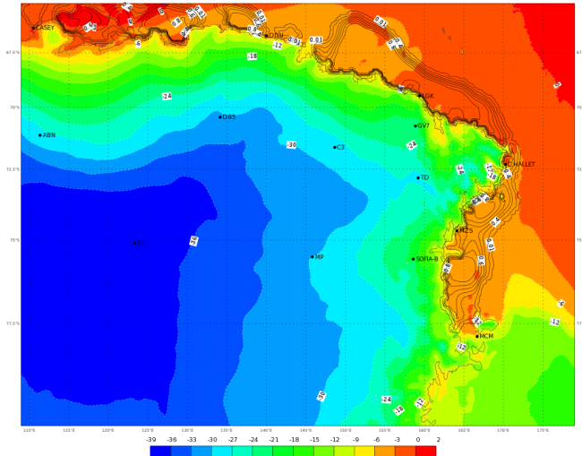
ECMWF 04 Febbraio 2018 00UTC Forecast T+54 VT: Martedì 06 Febbraio 2018 06UTC Terra Vittoria - Temperature at 2 m (°C)
