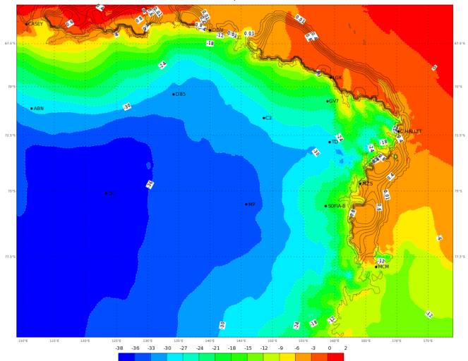
ECMWF 04 Febbraio 2018 00UTC Forecast T+30 VT: Lunedì 05 Febbraio 2018 06UTC Terra Vittoria - temperature at 2 m (°C)
