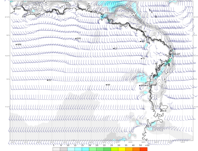
ECMWF 04 Febbraio 2018 00UTC Forecast T+36 VT: Lunedì 05 Febbraio 2018 12UTC Terra Vittoria - Wind at 10 m (kts)
