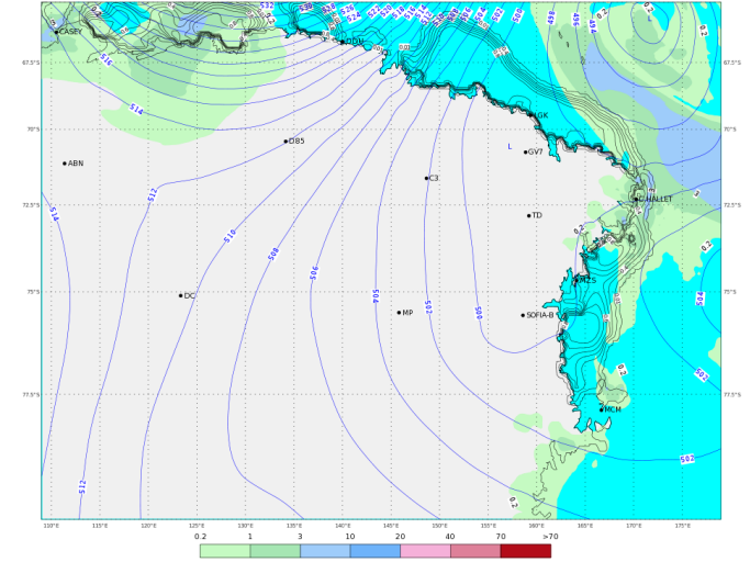
ECMWF 04 Febbraio 2018 00UTC Forecast T+30 VT: Lunedì 05 Febbraio 2018 06UTC Terra Vittoria - Geopotential at 500 hPa + 6h accumulated precipitation (mm)
