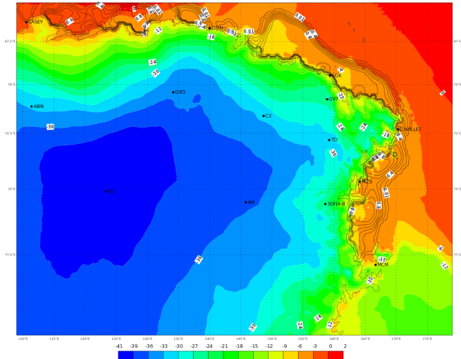
ECMWF 04 Febbraio 2018 00UTC Forecast T+36 VT: Lunedì 05 Febbraio 2018 12UTC Terra Vittoria - temperature at 2 m (°C)
