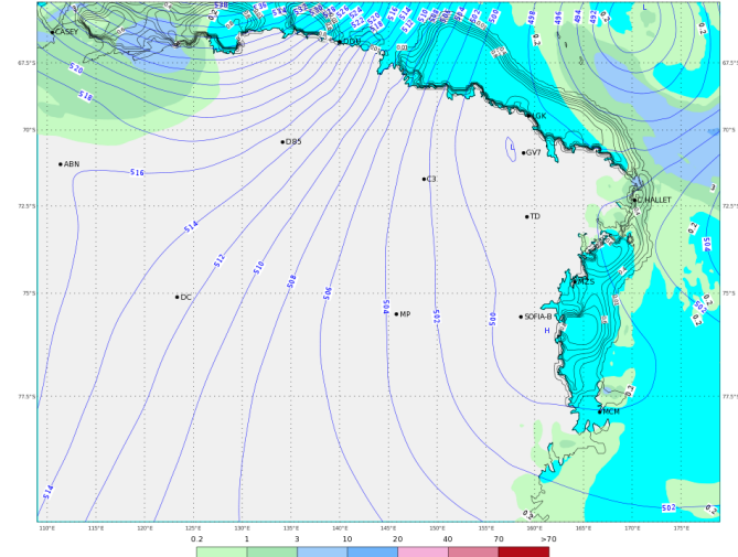
ECMWF 04 Febbraio 2018 00UTC Forecast T+24 VT: Lunedì 05 Febbraio 2018 00UTC Terra Vittoria - Geopotential at 500 hPa + 6h accumulated precipitation (mm)
