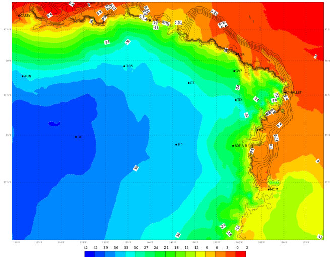
ECMWF 04 Febbraio 2018 00UTC Forecast T+24 VT: Lunedì 05 Febbraio 2018 00UTC Terra Vittoria - temperature at 2 m (°C)
