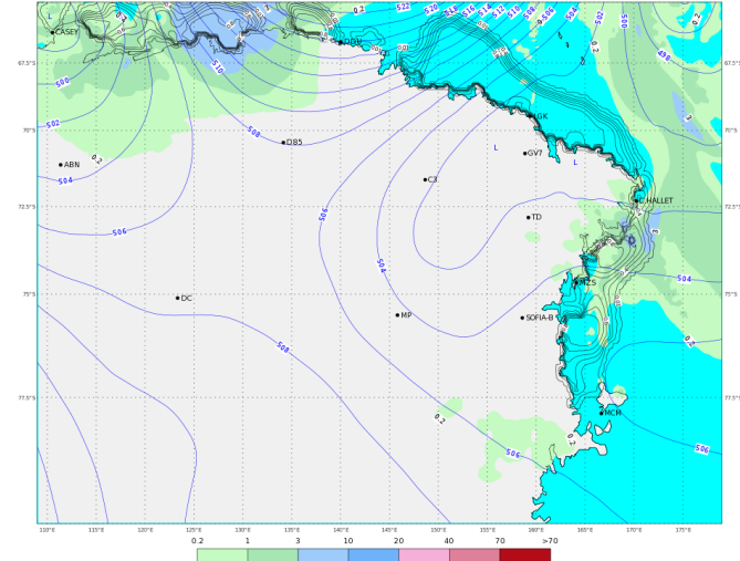
ECMWF 04 Febbraio 2018 00UTC Forecast T+48 VT: Martedì 06 Febbraio 2018 00UTC Terra Vittoria - Geopotential at 500 hPa + 6h accumulated precipitation (mm)
