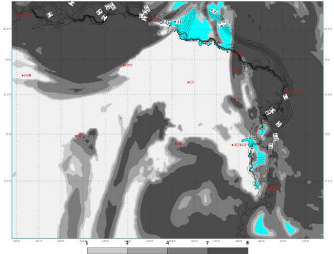
ECMWF 04 Febbraio 2018 00UTC Forecast T+30 VT: Lunedì 05 Febbraio 2018 06UTC Terra Vittoria - total cloud cover (oct)
