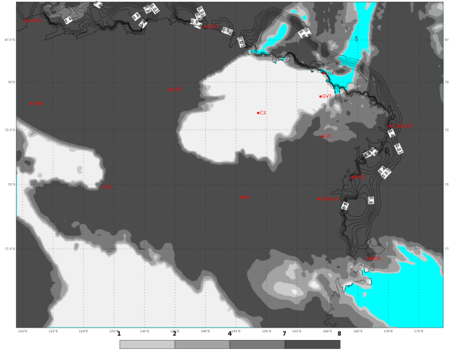
ECMWF 04 Febbraio 2018 00UTC Forecast T+54 VT: Martedì 06 Febbraio 2018 06UTC Terra Vittoria - Total cloud cover (oct)
