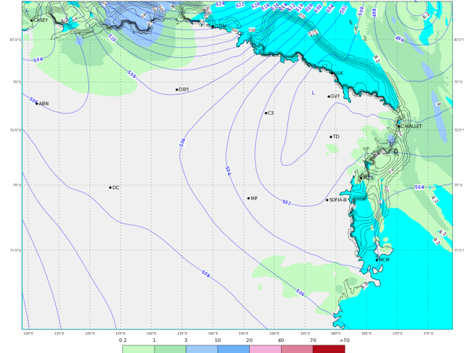
ECMWF 04 Febbraio 2018 00UTC Forecast T+42 VT: Lunedì 05 Febbraio 2018 18UTC Terra Vittoria - Geopotential at 500 hPa + 6h accumulated precipitation (mm)
