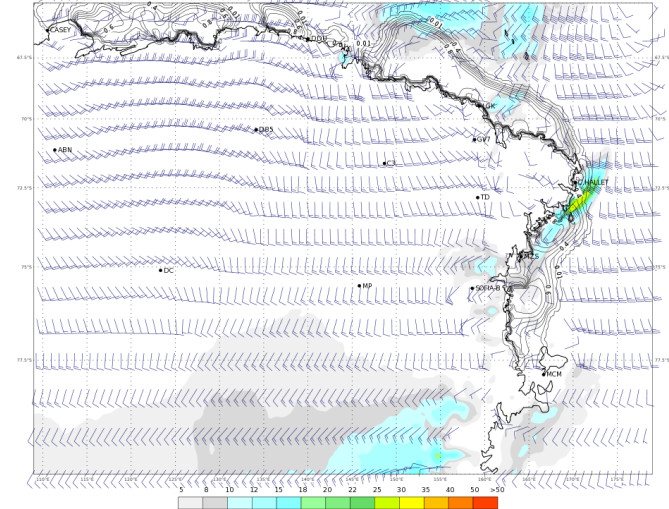
ECMWF 04 Febbraio 2018 00UTC Forecast T+48 VT: Martedì 06 Febbraio 2018 00UTC Terra Vittoria - Wind at 10 m (kts)
