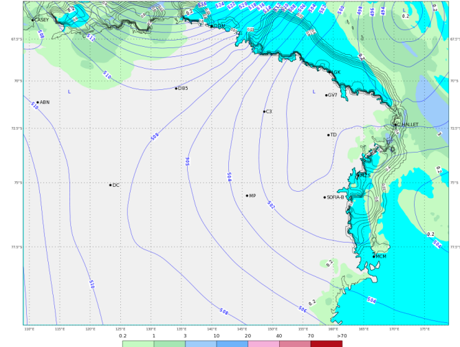
ECMWF 04 Febbraio 2018 00UTC Forecast T+36 VT: Lunedì 05 Febbraio 2018 12UTC Terra Vittoria - Geopotential at 500 hPa + 6h accumulated precipitation (mm)
