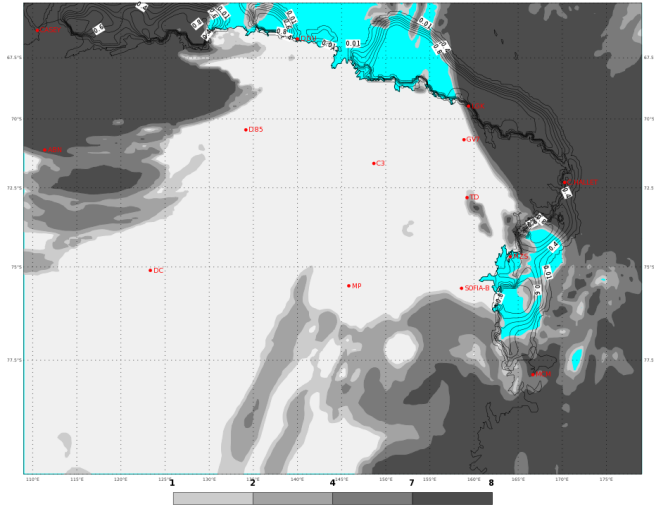
ECMWF 04 Febbraio 2018 00UTC Forecast T+18 VT: Domenica 04 Febbraio 2018 18UTC Terra Vittoria - Total cloud cover (oct)
