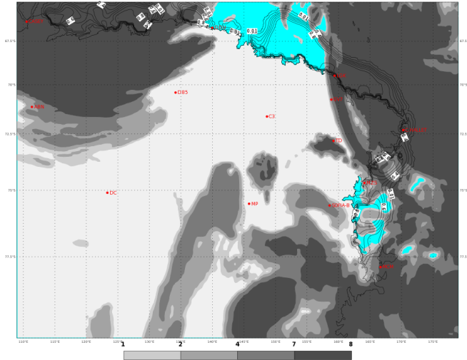
ECMWF 04 Febbraio 2018 00UTC Forecast T+24 VT: Lunedì 05 Febbraio 2018 00UTC Terra Vittoria - Total cloud cover (oct)
