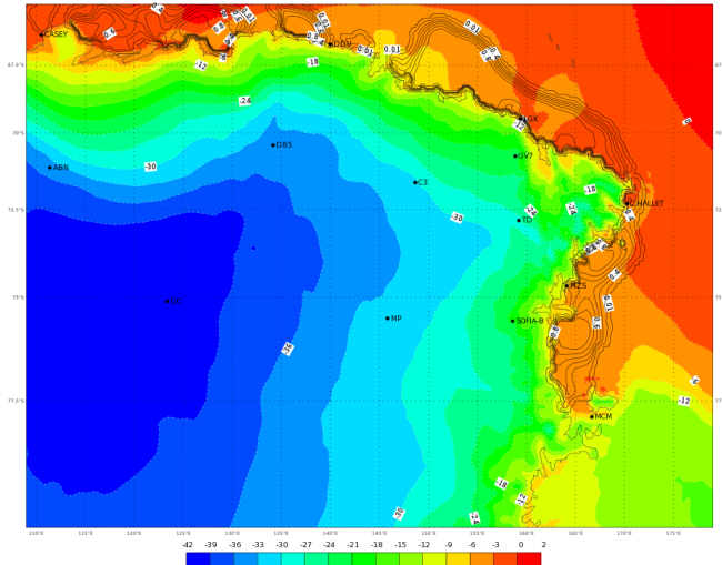
ECMWF 04 Febbraio 2018 00UTC Forecast T+48 VT: Martedì 06 Febbraio 2018 00UTC Terra Vittoria - Temperature at 2 m (°C)
