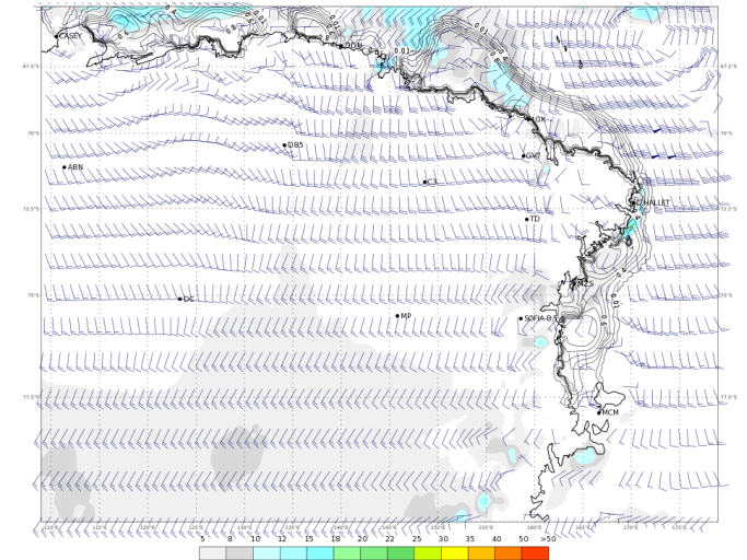
ECMWF 04 Febbraio 2018 00UTC Forecast T+30 VT: Lunedì 05 Febbraio 2018 06UTC Terra Vittoria - Wind at 10 m (kts)
