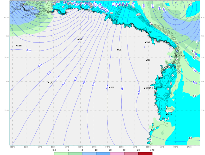
ECMWF 04 Febbraio 2018 00UTC Forecast T+18 VT: Domenica 04 Febbraio 2018 18UTC Terra Vittoria - Geopotential at 500 hPa + 6h accumulated precipitation (mm)
