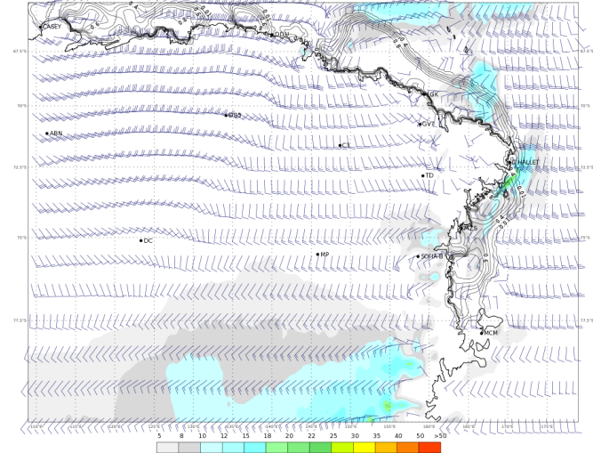
ECMWF 04 Febbraio 2018 00UTC Forecast T+54 VT: Martedì 06 Febbraio 2018 06UTC Terra Vittoria - Wind at 10 m (kts)
