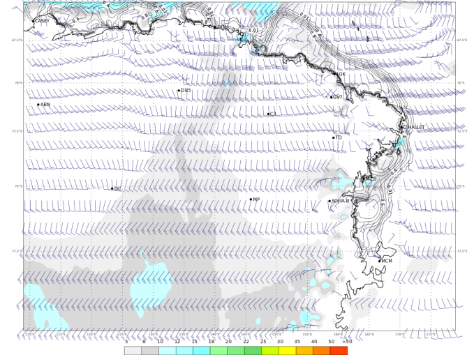
ECMWF 04 Febbraio 2018 00UTC Forecast T+24 VT: Lunedì 05 Febbraio 2018 00UTC Terra Vittoria - Wind at 10 m (kts)
