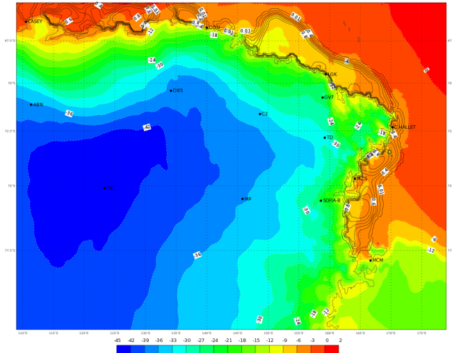
ECMWF 04 Febbraio 2018 00UTC Forecast T+42 VT: Lunedì 05 Febbraio 2018 18UTC Terra Vittoria - temperature at 2 m (°C)
