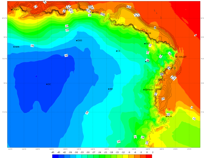
ECMWF 05 Febbraio 2018 00UTC Forecast T+18 VT: Lunedì 05 Febbraio 2018 18UTC Terra Vittoria - Temperature at 2 m (°C)
