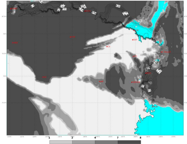
ECMWF 05 Febbraio 2018 00UTC Forecast T+42 VT: Martedì 06 Febbraio 2018 18UTC Terra Vittoria - Total cloud cover (oct)
