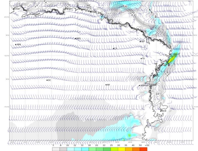
ECMWF 05 Febbraio 2018 00UTC Forecast T+24 VT: Martedì 06 Febbraio 2018 00UTC Terra Vittoria - Wind at 10 m (kts)
