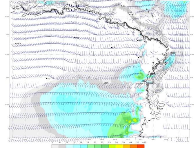
ECMWF 05 Febbraio 2018 00UTC Forecast T+42 VT: Martedì 06 Febbraio 2018 18UTC Terra Vittoria - Wind at 10 m (kts)
