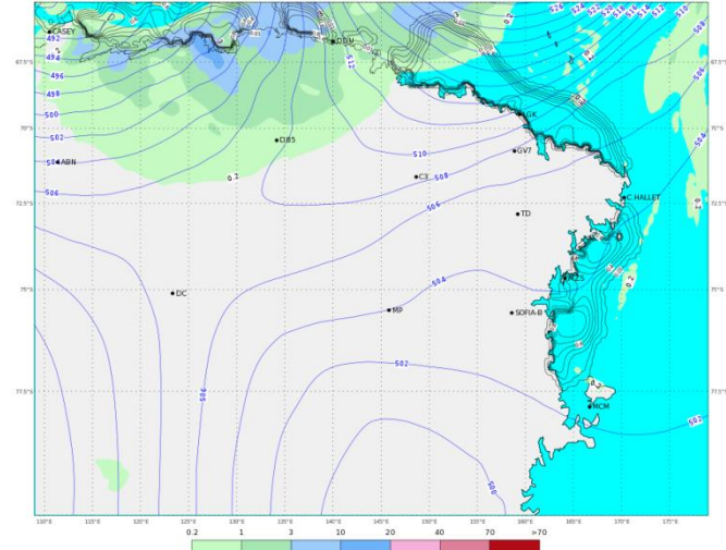
ECMWF 05 Febbraio 2018 00UTC Forecast T+48 VT: Mercoledì 07 Febbraio 2018 00UTC Terra Vittoria - Geopotential at 500 hPa + 6h accumulated precipitation (mm)
