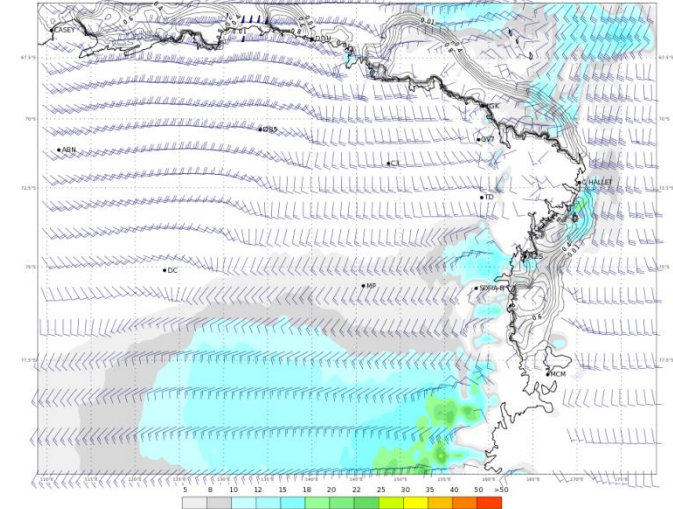
ECMWF 05 Febbraio 2018 00UTC Forecast T+36 VT: Martedì 06 Febbraio 2018 12UTC Terra Vittoria - Wind at 10 m (kts)
