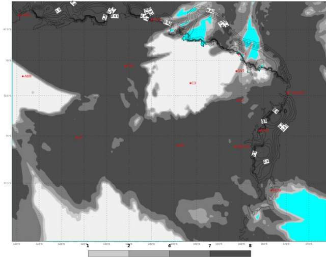
ECMWF 05 Febbraio 2018 00UTC Forecast T+24 VT: Martedì 06 Febbraio 2018 00UTC Terra Vittoria - Total cloud cover (oct)
