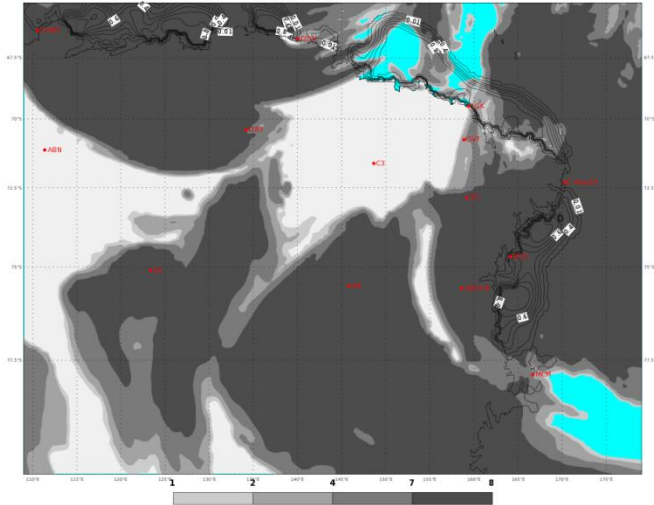
ECMWF 05 Febbraio 2018 00UTC Forecast T+18 VT: Lunedì 05 Febbraio 2018 18UTC Terra Vittoria - Total cloud cover (oct)
