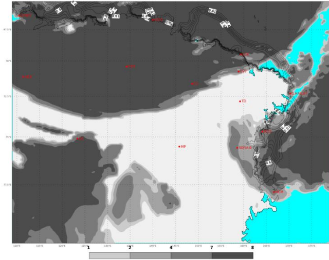
ECMWF 05 Febbraio 2018 00UTC Forecast T+54 VT: Mercoledì 07 Febbraio 2018 06UTC Terra Vittoria - Total cloud cover (oct)
