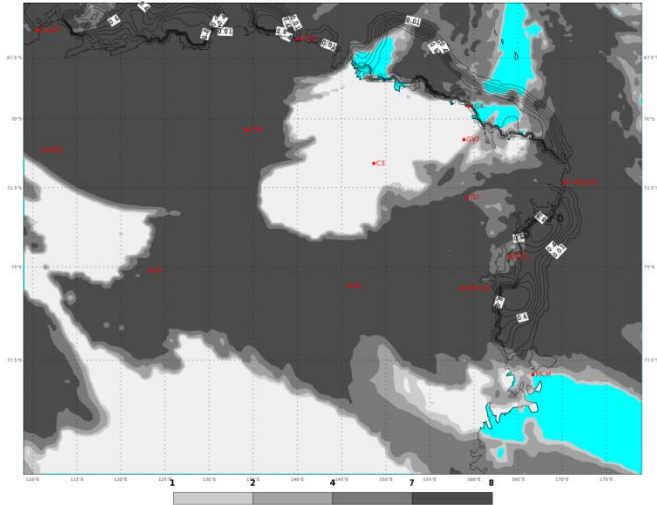
ECMWF 05 Febbraio 2018 00UTC Forecast T+30 VT: Martedì 06 Febbraio 2018 06UTC Terra Vittoria - Total cloud cover (oct)
