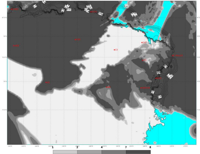
ECMWF 05 Febbraio 2018 00UTC Forecast T+36 VT: Martedì 06 Febbraio 2018 12UTC Terra Vittoria - Total cloud cover (oct)
