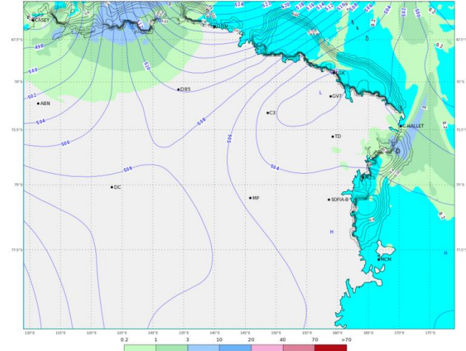
ECMWF 05 Febbraio 2018 00UTC Forecast T+30 VT: Martedì 06 Febbraio 2018 06UTC Terra Vittoria - Geopotential at 500 hPa + 6h accumulated precipitation (mm)
