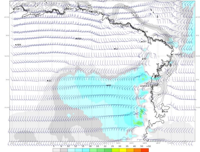
ECMWF 05 Febbraio 2018 00UTC Forecast T+54 VT: Mercoledì 07 Febbraio 2018 06UTC Terra Vittoria - Wind at 10 m (kts)
