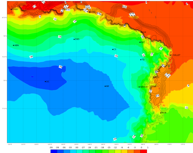
ECMWF 05 Febbraio 2018 00UTC Forecast T+54 VT: Mercoledì 07 Febbraio 2018 06UTC Terra Vittoria - Temperature at 2 m (°C)
