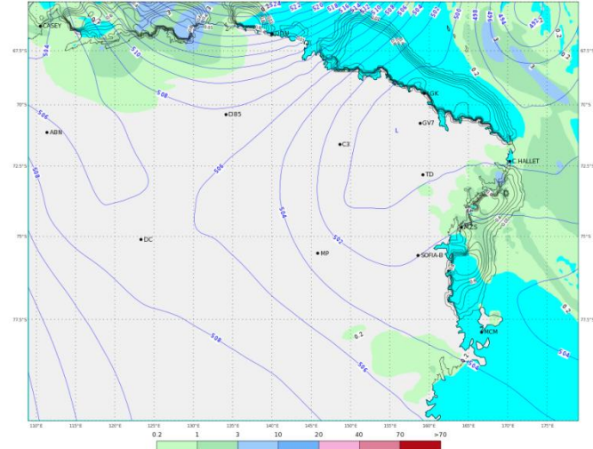
ECMWF 05 Febbraio 2018 00UTC Forecast T+18 VT: Lunedì 05 Febbraio 2018 18UTC Terra Vittoria - Geopotential at 500 hPa + 6h accumulated precipitation (mm)
