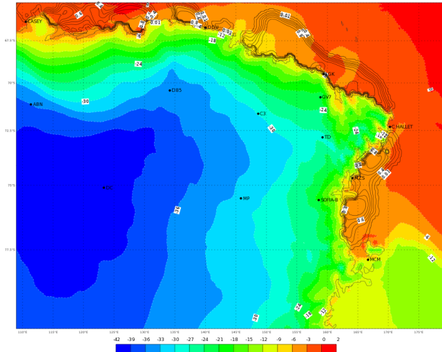
ECMWF 05 Febbraio 2018 00UTC Forecast T+24 VT: Martedì 06 Febbraio 2018 00UTC Terra Vittoria - Temperature at 2 m (°C)
