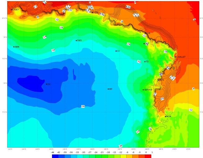
ECMWF 05 Febbraio 2018 00UTC Forecast T+48 VT: Mercoledì 07 Febbraio 2018 00UTC Terra Vittoria - Temperature at 2 m (°C)
