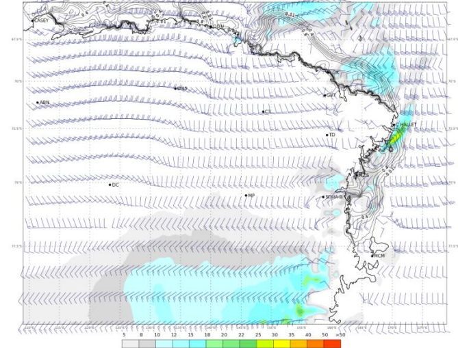
ECMWF 05 Febbraio 2018 00UTC Forecast T+30 VT: Martedì 06 Febbraio 2018 06UTC Terra Vittoria - Wind at 10 m (kts)
