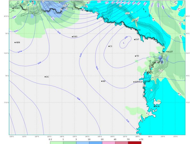
ECMWF 05 Febbraio 2018 00UTC Forecast T+24 VT: Martedì 06 Febbraio 2018 00UTC Terra Vittoria - Geopotential at 500 hPa + 6h accumulated precipitation (mm)
