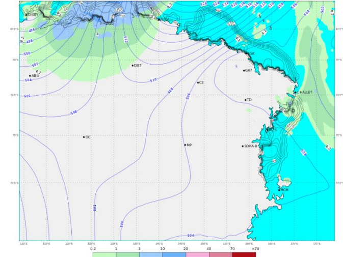
ECMWF 05 Febbraio 2018 00UTC Forecast T+36 VT: Martedì 06 Febbraio 2018 12UTC Terra Vittoria - Geopotential at 500 hPa + 6h accumulated precipitation (mm)
