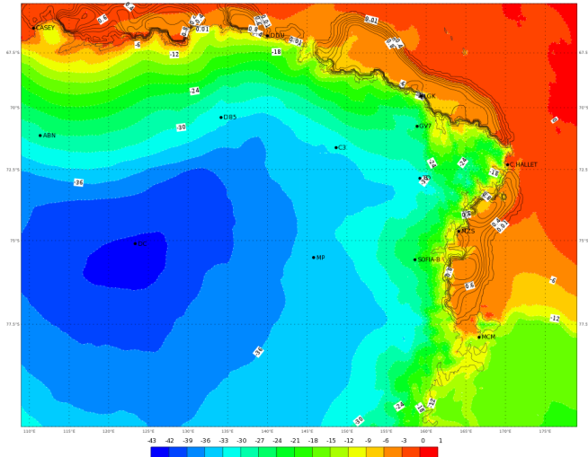
ECMWF 05 Febbraio 2018 00UTC Forecast T+36 VT: Martedì 06 Febbraio 2018 12UTC Terra Vittoria - Temperature at 2 m (°C)
