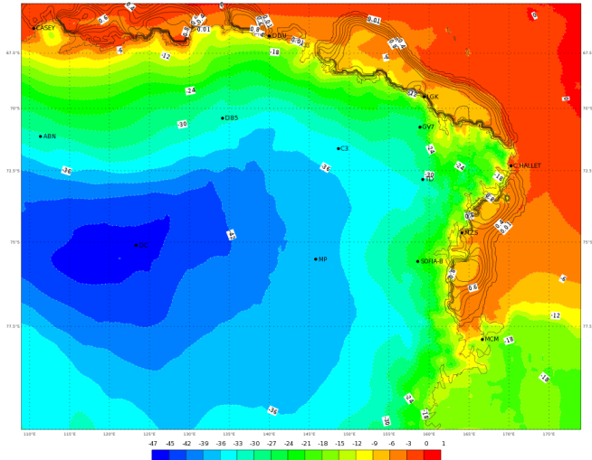
ECMWF 05 Febbraio 2018 00UTC Forecast T+42 VT: Martedì 06 Febbraio 2018 18UTC Terra Vittoria - Temperature at 2 m (°C)
