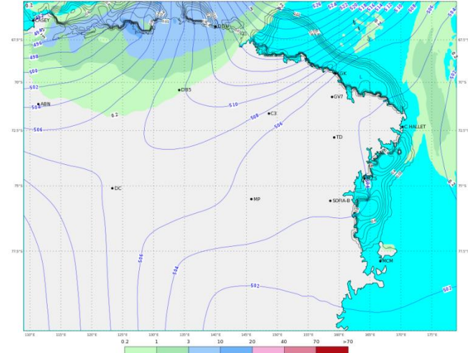
ECMWF 05 Febbraio 2018 00UTC Forecast T+42 VT: Martedì 06 Febbraio 2018 18UTC Terra Vittoria - Geopotential at 500 hPa + 6h accumulated precipitation (mm)
