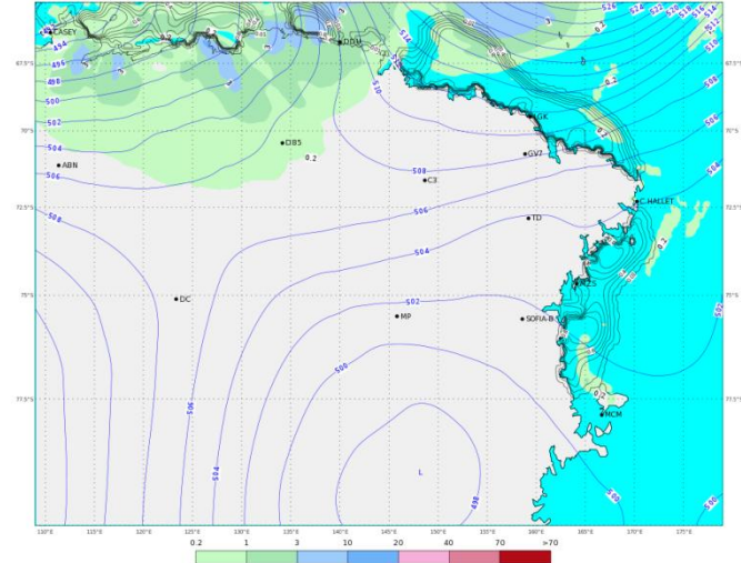
ECMWF 05 Febbraio 2018 00UTC Forecast T+54 VT: Mercoledì 07 Febbraio 2018 06UTC Terra Vittoria - Geopotential at 500 hPa + 6h accumulated precipitation (mm)
