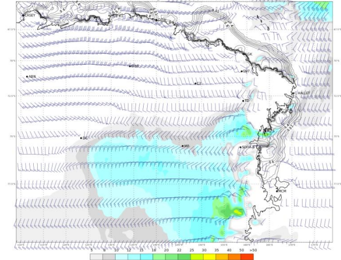
ECMWF 05 Febbraio 2018 00UTC Forecast T+48 VT: Mercoledì 07 Febbraio 2018 00UTC Terra Vittoria - Wind at 10 m (kts)
