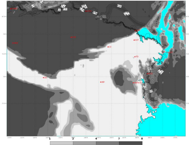
ECMWF 05 Febbraio 2018 00UTC Forecast T+48 VT: Mercoledì 07 Febbraio 2018 00UTC Terra Vittoria - Total cloud cover (oct)
