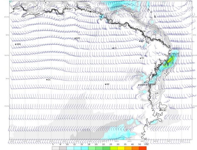
ECMWF 05 Febbraio 2018 00UTC Forecast T+18 VT: Lunedì 05 Febbraio 2018 18UTC Terra Vittoria - Wind at 10 m (kts)
