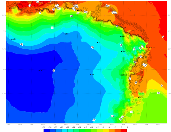
ECMWF 05 Febbraio 2018 00UTC Forecast T+30 VT: Martedì 06 Febbraio 2018 06UTC Terra Vittoria - Temperature at 2 m (°C)
