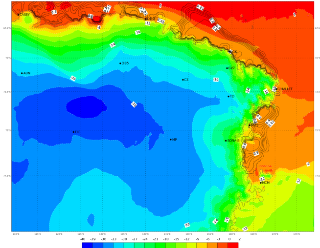
ECMWF 08 Febbraio 2018 00UTC Forecast T+30 VT: Venerdì 09 Febbraio 2018 06UTC Terra Vittoria - Temperature at 2 m (°C)
