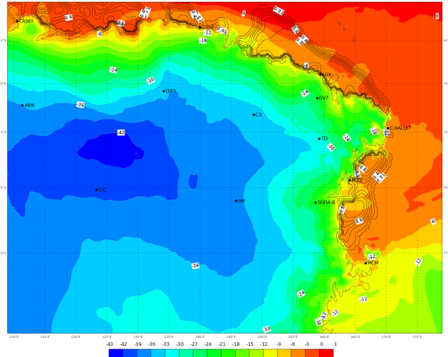
ECMWF 08 Febbraio 2018 00UTC Forecast T+24 VT: Venerdì 09 Febbraio 2018 00UTC Terra Vittoria - Temperature at 2 m (°C)
