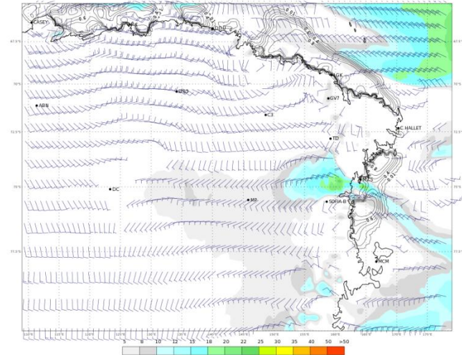
ECMWF 08 Febbraio 2018 00UTC Forecast T+54 VT: Sabato 10 Febbraio 2018 06UTC Terra Vittoria - Wind at 10 m (kts)
