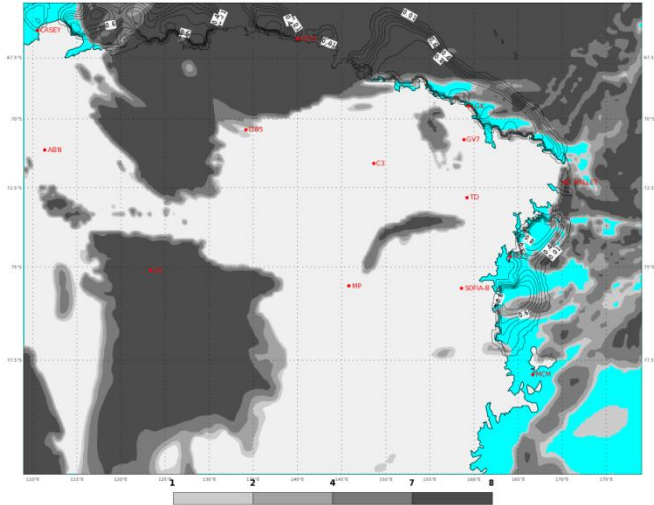
ECMWF 08 Febbraio 2018 00UTC Forecast T+30 VT: Venerdì 09 Febbraio 2018 06UTC Terra Vittoria - Total cloud cover (oct)
