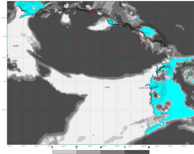
ECMWF 08 Febbraio 2018 00UTC Forecast T+54 VT: Sabato 10 Febbraio 2018 06UTC Terra Vittoria - Total cloud cover (oct)
