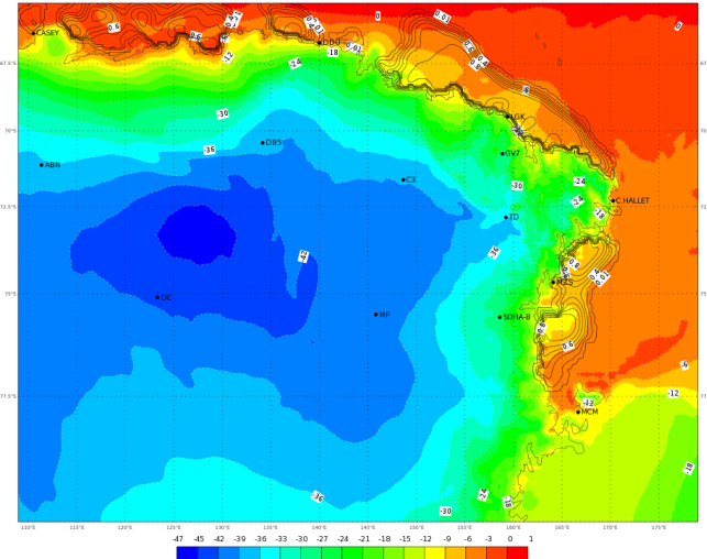
ECMWF 08 Febbraio 2018 00UTC Forecast T+18 VT: Giovedì 08 Febbraio 2018 18UTC Terra Vittoria - Temperature at 2 m (°C)
