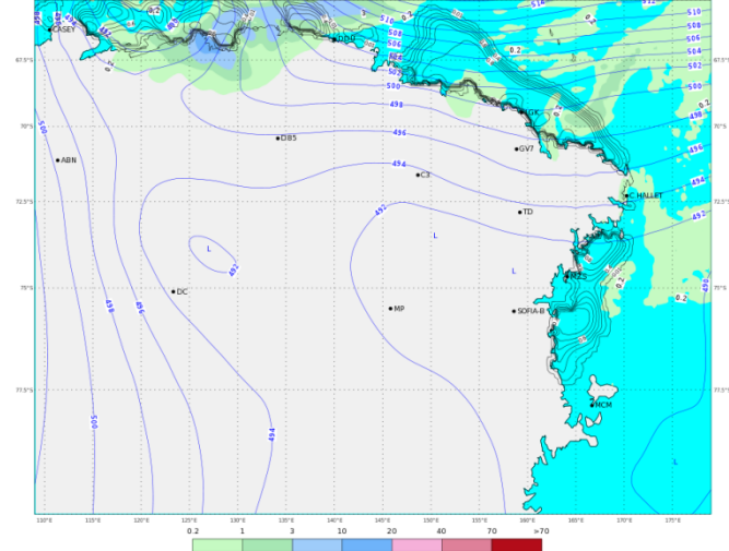
ECMWF 08 Febbraio 2018 00UTC Forecast T+18 VT: Giovedì 08 Febbraio 2018 18UTC Terra Vittoria - Geopotential at 500 hPa + 6h accumulated precipitation (mm)
