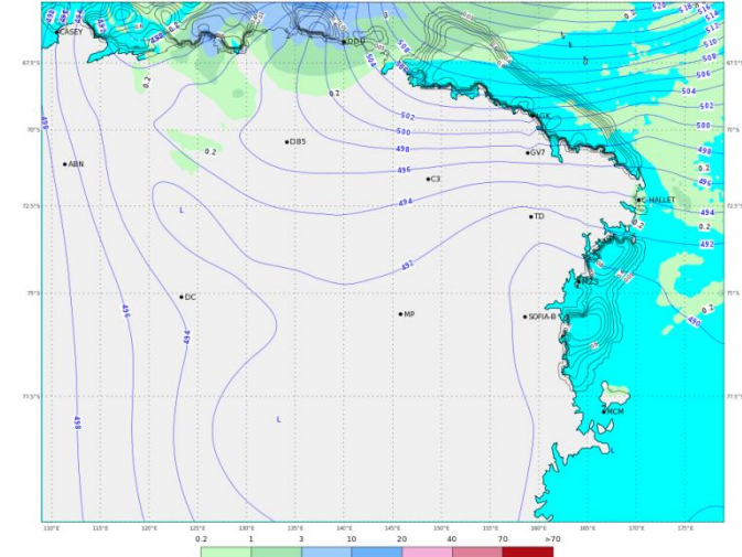
ECMWF 08 Febbraio 2018 00UTC Forecast T+30 VT: Venerdì 09 Febbraio 2018 06UTC Terra Vittoria - Geopotential at 500 hPa + 6h accumulated precipitation (mm)
