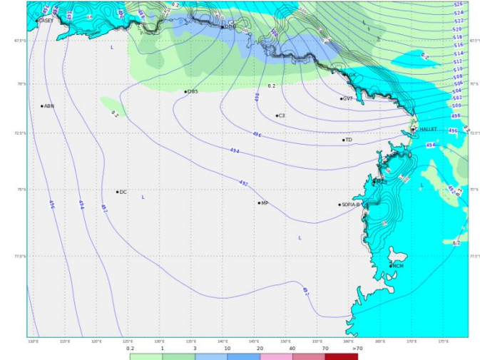
ECMWF 08 Febbraio 2018 00UTC Forecast T+42 VT: Venerdì 09 Febbraio 2018 18UTC Terra Vittoria - Geopotential at 500 hPa + 6h accumulated precipitation (mm)
