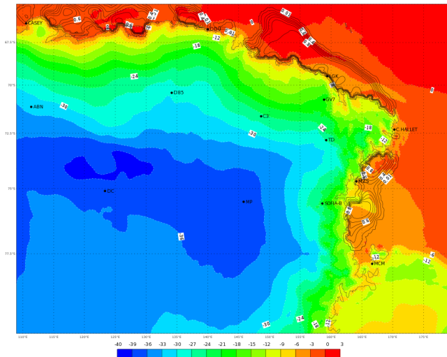
ECMWF 08 Febbraio 2018 00UTC Forecast T+54 VT: Sabato 10 Febbraio 2018 06UTC Terra Vittoria - Temperature at 2 m (°C)
