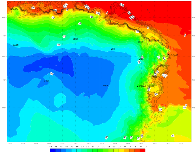
ECMWF 08 Febbraio 2018 00UTC Forecast T+42 VT: Venerdì 09 Febbraio 2018 18UTC Terra Vittoria - Temperature at 2 m (°C)
