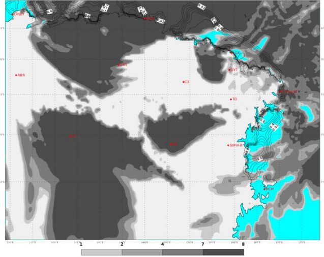
ECMWF 08 Febbraio 2018 00UTC Forecast T+24 VT: Venerdì 09 Febbraio 2018 00UTC Terra Vittoria - Total cloud cover (oct)
