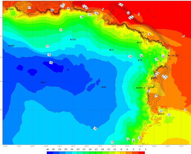
ECMWF 08 Febbraio 2018 00UTC Forecast T+48 VT: Sabato 10 Febbraio 2018 00UTC Terra Vittoria - Temperature at 2 m (°C)
