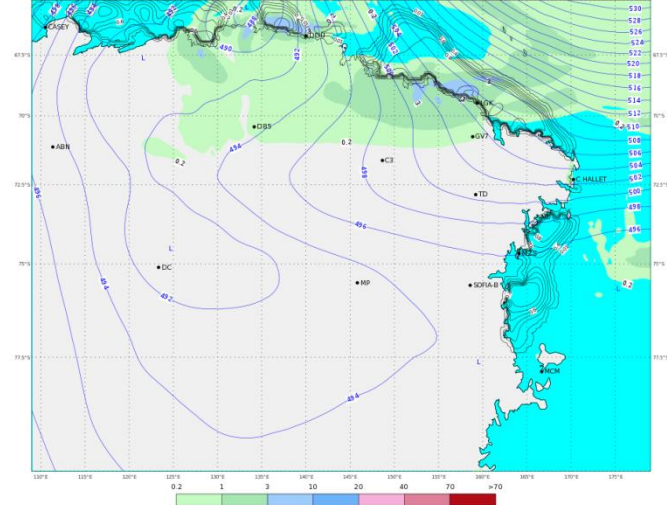
ECMWF 08 Febbraio 2018 00UTC Forecast T+48 VT: Sabato 10 Febbraio 2018 00UTC Terra Vittoria - Geopotential at 500 hPa + 6h accumulated precipitation (mm)
