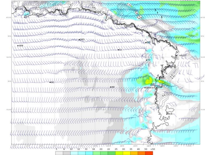
ECMWF 08 Febbraio 2018 00UTC Forecast T+42 VT: Venerdì 09 Febbraio 2018 18UTC Terra Vittoria - Wind at 10 m (kts)
