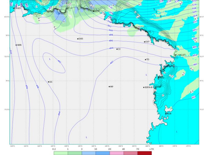
ECMWF 08 Febbraio 2018 00UTC Forecast T+24 VT: Venerdì 09 Febbraio 2018 00UTC Terra Vittoria - Geopotential at 500 hPa + 6h accumulated precipitation (mm)
