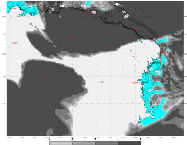
ECMWF 08 Febbraio 2018 00UTC Forecast T+42 VT: Venerdì 09 Febbraio 2018 18UTC Terra Vittoria - Total cloud cover (oct)
