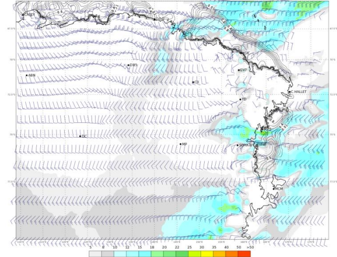
ECMWF 08 Febbraio 2018 00UTC Forecast T+18 VT: Giovedì 08 Febbraio 2018 18UTC Terra Vittoria - Wind at 10 m (kts)
