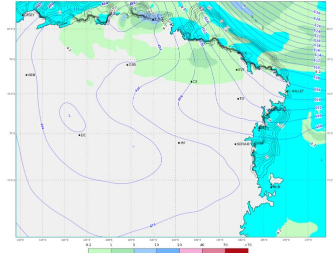
ECMWF 08 Febbraio 2018 00UTC Forecast T+54 VT: Sabato 10 Febbraio 2018 06UTC Terra Vittoria - Geopotential at 500 hPa + 6h accumulated precipitation (mm)
