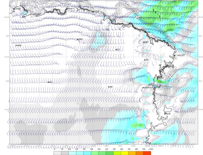
ECMWF 08 Febbraio 2018 00UTC Forecast T+24 VT: Venerdì 09 Febbraio 2018 00UTC Terra Vittoria - Wind at 10 m (kts)
