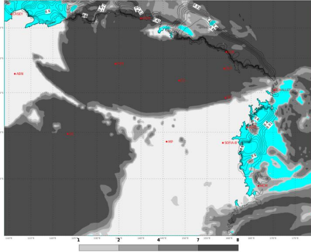
ECMWF 08 Febbraio 2018 00UTC Forecast T+48 VT: Sabato 10 Febbraio 2018 00UTC Terra Vittoria - Total cloud cover (oct)
