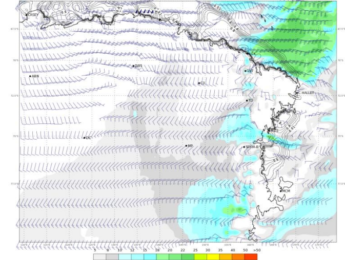
ECMWF 08 Febbraio 2018 00UTC Forecast T+30 VT: Venerdì 09 Febbraio 2018 06UTC Terra Vittoria - Wind at 10 m (kts)
