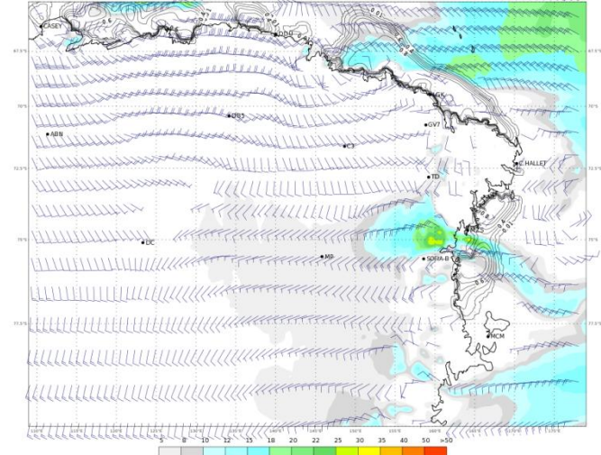
ECMWF 08 Febbraio 2018 00UTC Forecast T+48 VT: Sabato 10 Febbraio 2018 00UTC Terra Vittoria - Wind at 10 m (kts)
