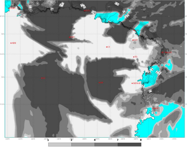
ECMWF 08 Febbraio 2018 00UTC Forecast T+18 VT: Giovedì 08 Febbraio 2018 18UTC Terra Vittoria - Total cloud cover (oct)
